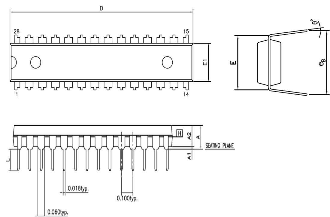
图 25–1. DIP-28
