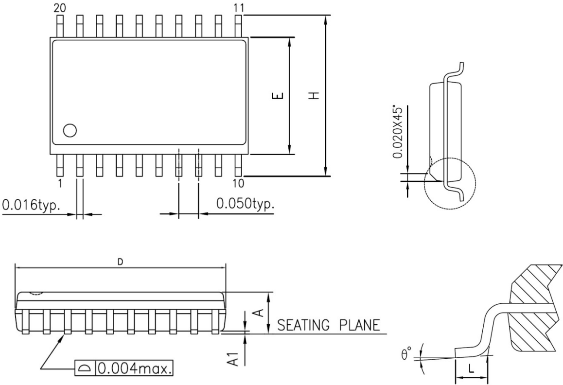
图 25-4. SOP-20
