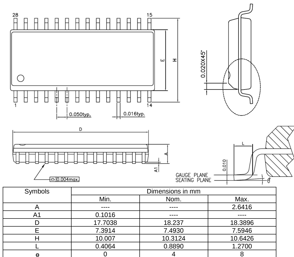
图 25-2. SOP-28
