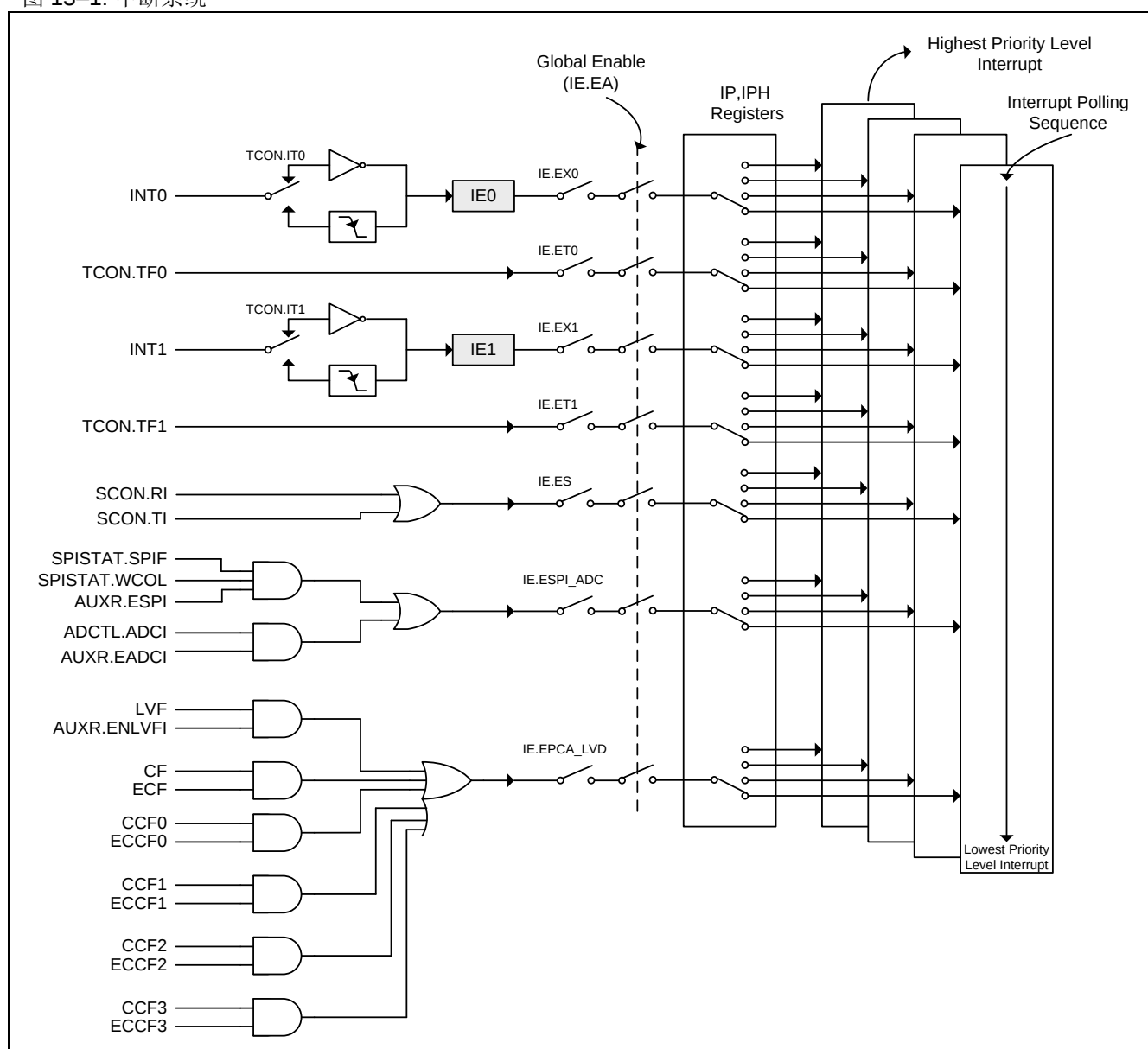
图 13-1. 中断系统
