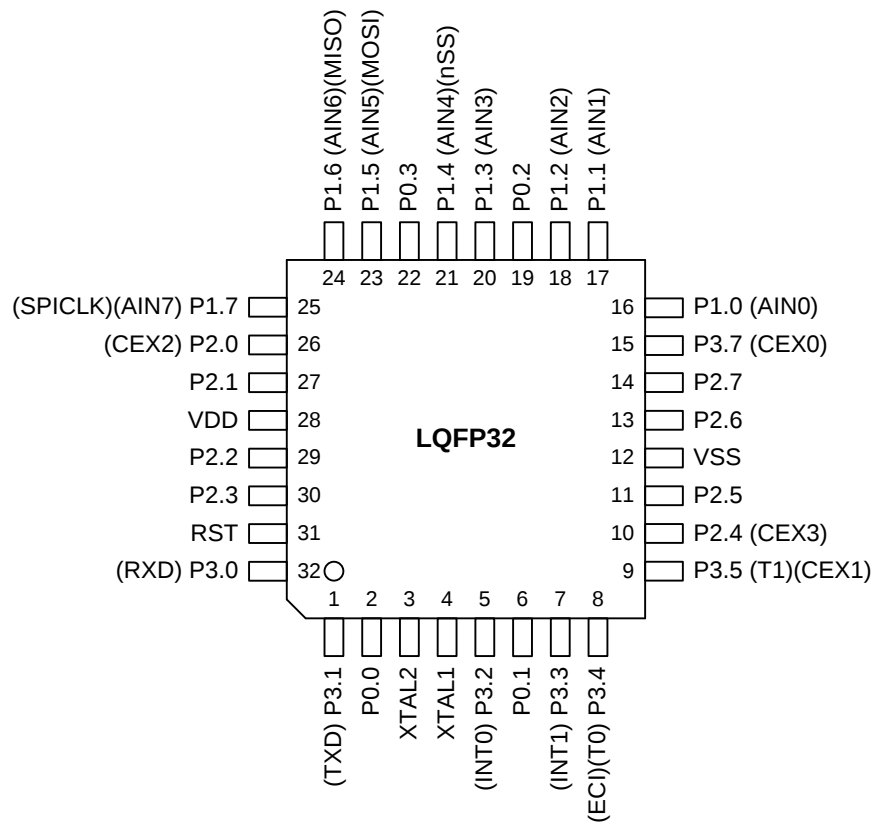
图 4-3. MA803_MA804 32-脚 顶视图
