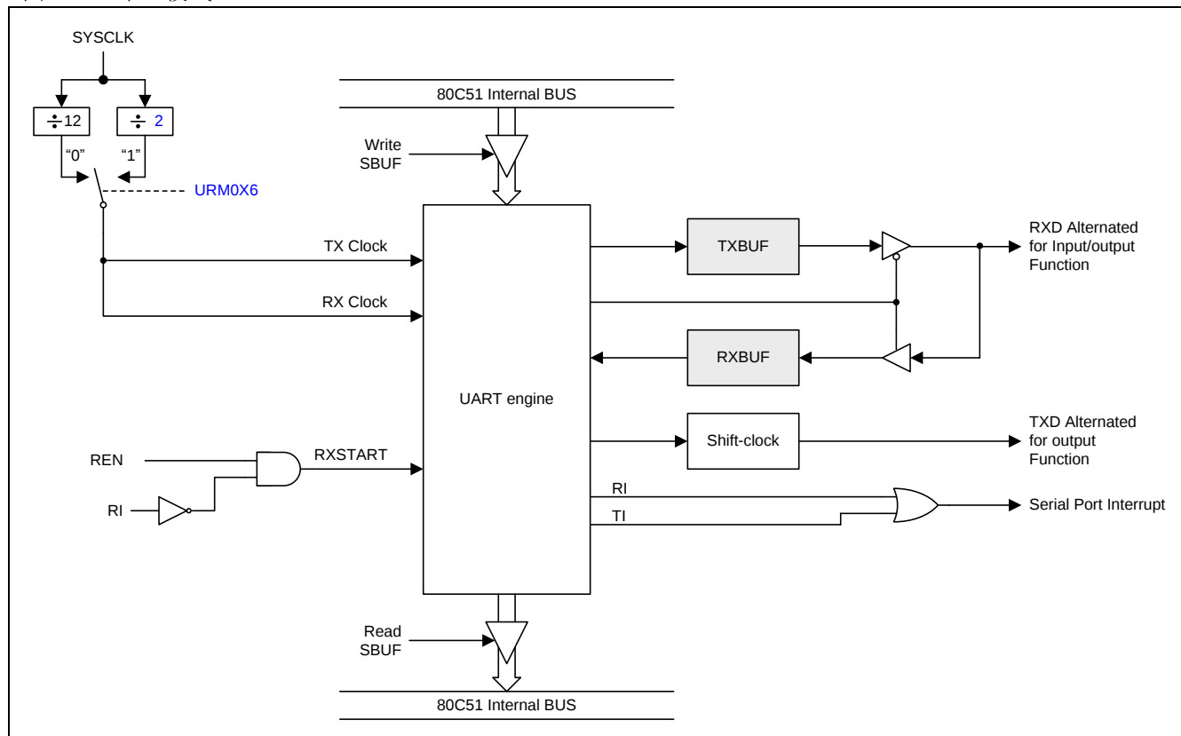
图 15-3. 串口模式 0
