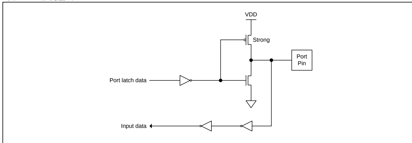
图 12-2. 推挽输出
