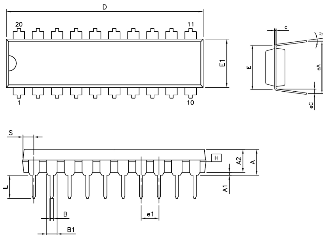
图 25-3. DIP-20
