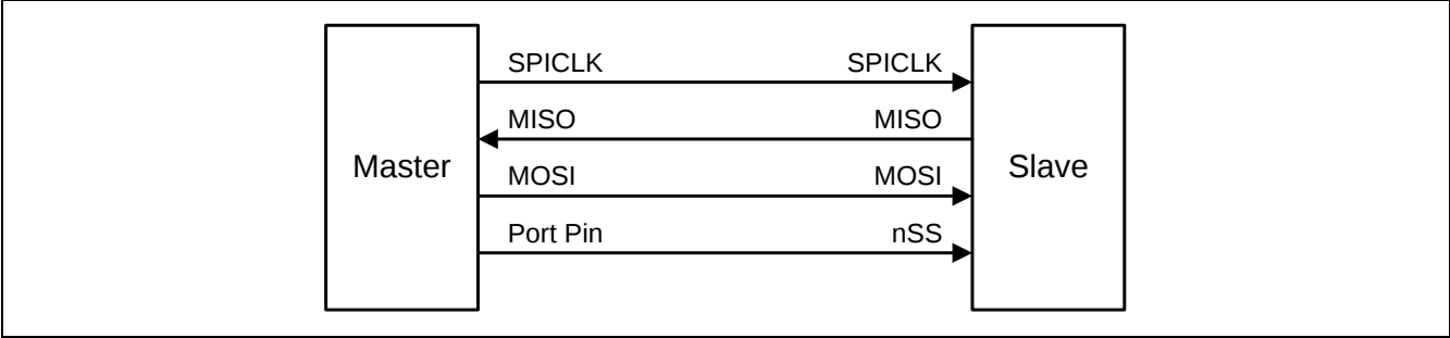
图 17-2. SPI 单主从机配置
