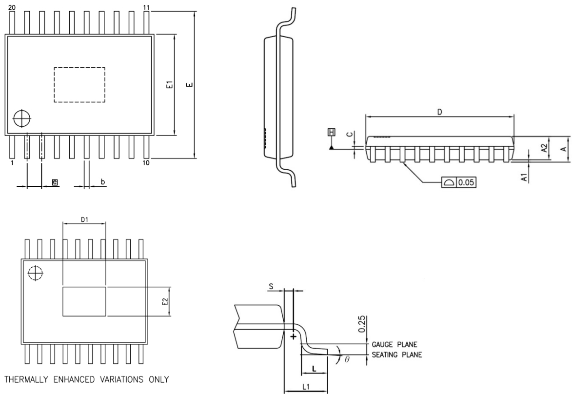
图 25-5. TSSOP-20
