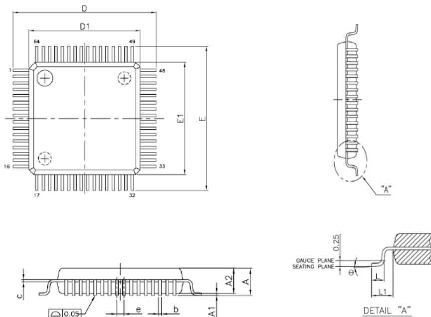
图 6.3: LQFP64 7X7mm, 0.4mm 间距以及封装参数
