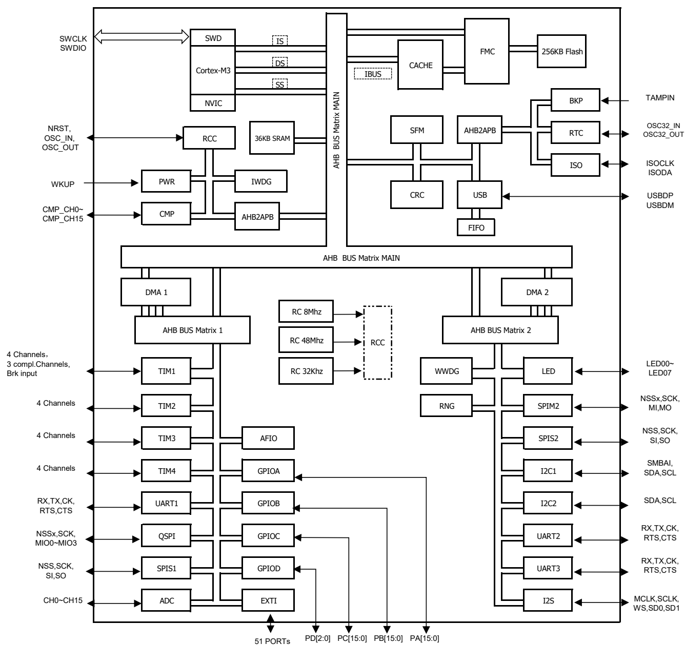
图 3.1: MG32F104xx 系统框图
