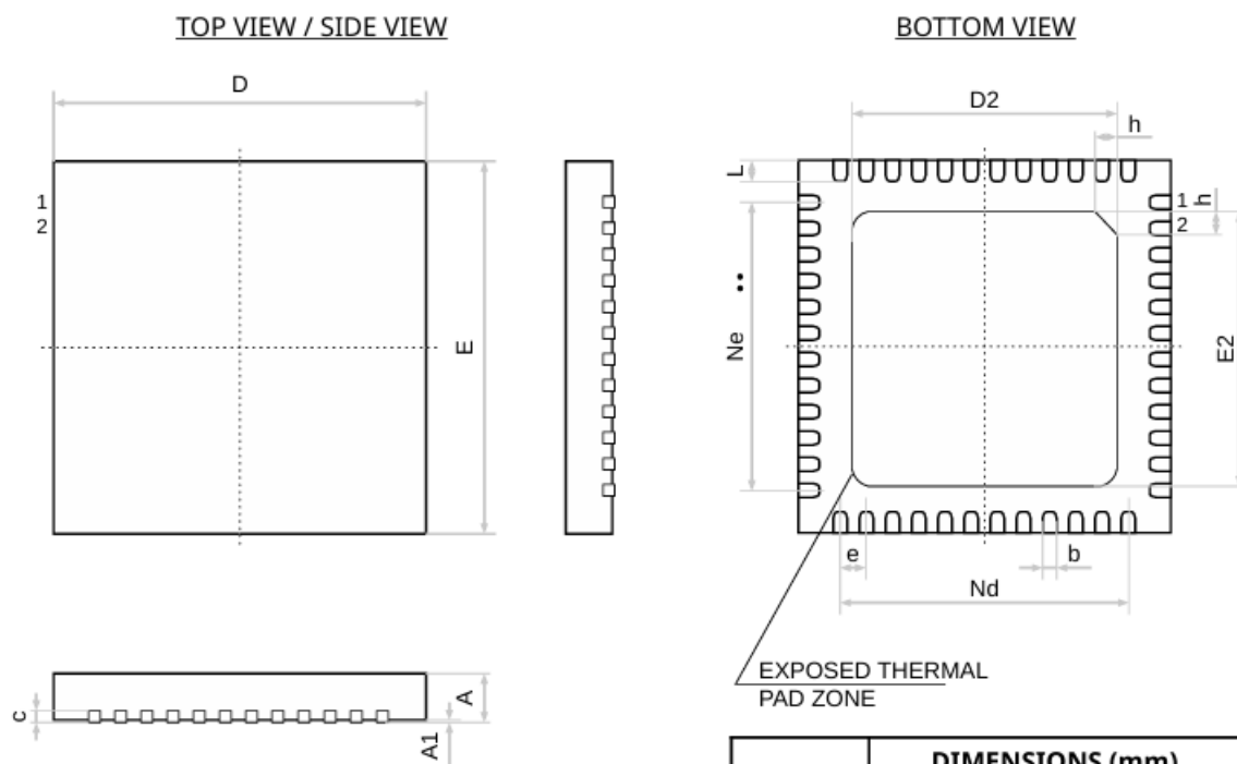
图 6.5: QFN48 6X6mm, 0.4mm 间距以及封装参数
