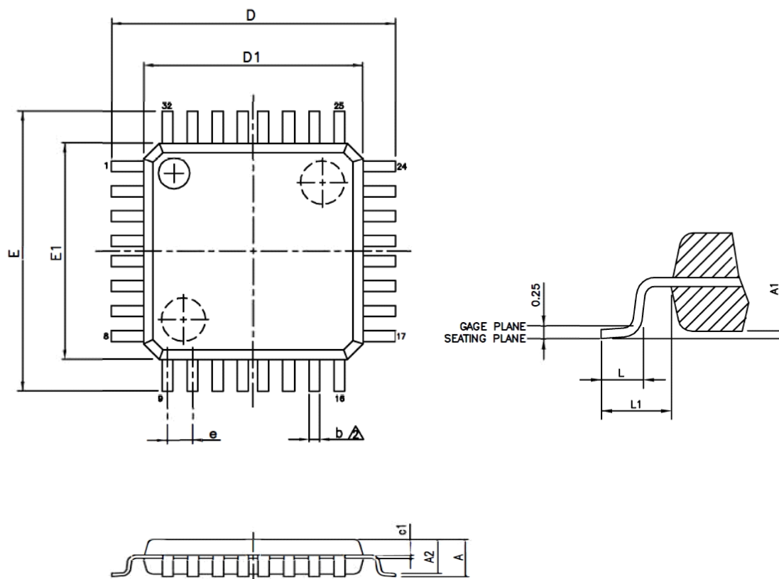
图 9-1. LQFP-32 (7mm X 7mm) ~ AD32
