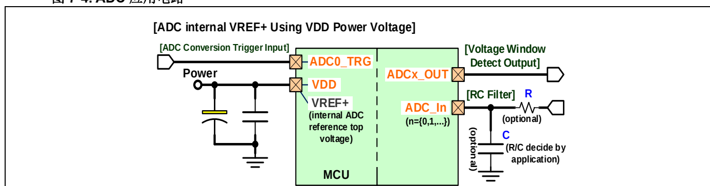
图 7-4. ADC 应用电路
