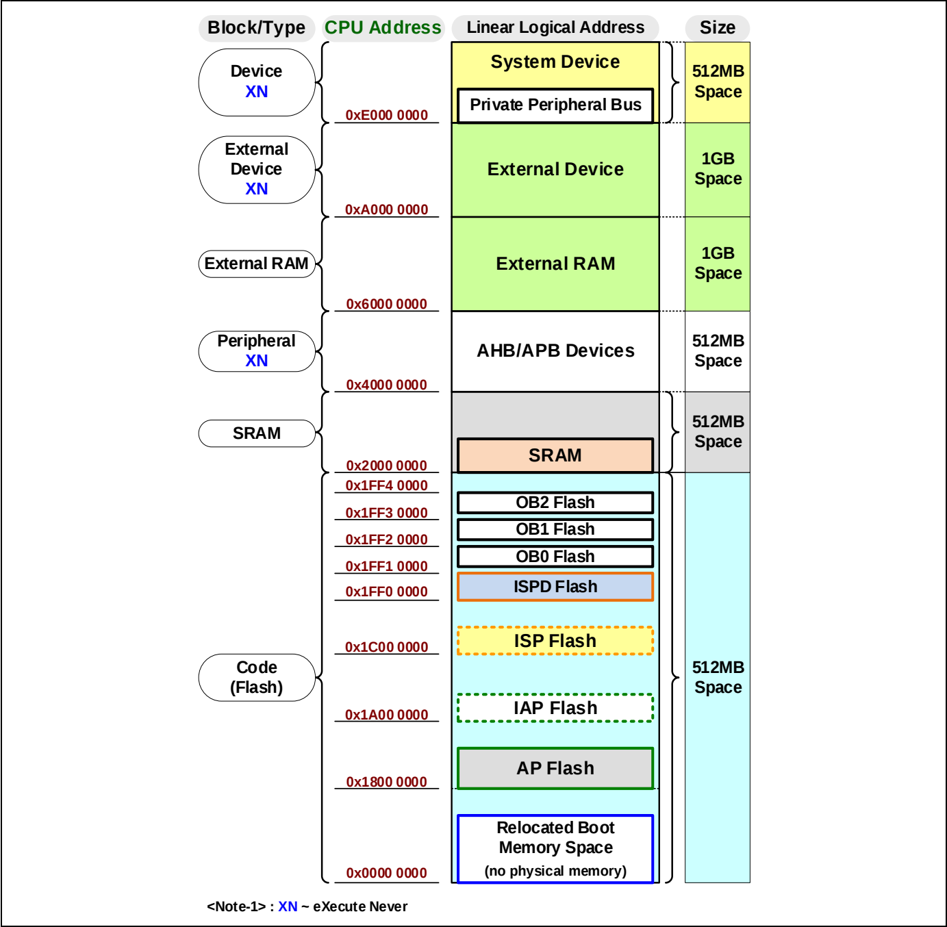
图 5-1. 内存映射
