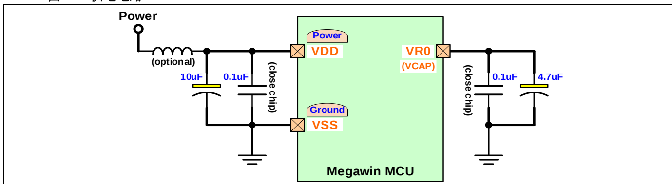
图 7-1. 供电电路
