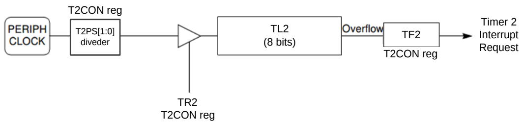
图 13.4.15 定时器 2 模式 3
