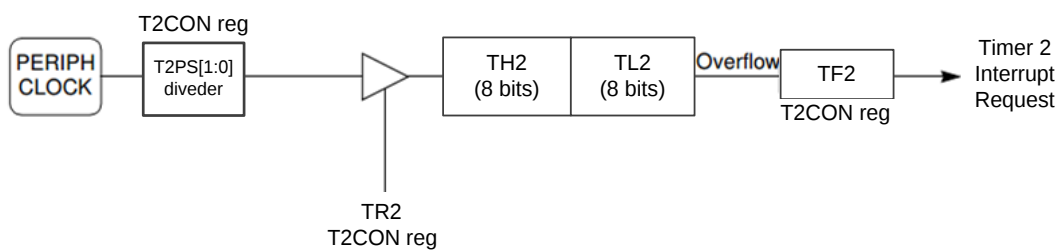
图 13.4.13 定时器 2 模式 1
