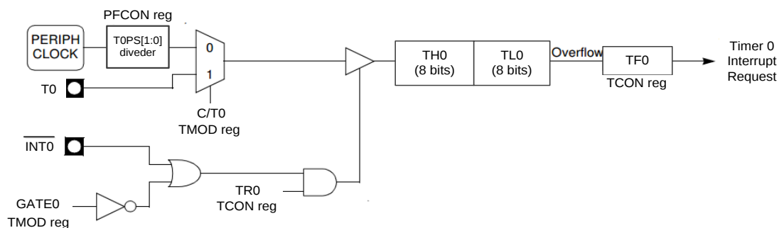
图 13.4.6 定时器 0 模式 1
