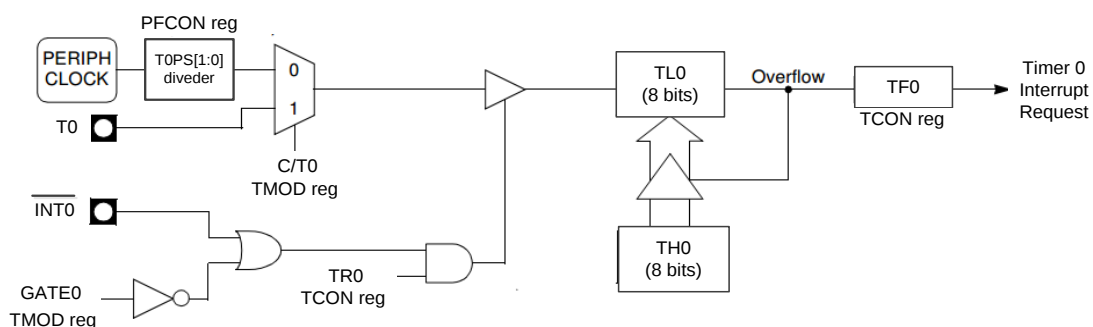
图 13.4.7 定时器0 模式 2
