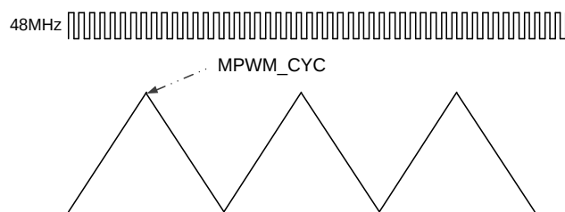
图 19.6.7 : 电机 PWM 是向上向下定时器 r
