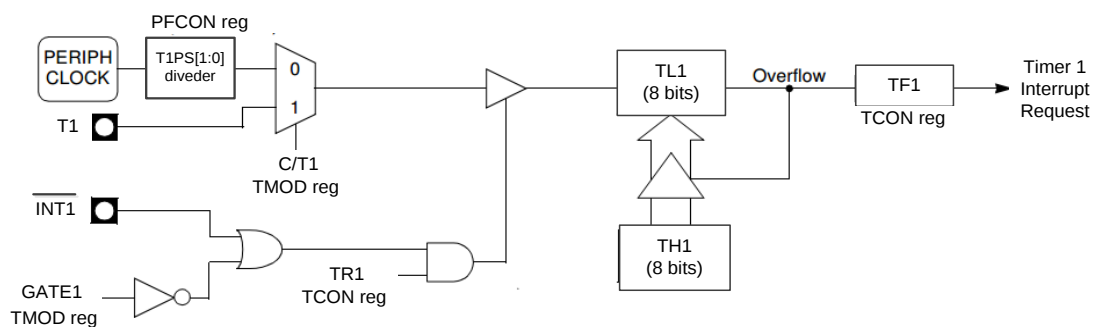
图 13.4.11 定时器 1 模式 2
