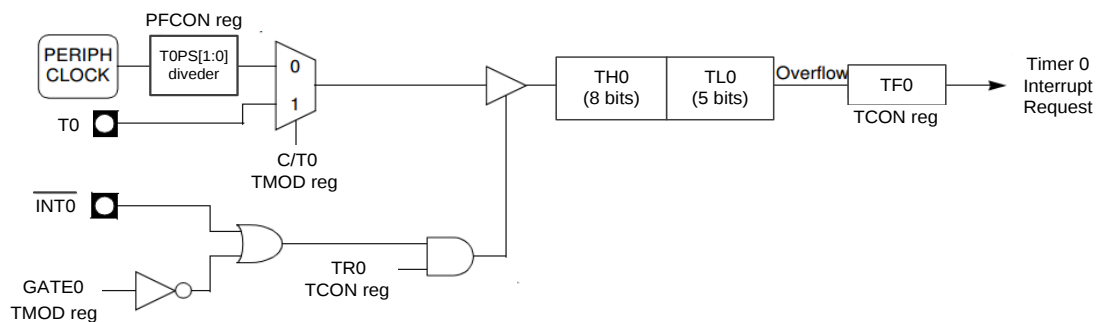
图 13.4.5 定时器 0 模式 0
