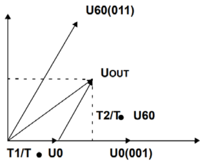
图 25.6.3：平均 SVPWM
