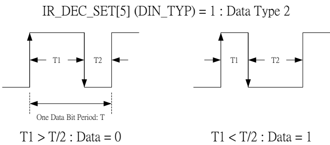
图 23.1.2 : 输入数据类型选择
