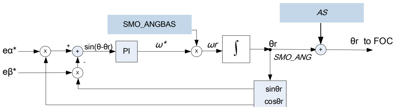
图 25.5.3 : PLL 架构
