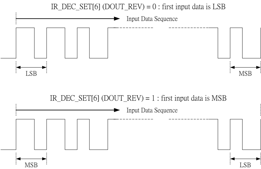
图 23.1.3 : 输出数据反向选择
