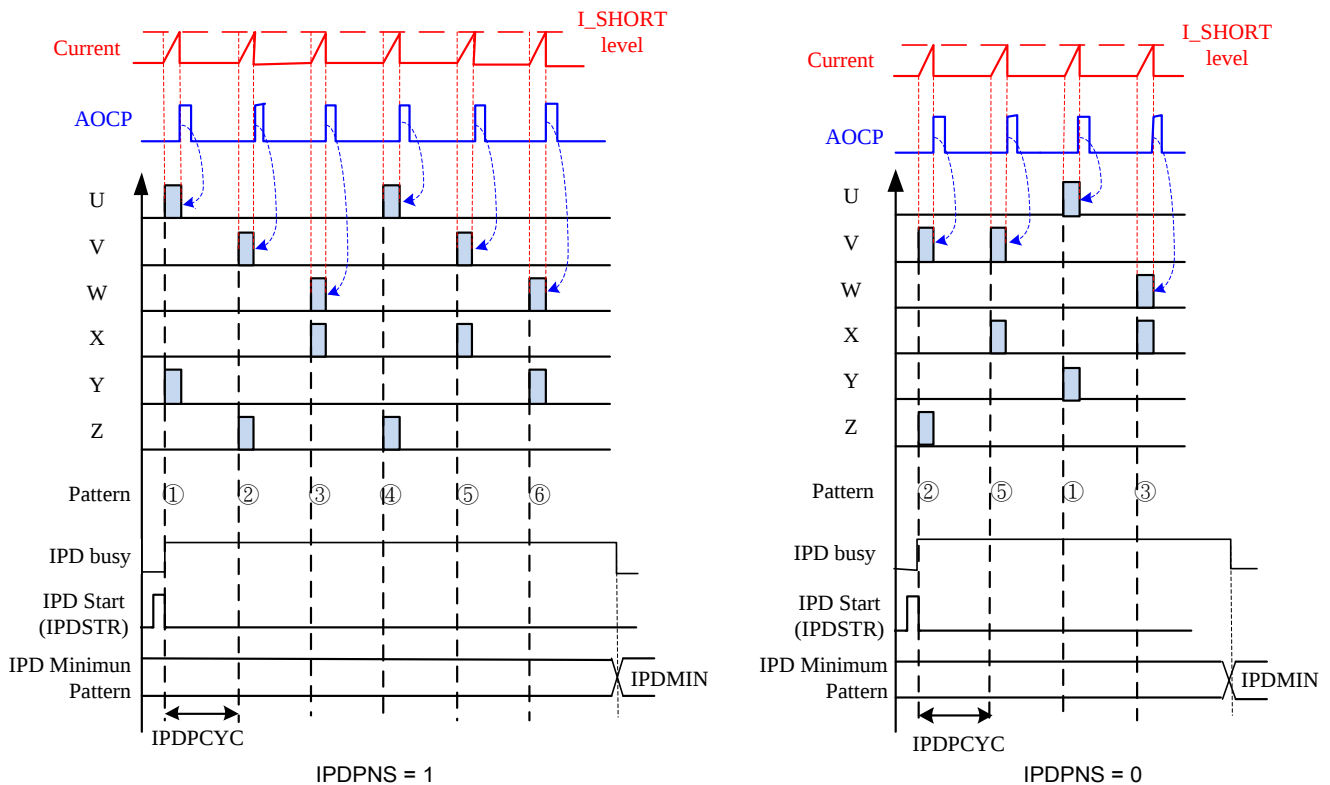
图 25.9.2 : 6-pattern 或 4-pattern 旋转前转子位置检测的 IPD
