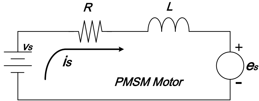
图 25.5.2：电机模型
