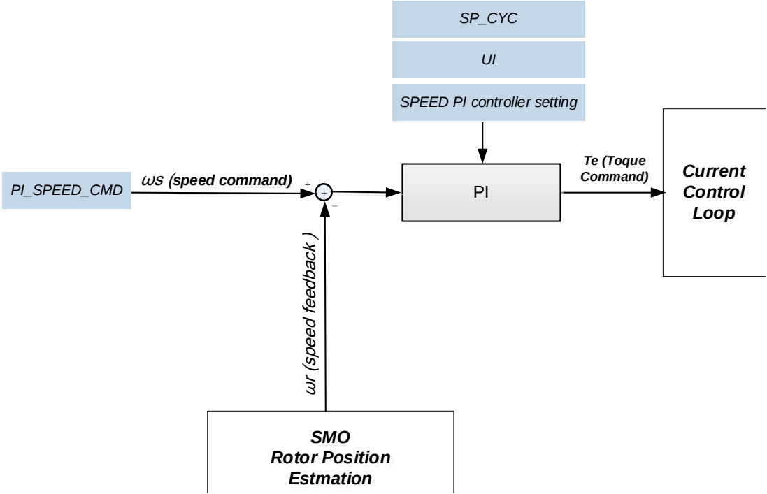
图 25.7.1：速度控制环模块框图
