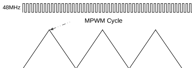
图 25.6.6：电机 PWM 向上向下定时器
