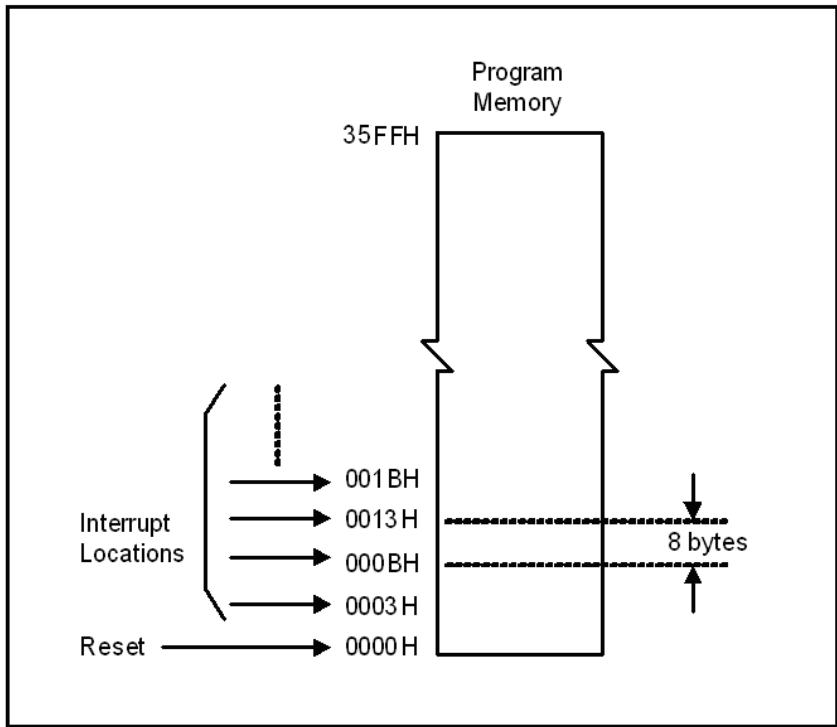
图 8-1 程序存储器
