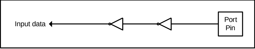
图 10-3 仅输入
