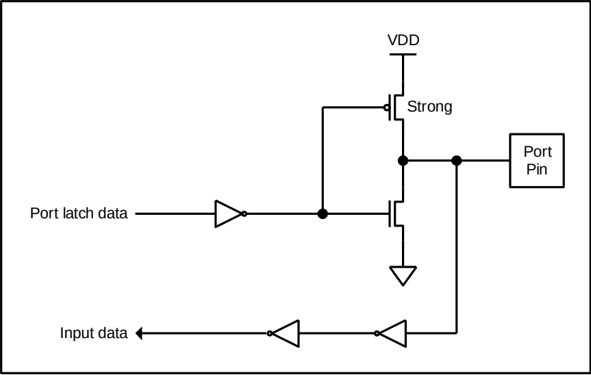
图 10-2 推挽输出
