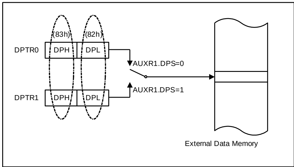
图 9-1 双 DPTR
