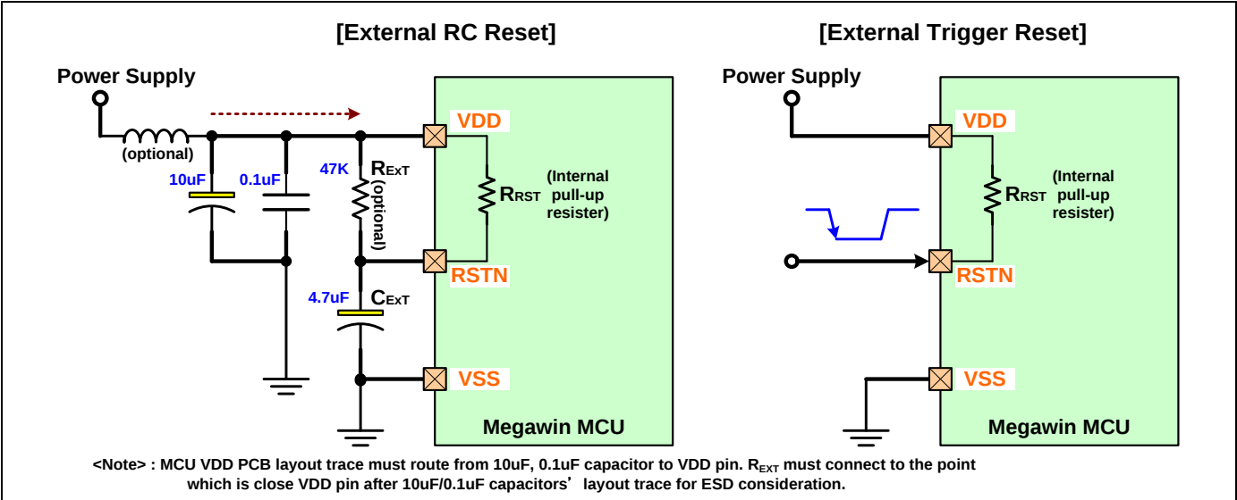
图 7-2. 复位电路
