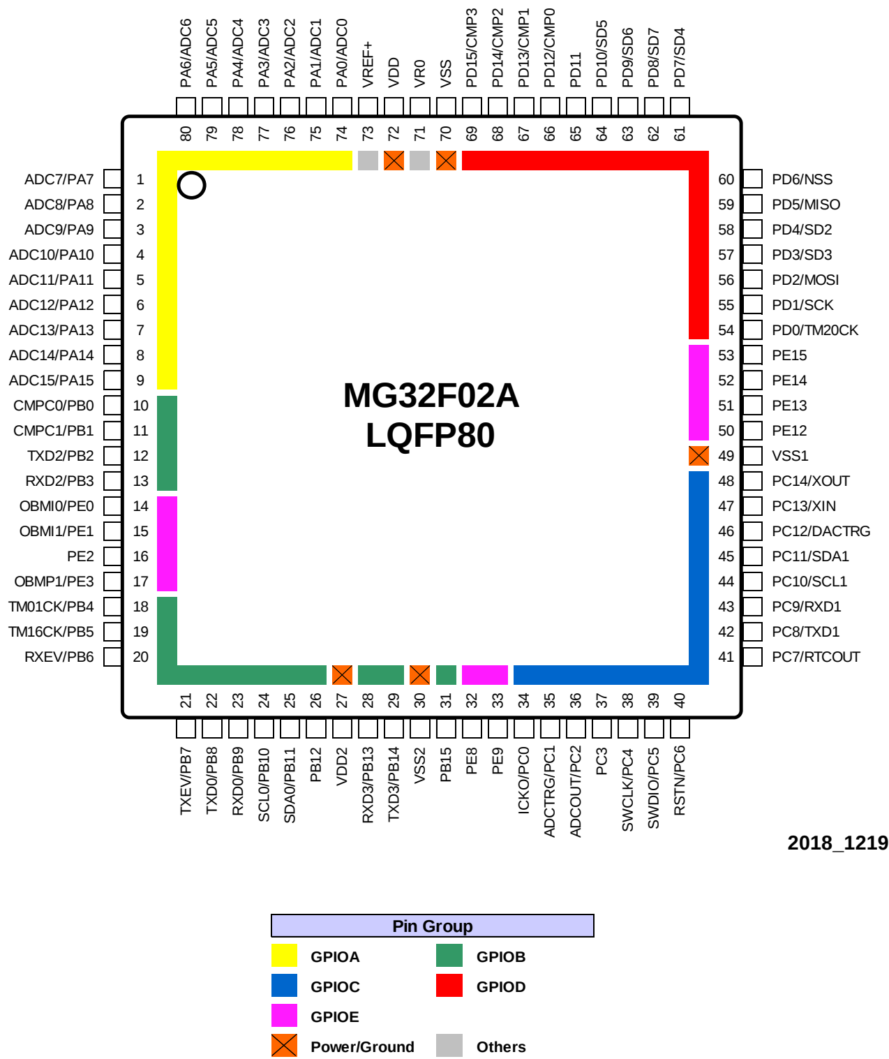
图 4-1. LQFP80 封装引脚
