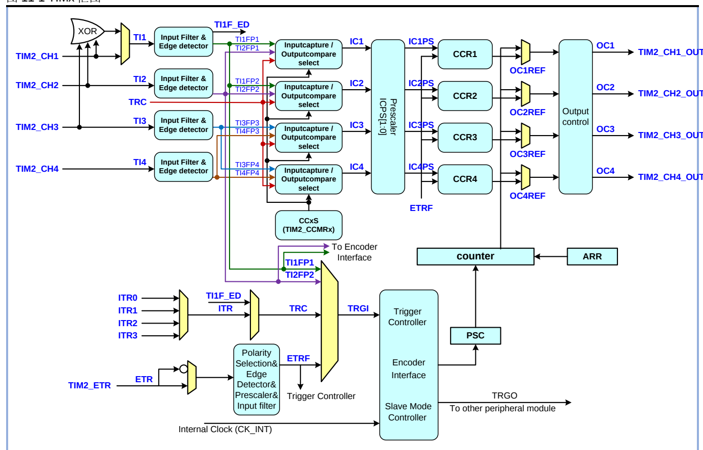
图 11-1 TIMx 框图
