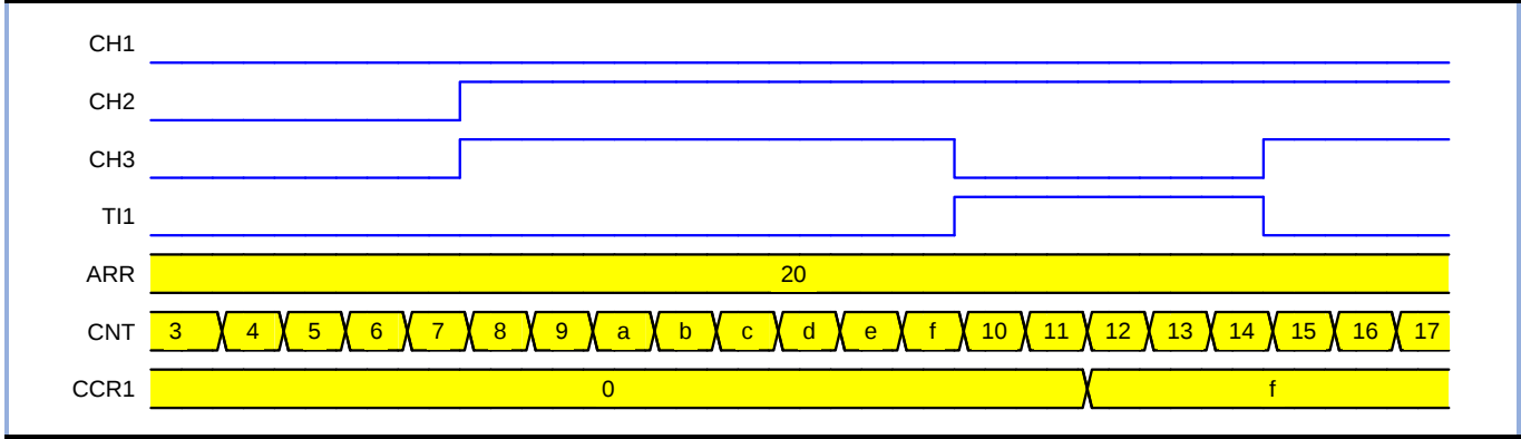
图 11-29（TI1 异或输入）输入捕获波形图
