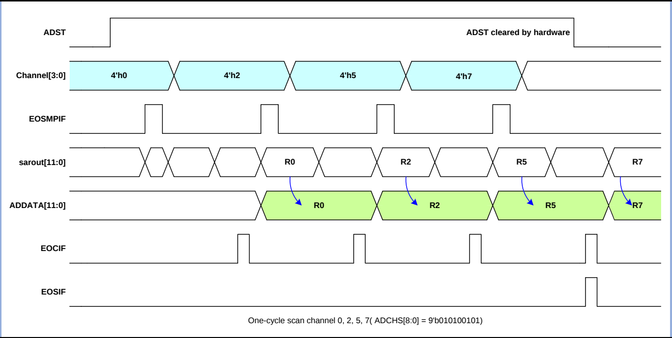
图 16-5 单周期扫描下使能通道转换时序图（通道方向从低到高）
