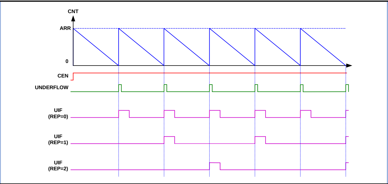
图 10-14 边沿对齐模式递减计数时序图
