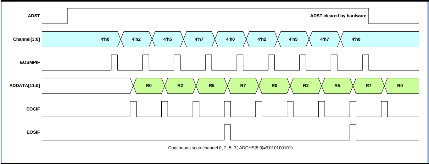
图 16-6 连续扫描模式使能通道转换时序图（通道方向由低到高）
