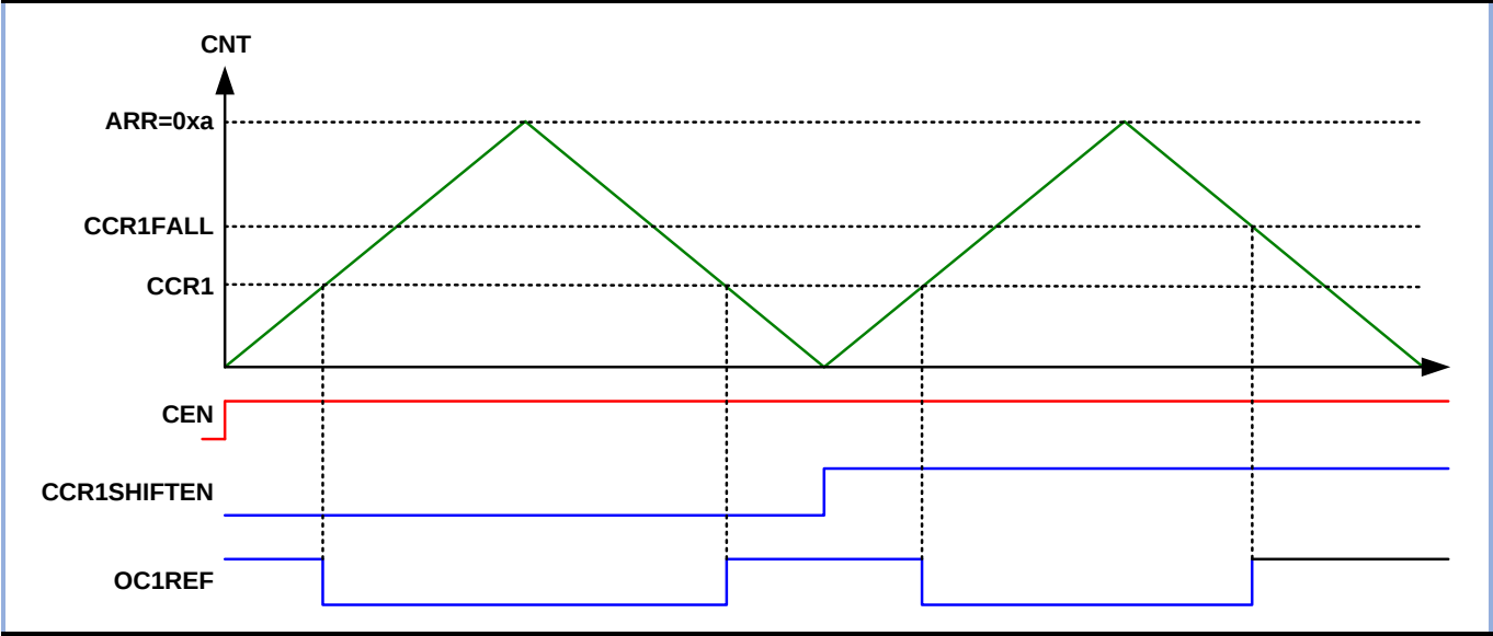
图 10-20 移相功能
