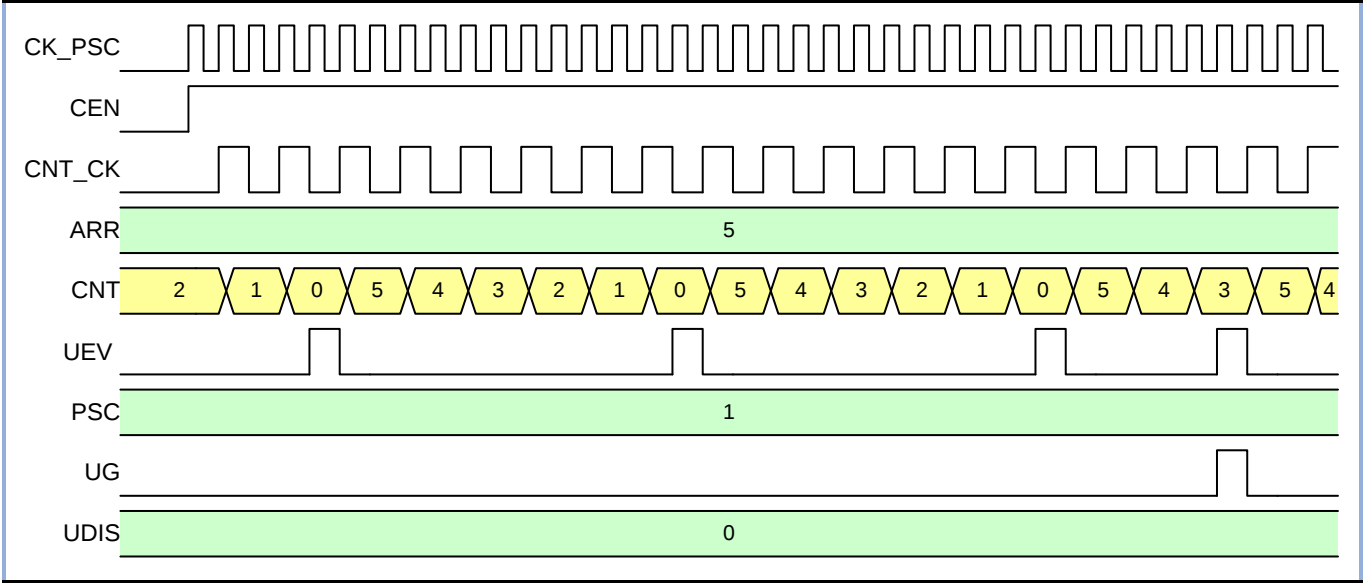
图 11-8 递减计数模式 (UDIS=0)
