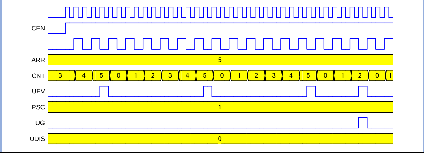
图 12-3 递增计数模式(UDIS=0)
