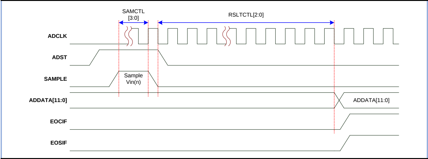
图 16-3 单次转换模式时序图
