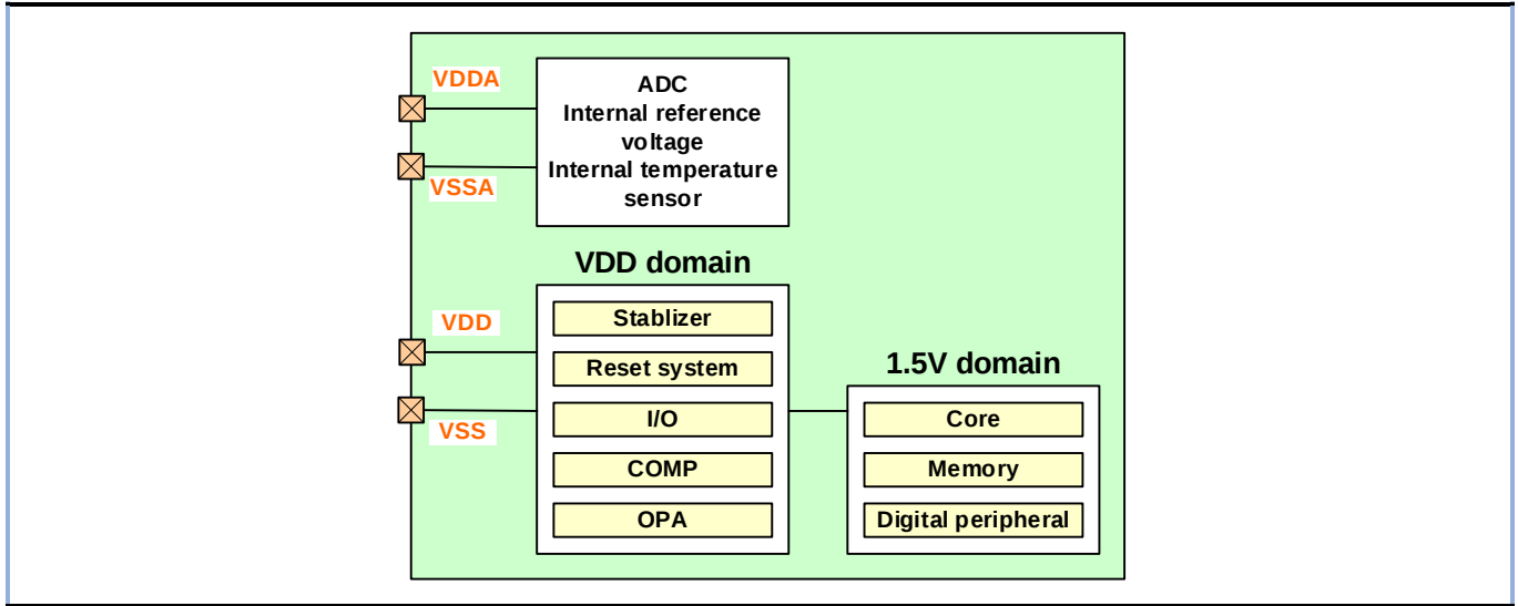
图 3-1 电源控制框图
