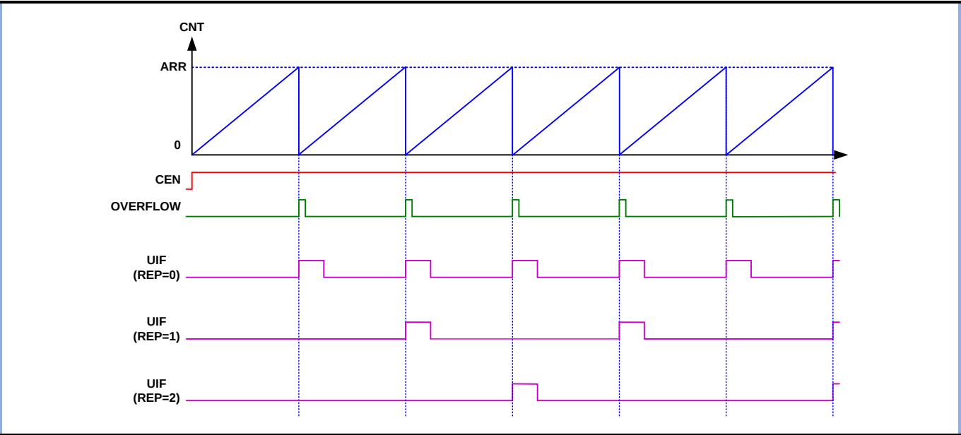
图 10-13 边沿对齐模式递增计数时序图
