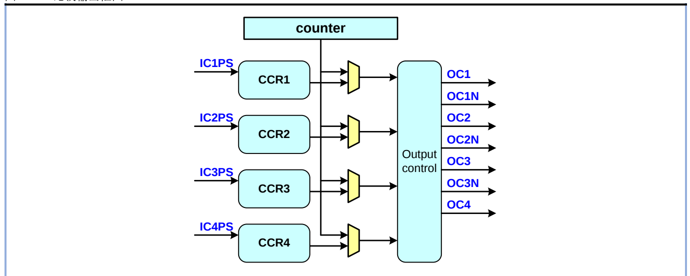
图 11-14 比较输出框图
