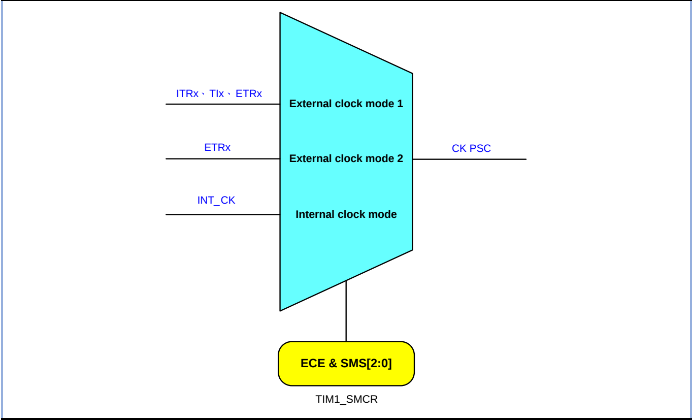
图 10-2 时钟选择
