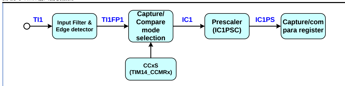
图 13-5 TIMx 输入捕获框图
