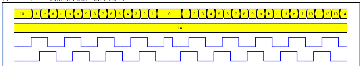
图 11-24 IC1FP1 反相编码器接口模式时序图
