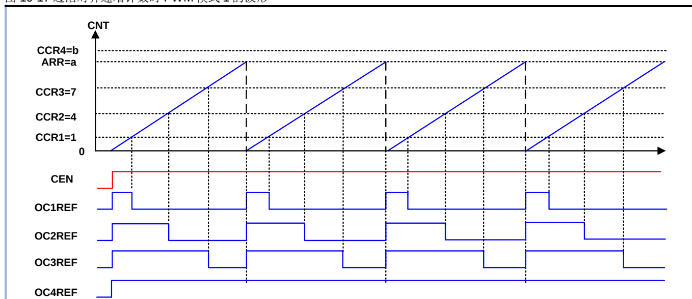
图 10-17 边沿对齐递增计数时 PWM 模式 1 的波形
