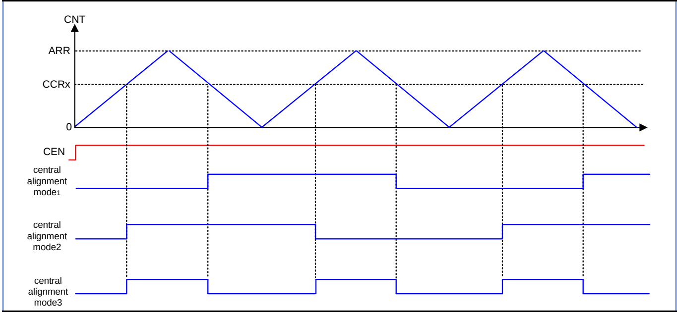
图 10-23 中心对齐模式下 CCx_SETTRGO 输出示例
