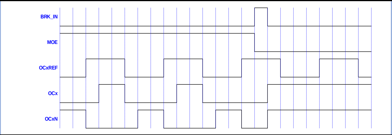
图 10-28 响应刹车输出 (OISx=1, OISxN=1)
