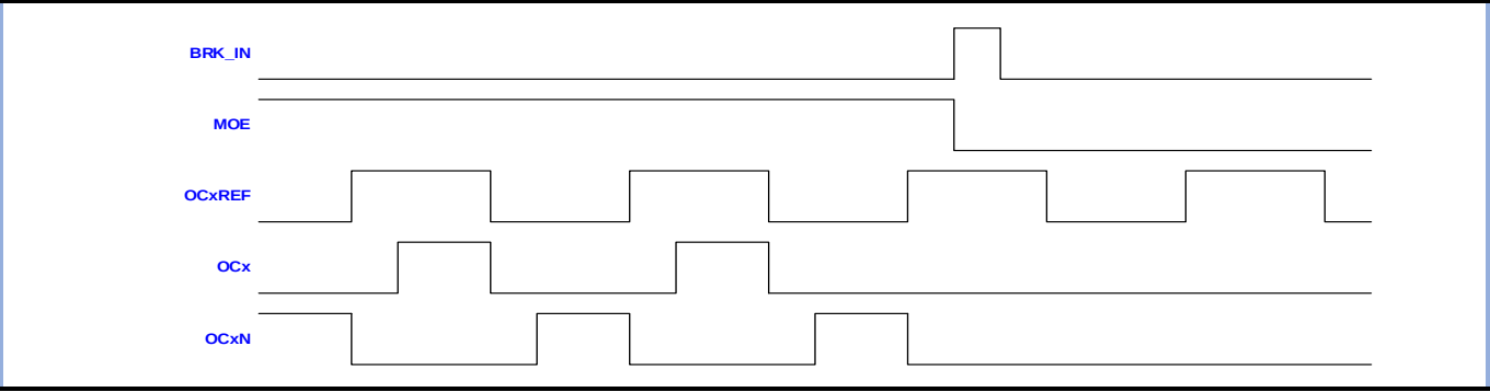
图 10-25 响应刹车输出 (OISx=0 , OISxN=0)
