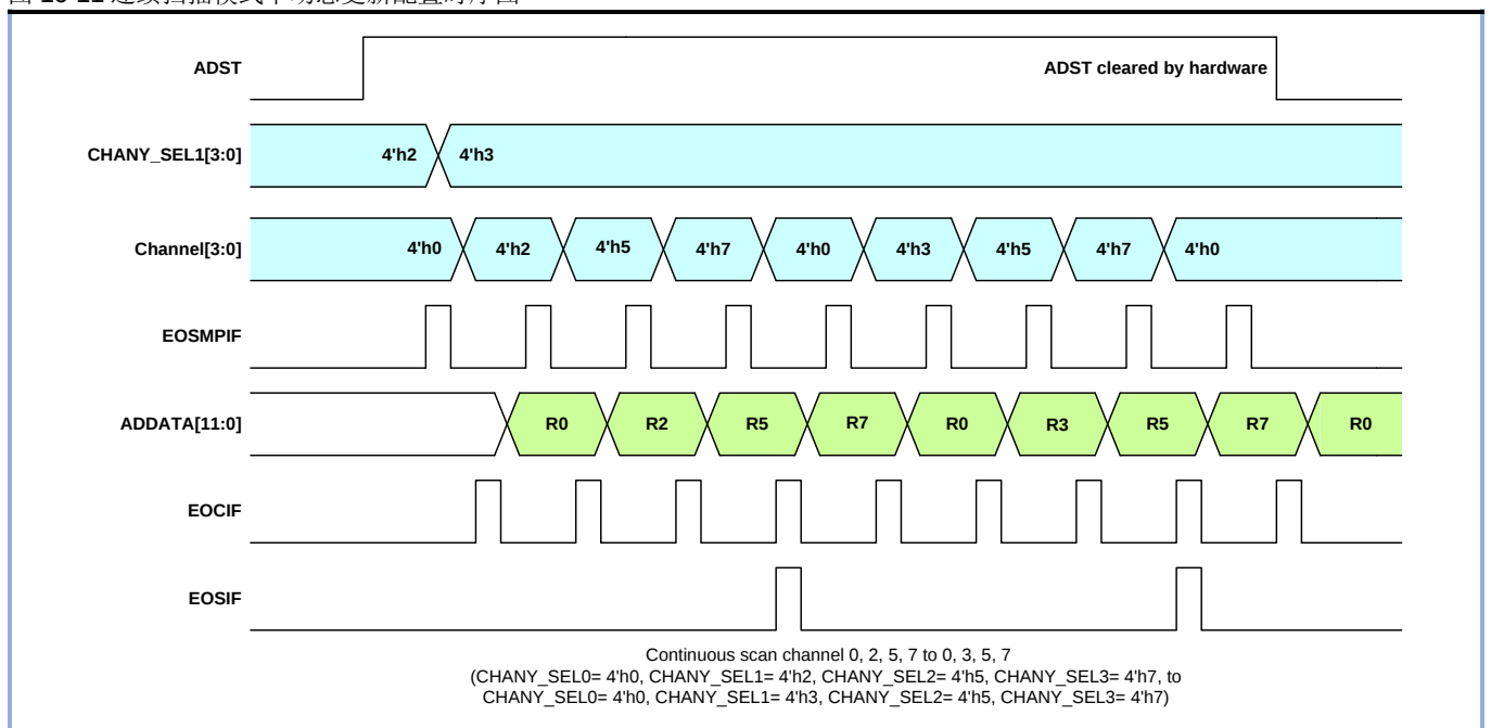
图 16-11 连续扫描模式下动态更新配置时序图
