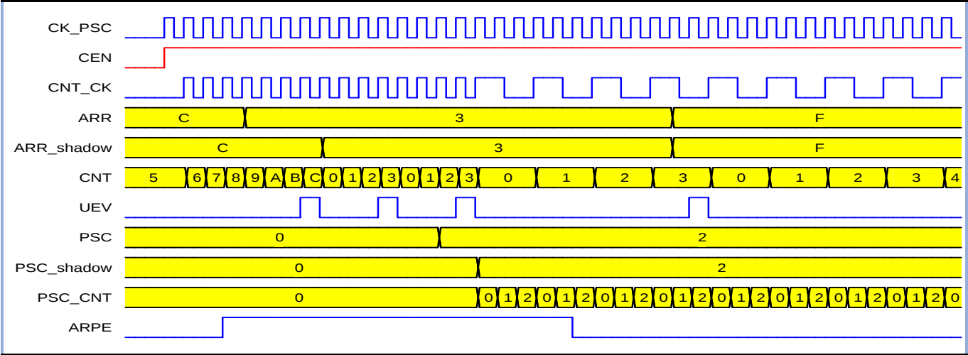
图 10-5 自动预转载
