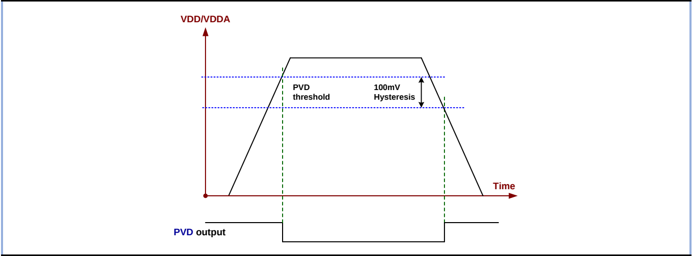
图 3-3 PVD 阈值波形图
