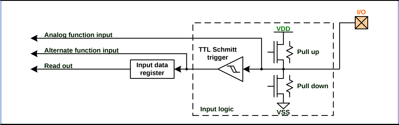
图 9-5 模拟输入
