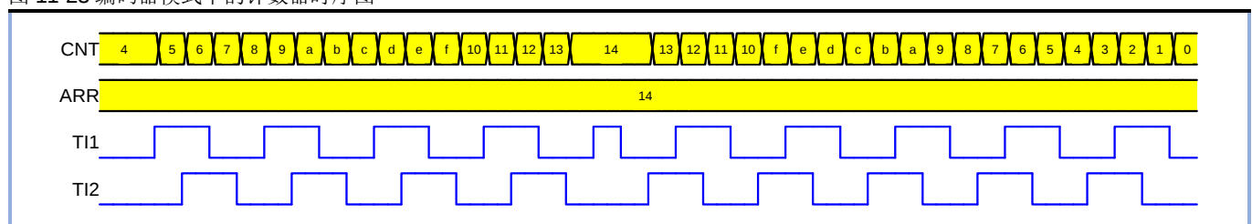
图 11-23 编码器模式下的计数器时序图
