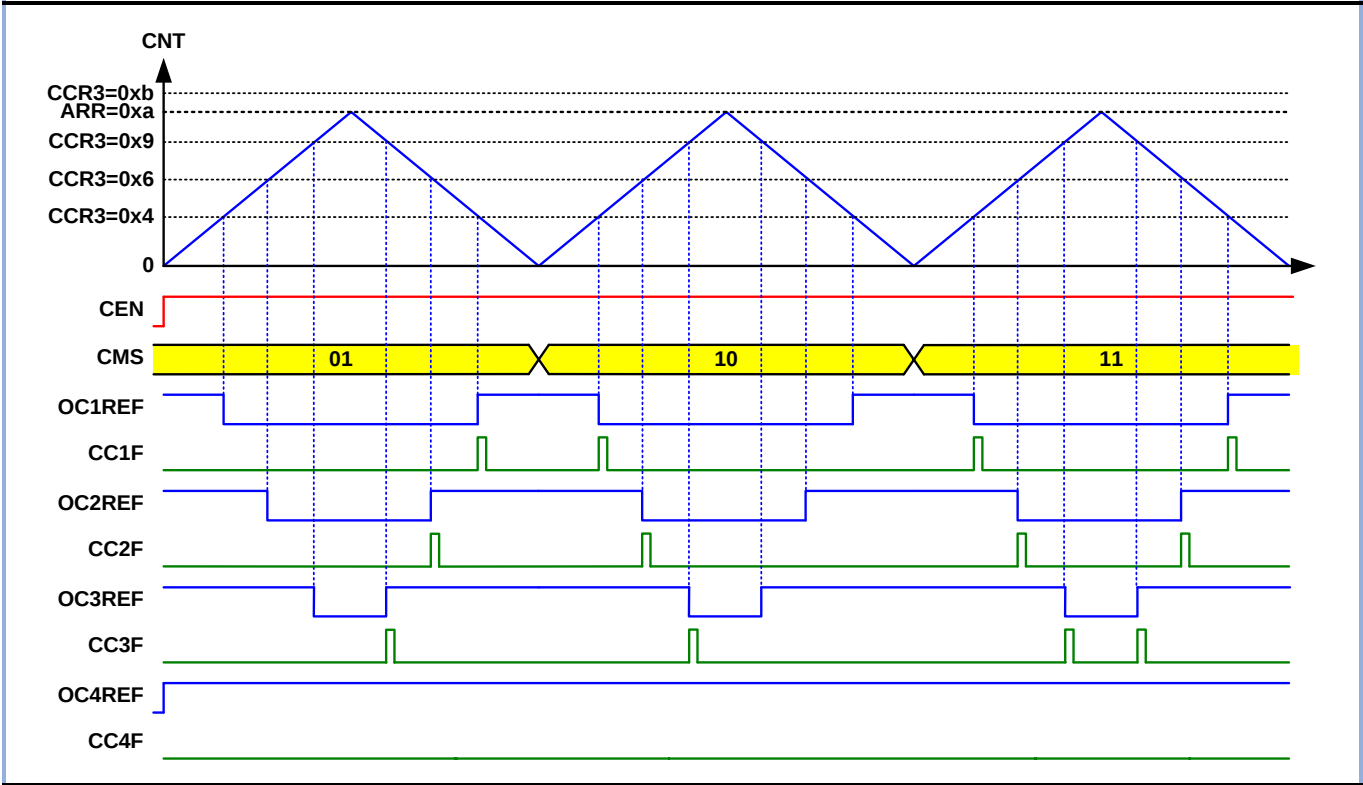
图 10-19 中心对齐 PWM 模式 1 的波形
