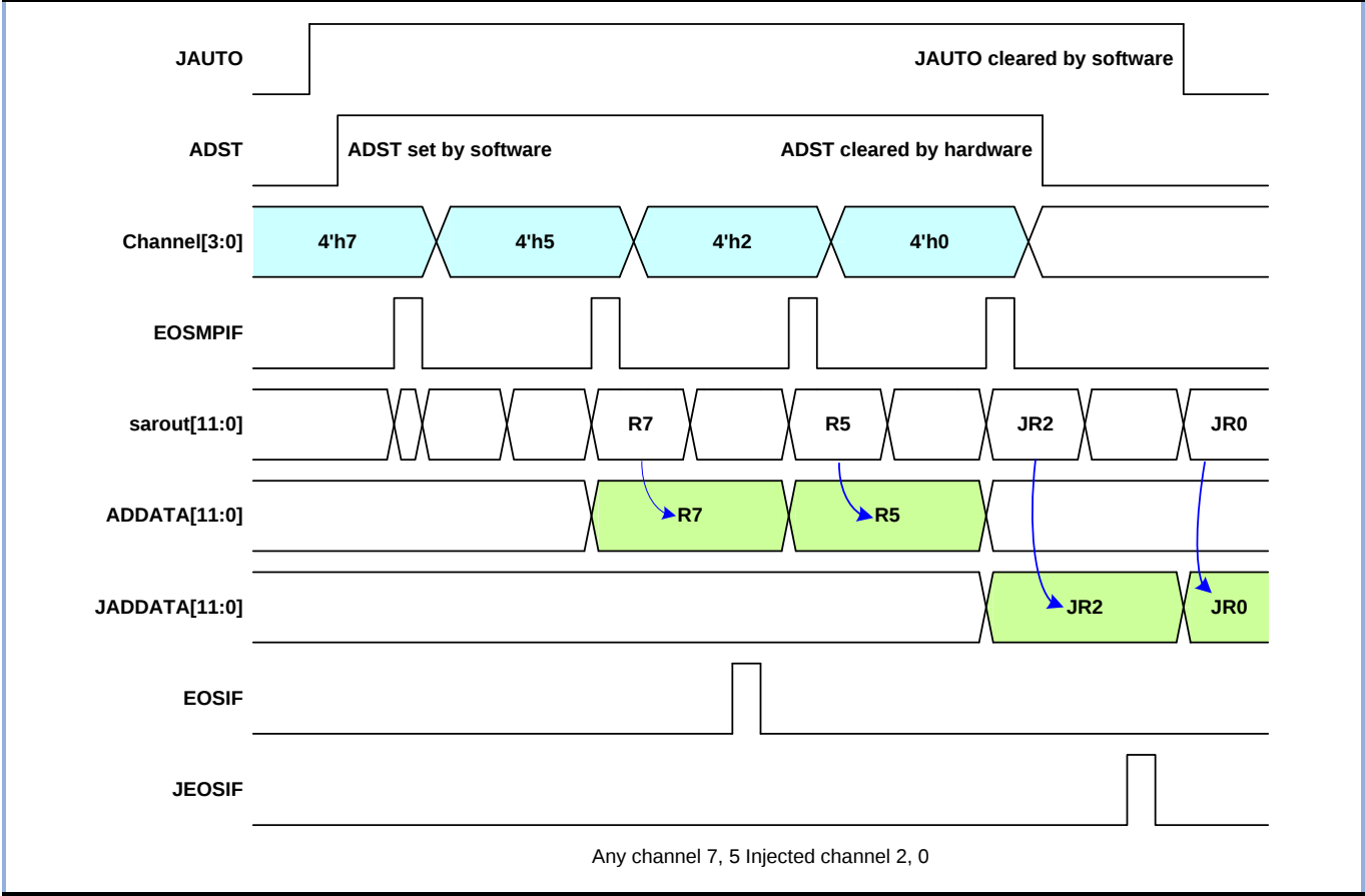
图 16-12 单周期扫描通道模式下自动注入通道转换时序图
