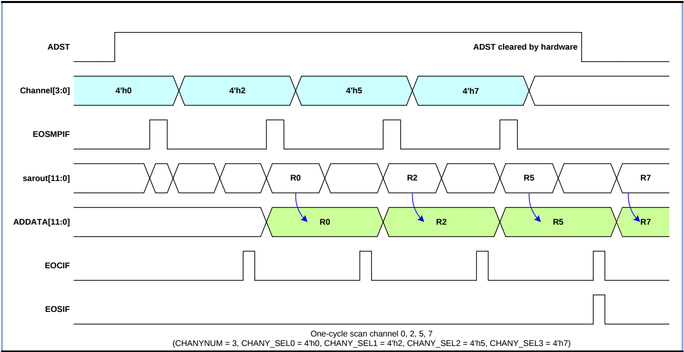
图 16-9 单周期扫描下通道转换时序图
