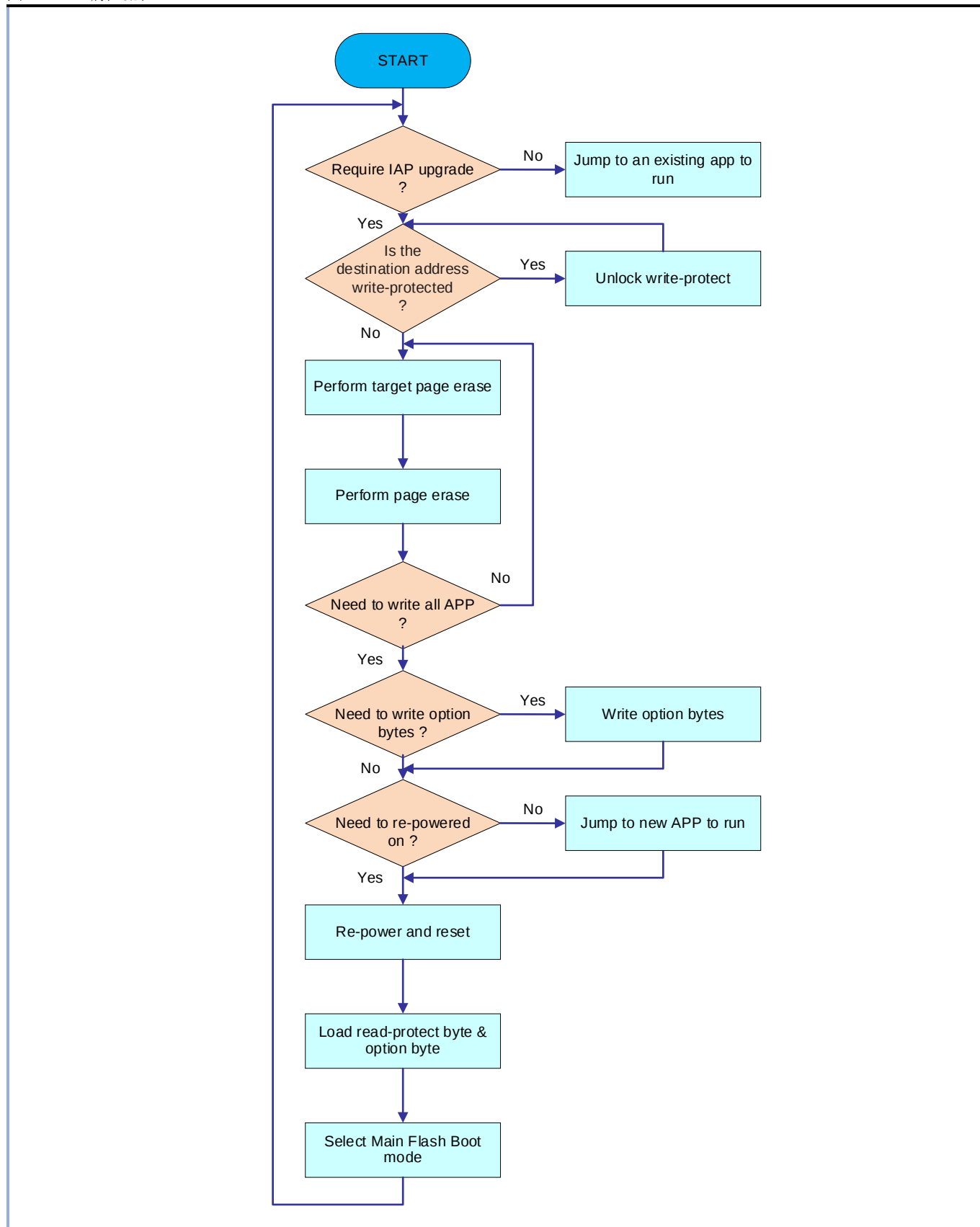
图 2-2 IAP 编程流程
