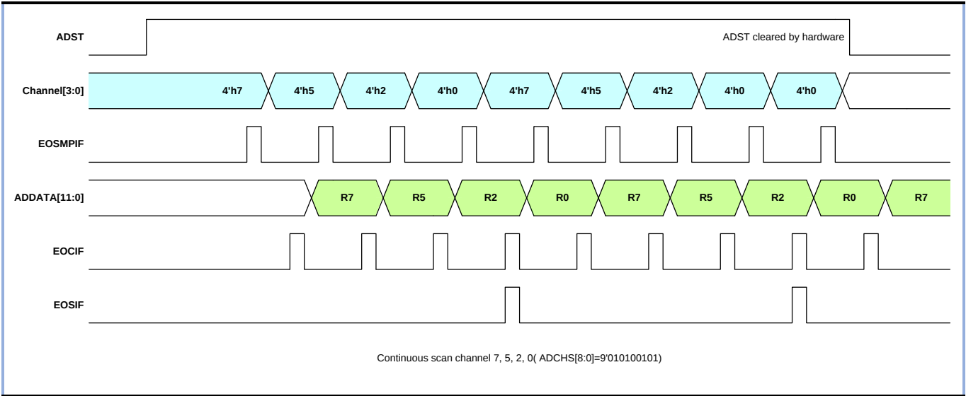
图 16-7 连续扫描模式使能通道转换时序图（通道方向由高到低）
