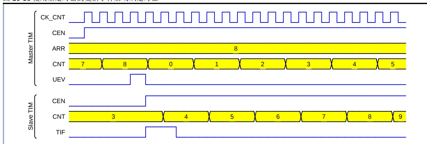
图 10-38 使用主定时器的更新事件启动从定时器
