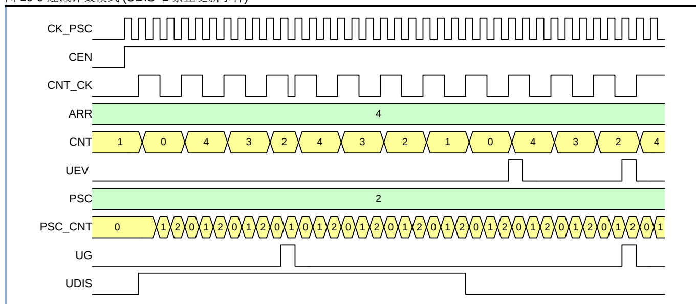
图 10-9 递减计数模式 (UDIS=1 禁止更新事件)
