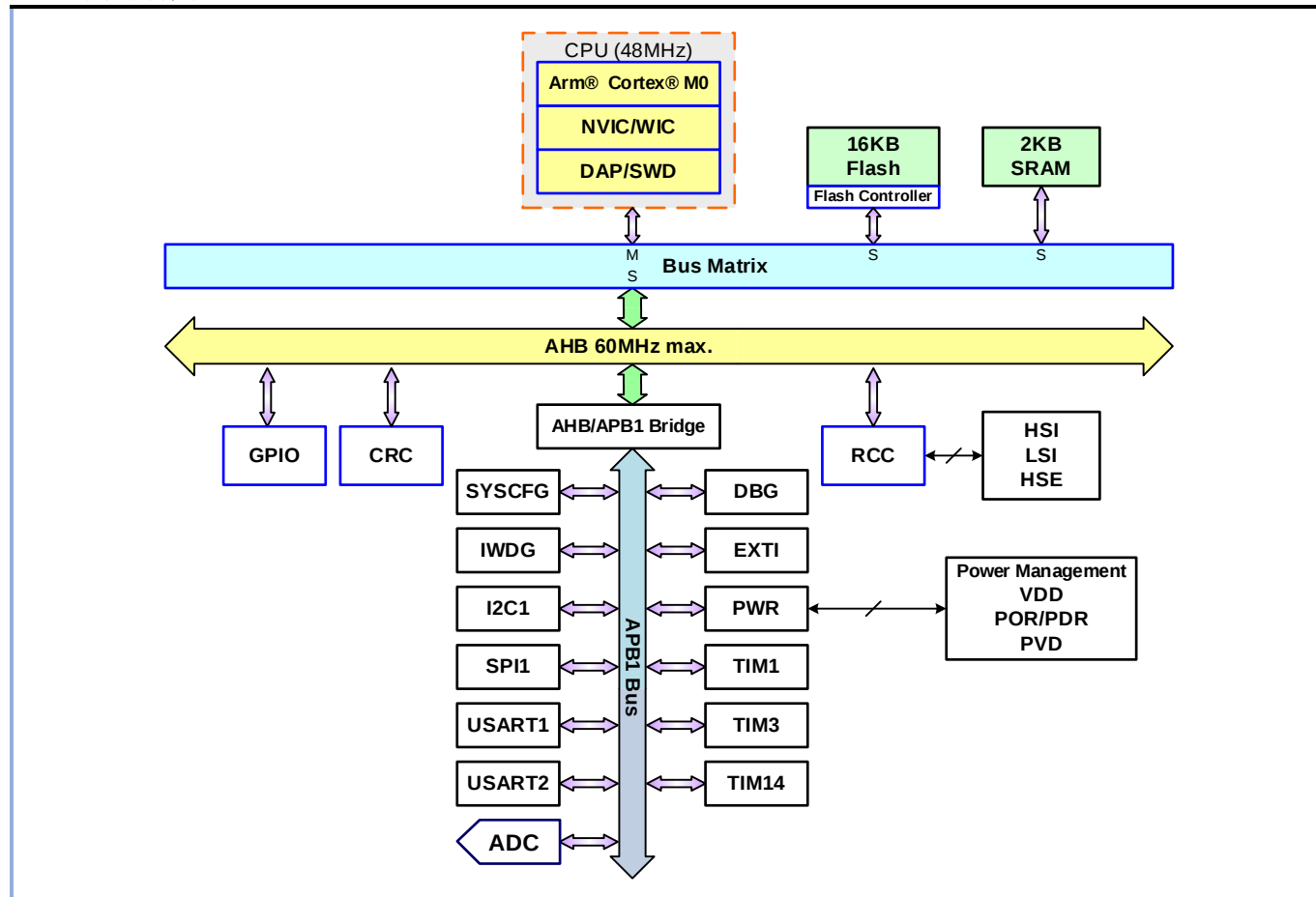
图 1-1 系统架构图
