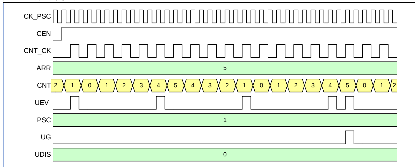
图 10-10 中央计数模式 (UDIS=0)
