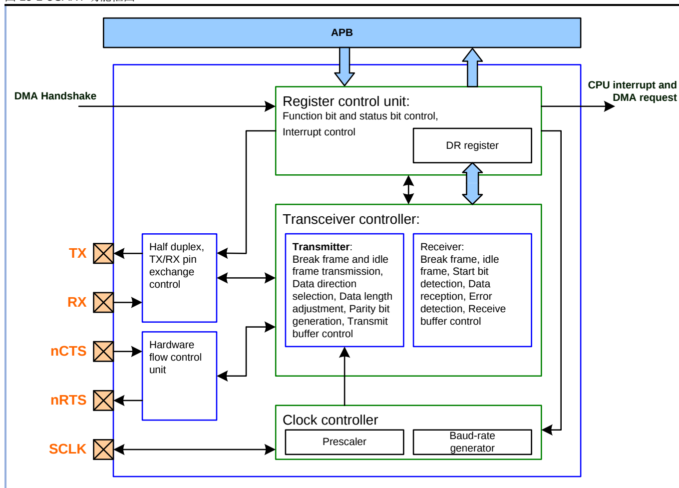
图 15-1 USART 功能框图
