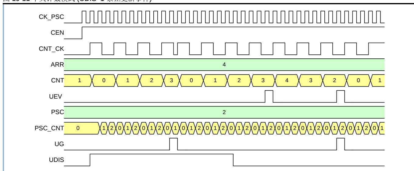
图 10-11 中央计数模式 (UDIS=1 禁止更新事件)
