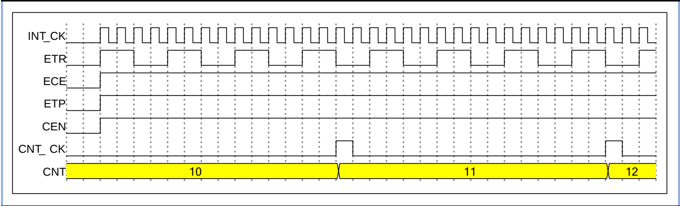
图 11-4 外部时钟模式 2 下的控制电路
