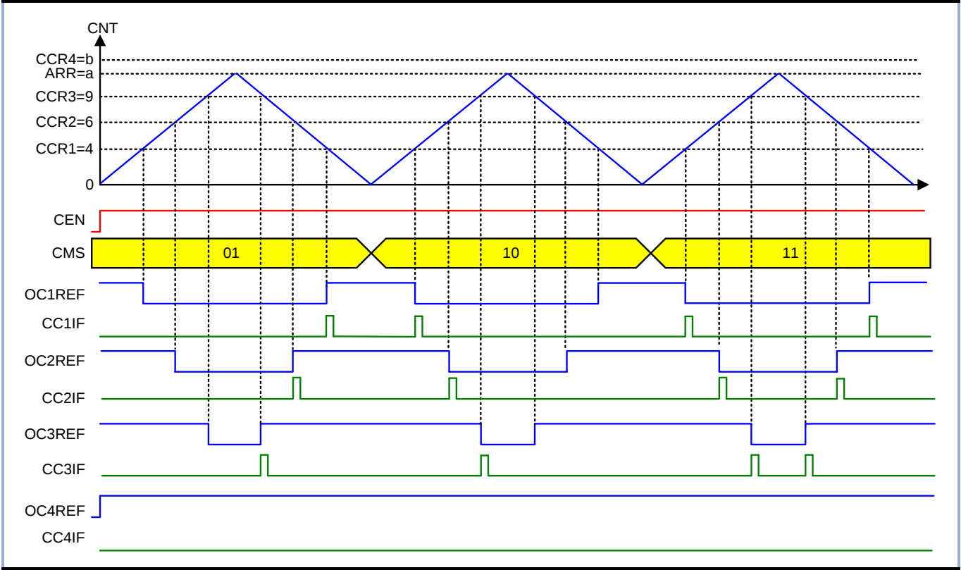
图 11-18 中心对齐 PWM 模式 1 的波形
