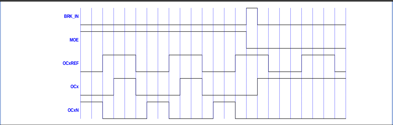
图 10-28 响应刹车输出 (OISx=1, OISxN=1)
