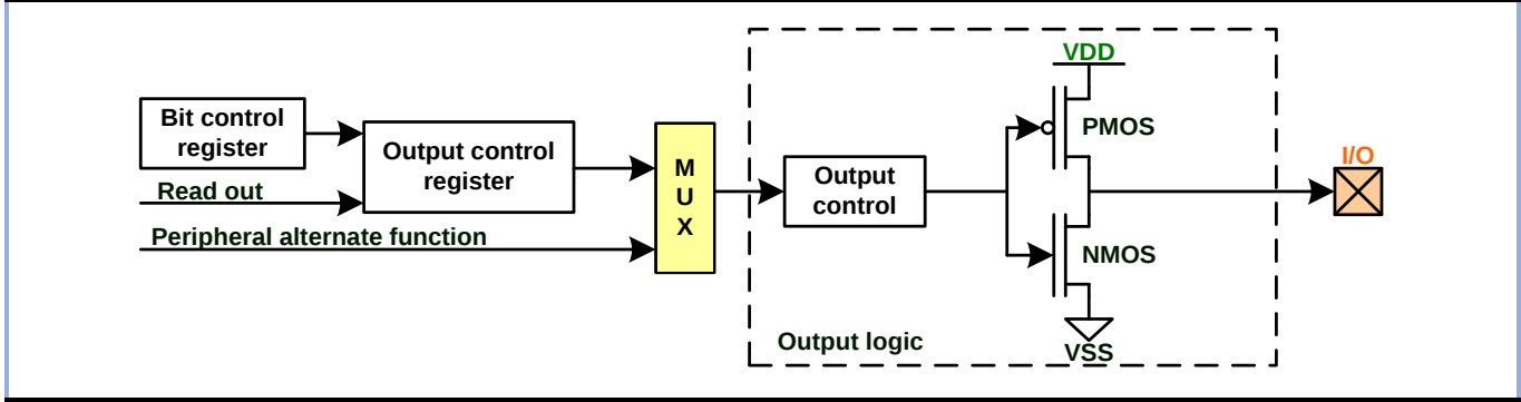
图 9-3 输出配置
