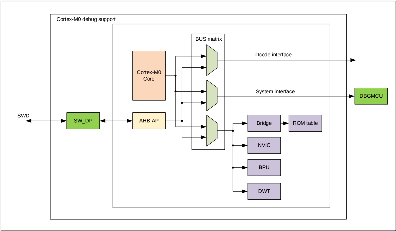
图 19-1 调试功能框图
