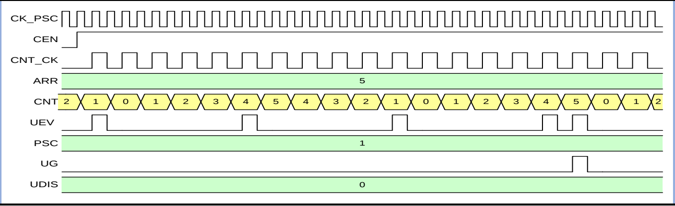
图 11-10 中心计数模式 (UDIS=0)
