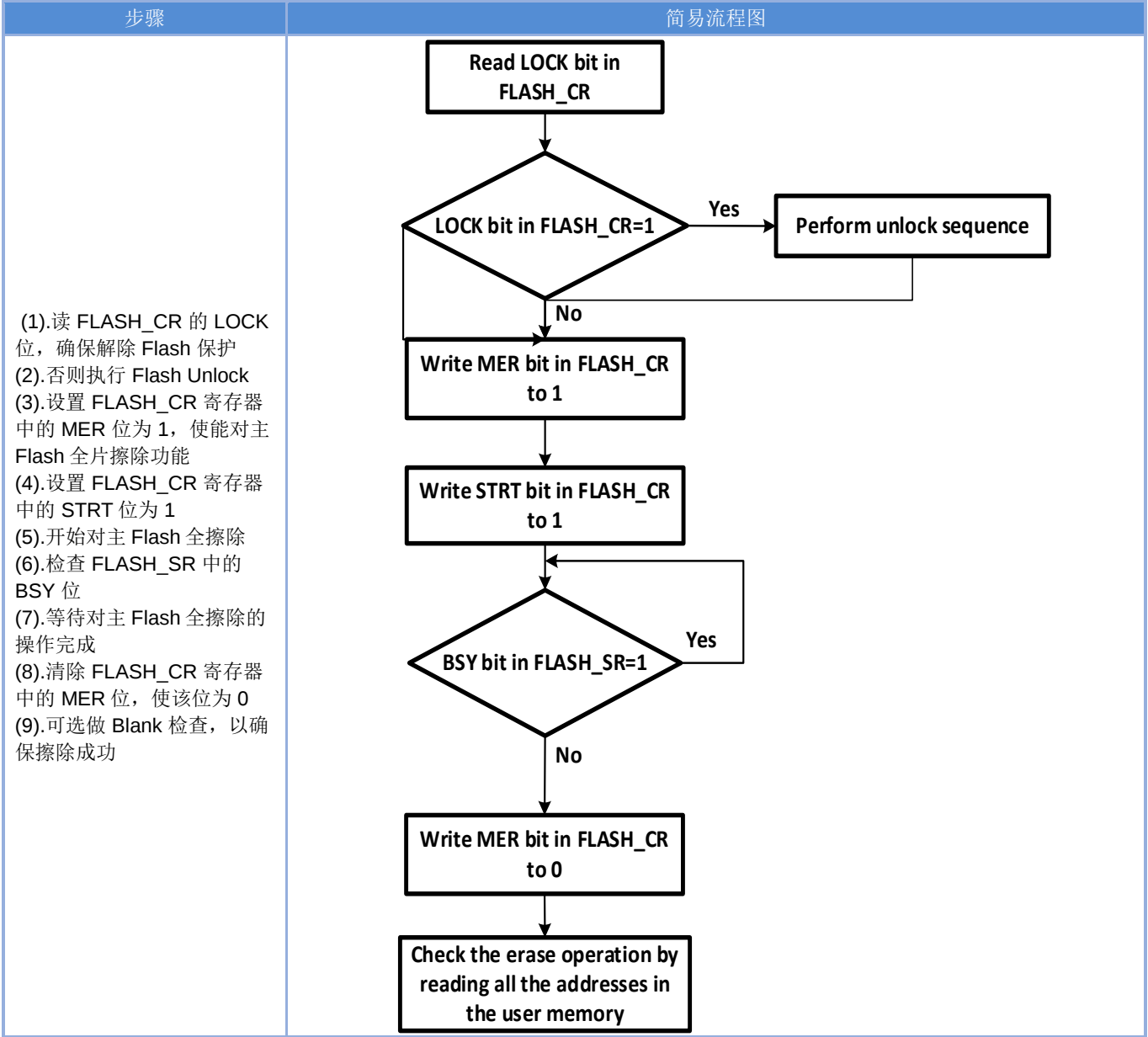
主 Flash 存储器擦除流程:
