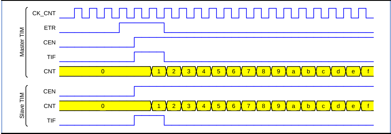
图 10-39 主定时器 TIM1 同步启动主定时器和从定时器
