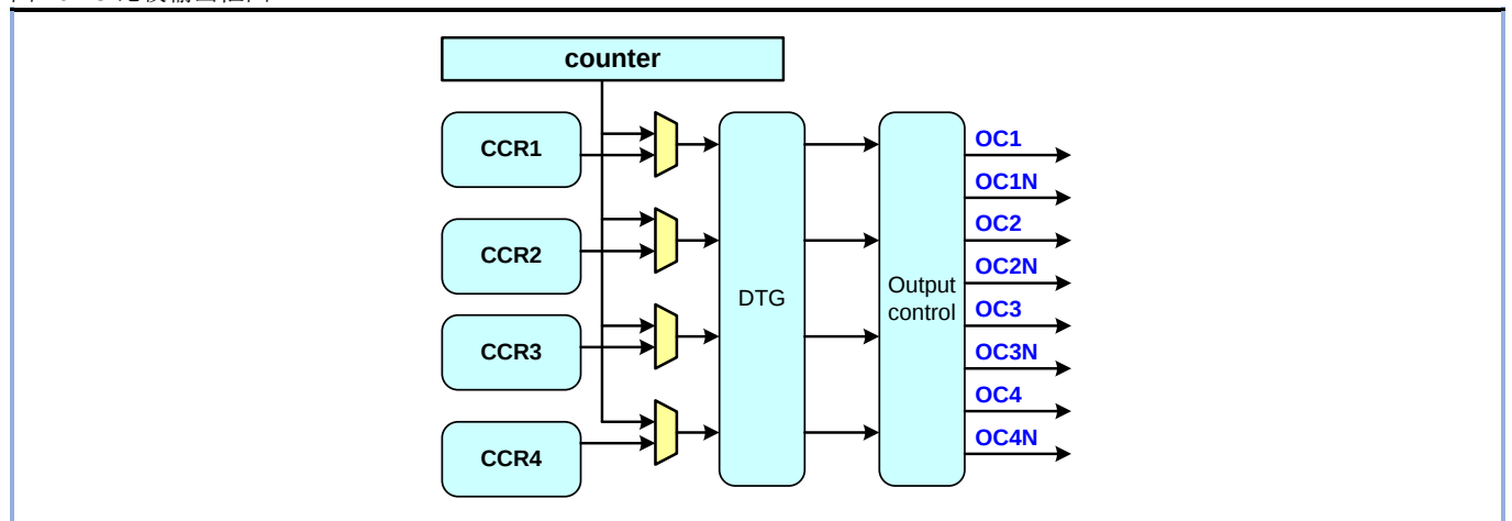
图 10-15 比较输出框图
