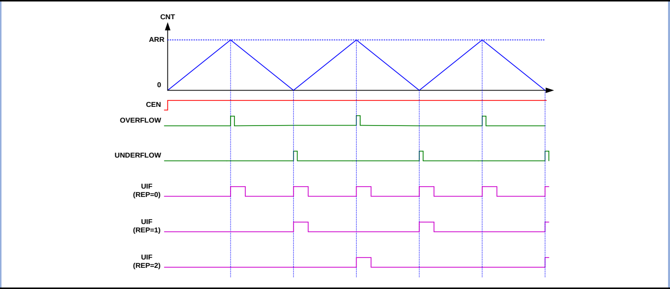
图 10-12 中心对齐模式重复计数时序图
