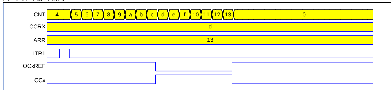
图 10-30 单脉冲模式
