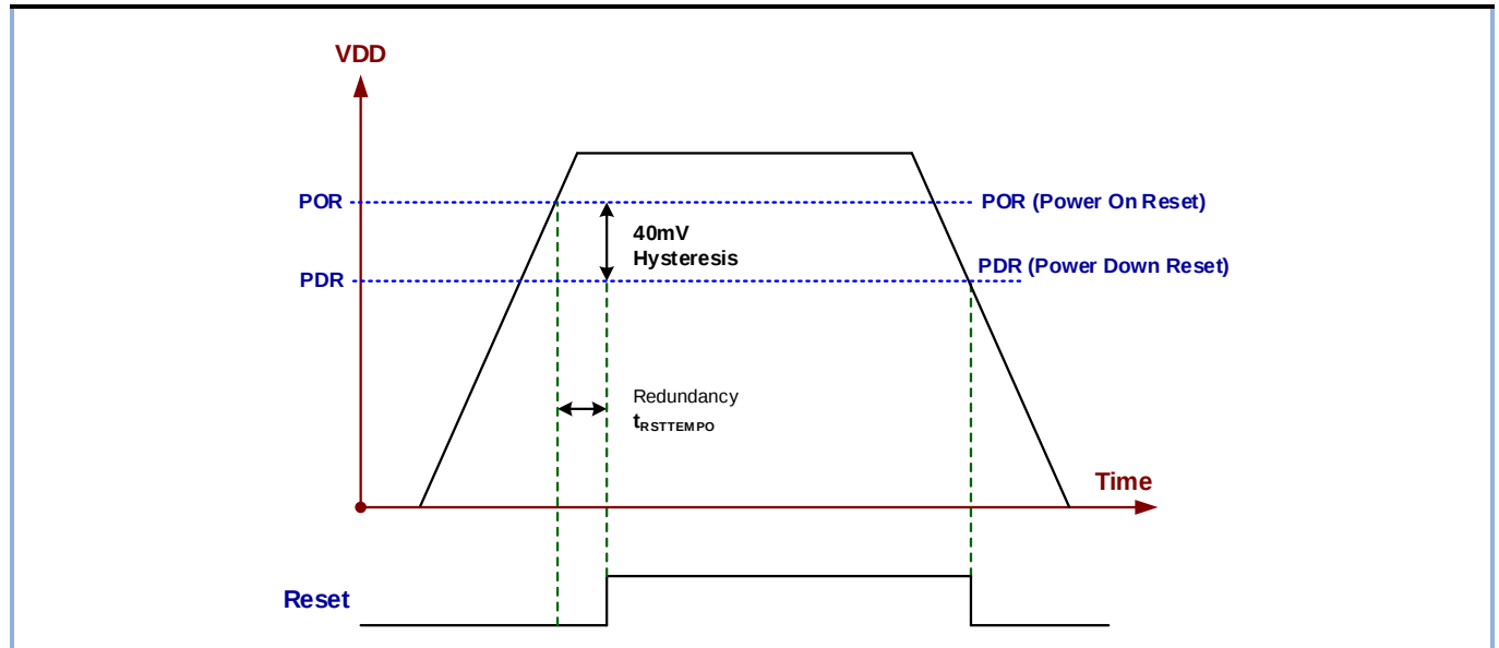
图 3-2 上电复位和掉电复位波形图
