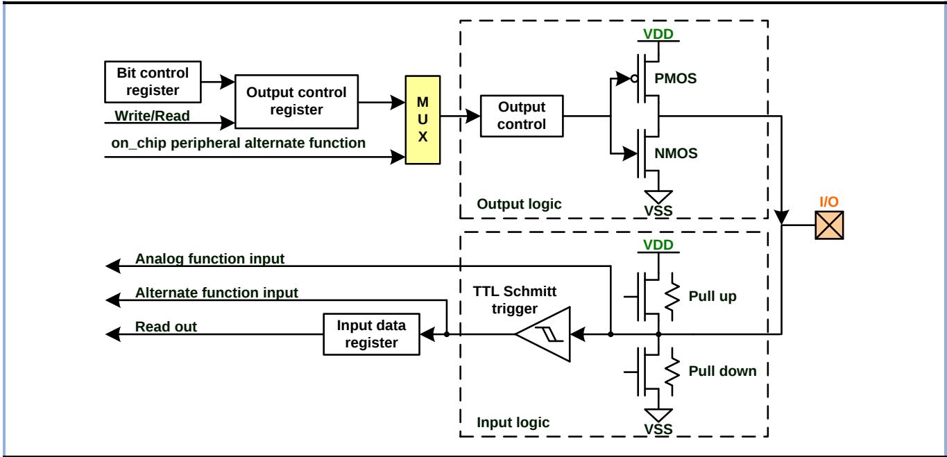
图 9-1 标准 I/O 端口
