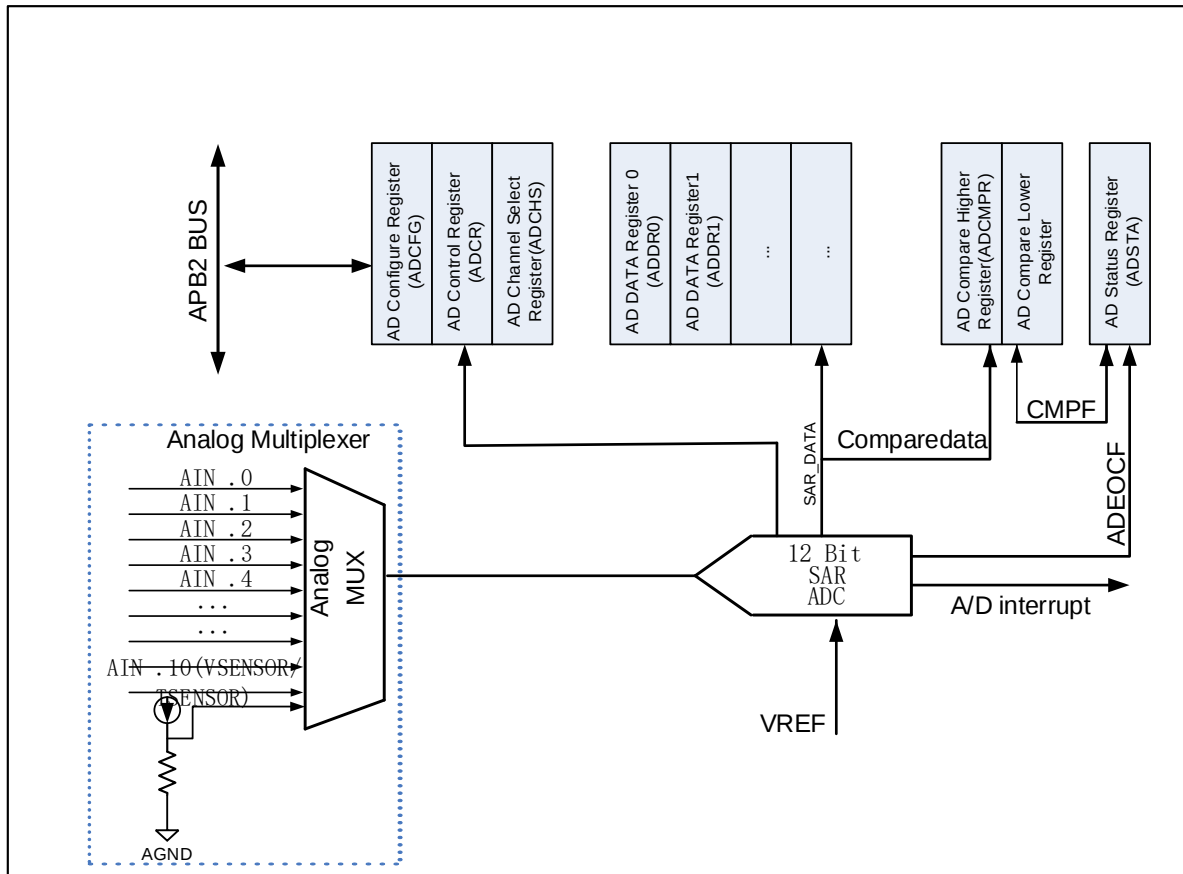
图 16-1 ADC 系统框图
