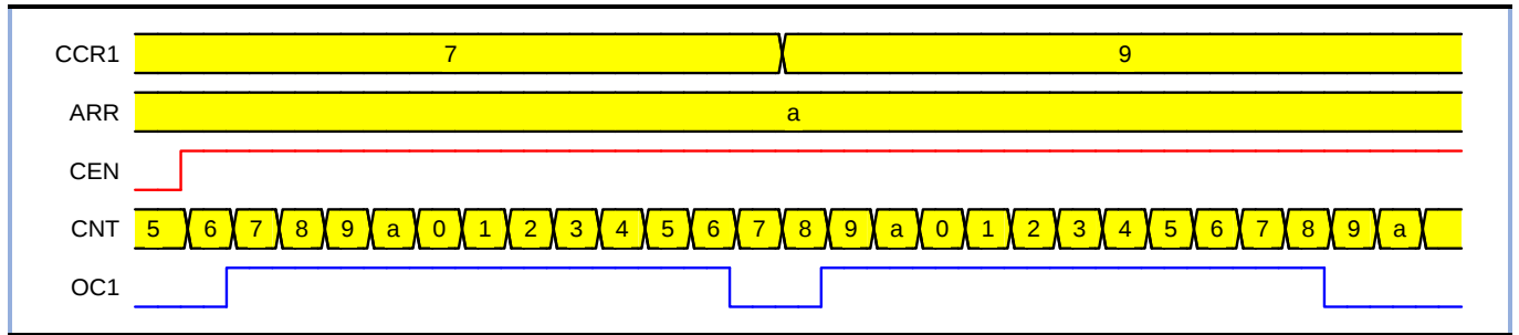
图 13-7 比较输出模式，OC1 信号在匹配时翻转
