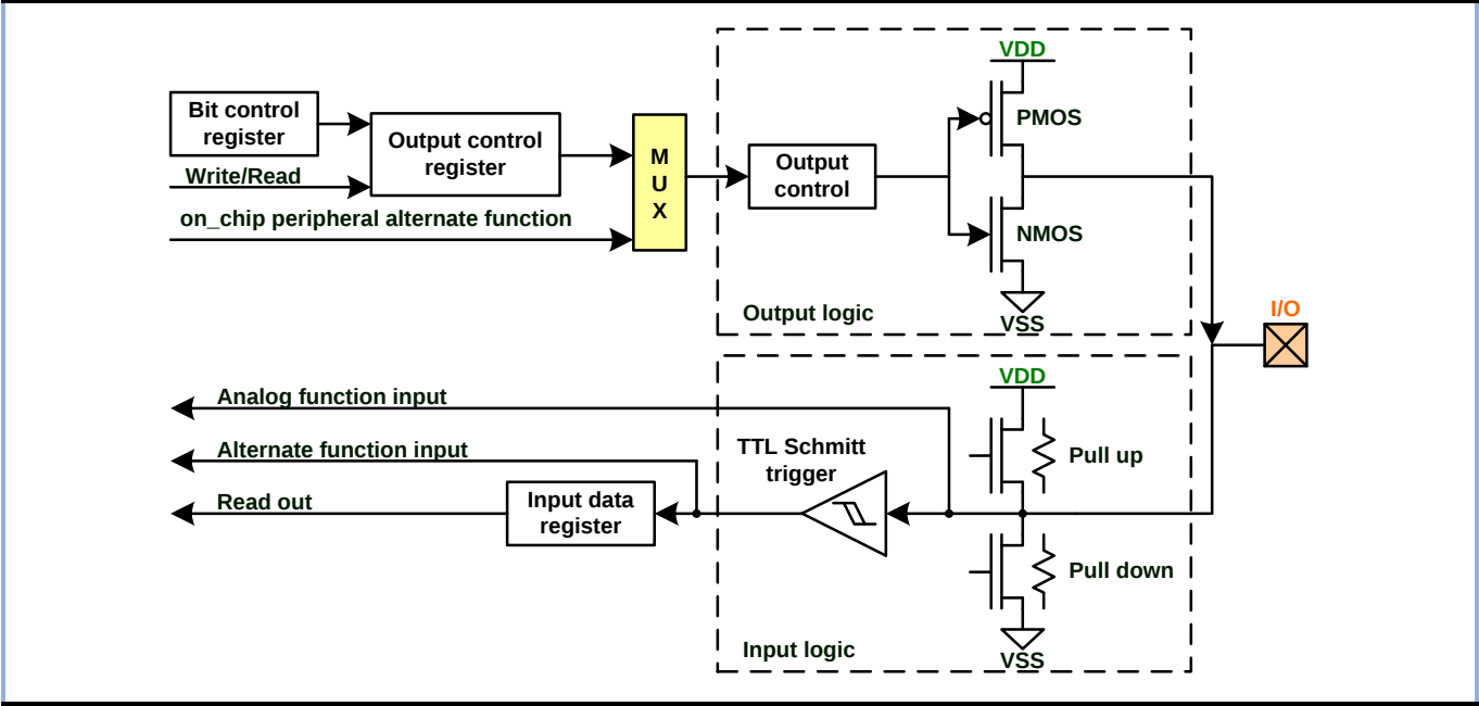
图 9-4 复用功能配置
