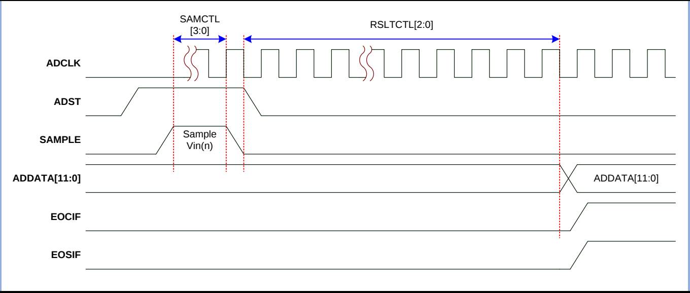
图 16-8 单次转换模式下通道转换时序图
