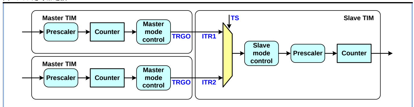
图 10-35 定时器连接
