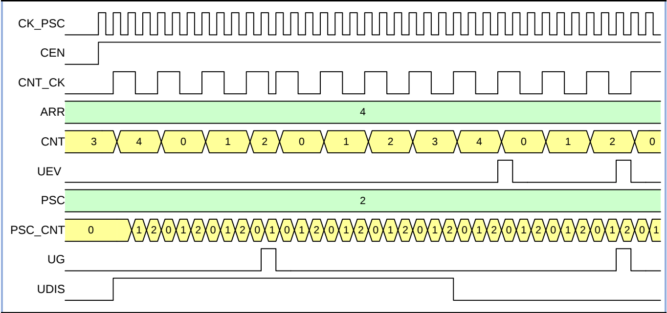
图 11-7 递增计数模式 (UDIS =1, 禁止更新事件)
