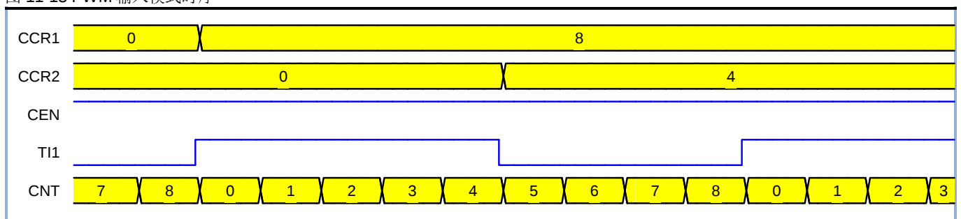
图 11-13 PWM 输入模式时序
