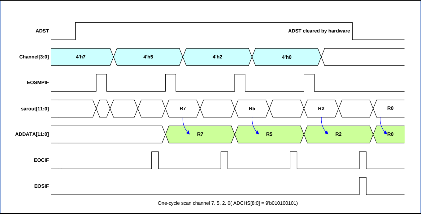
图 16-4 单周期扫描下使能通道转换时序图（通道方向从高到低）
