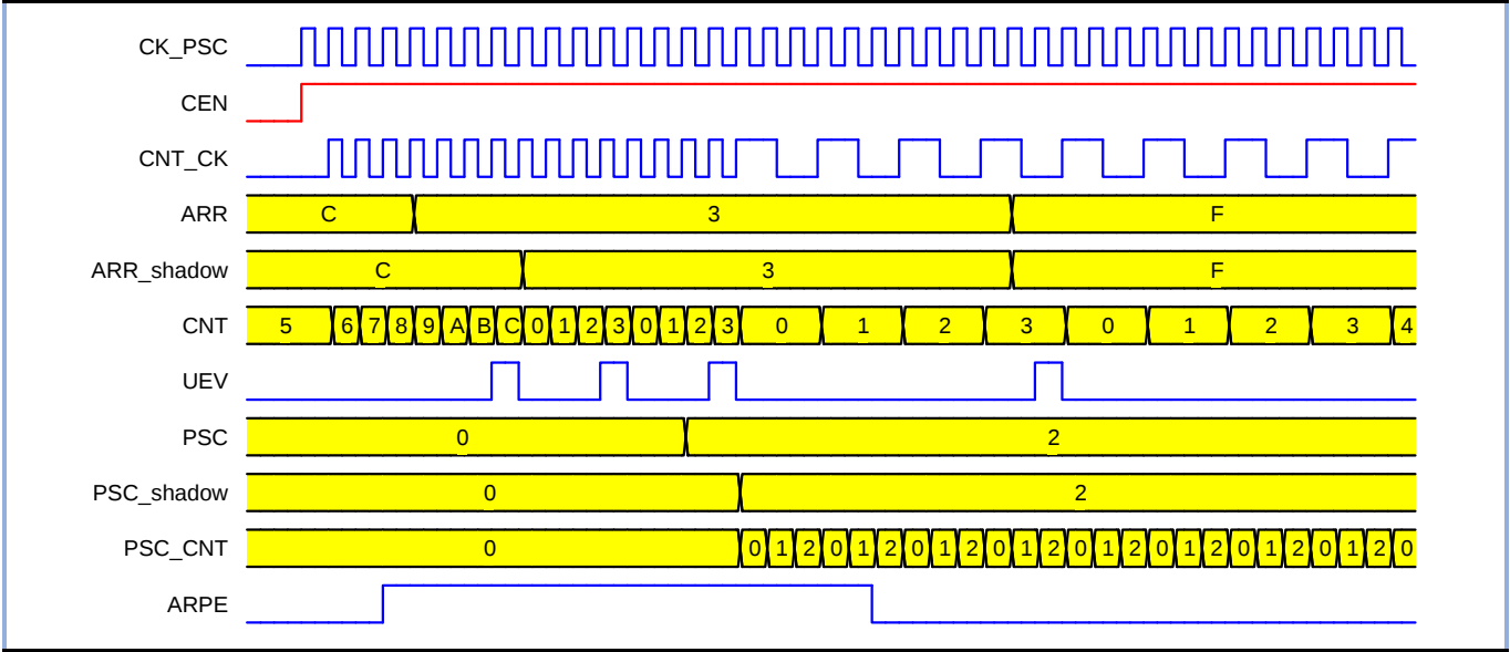
图 13-2 自动预加载
