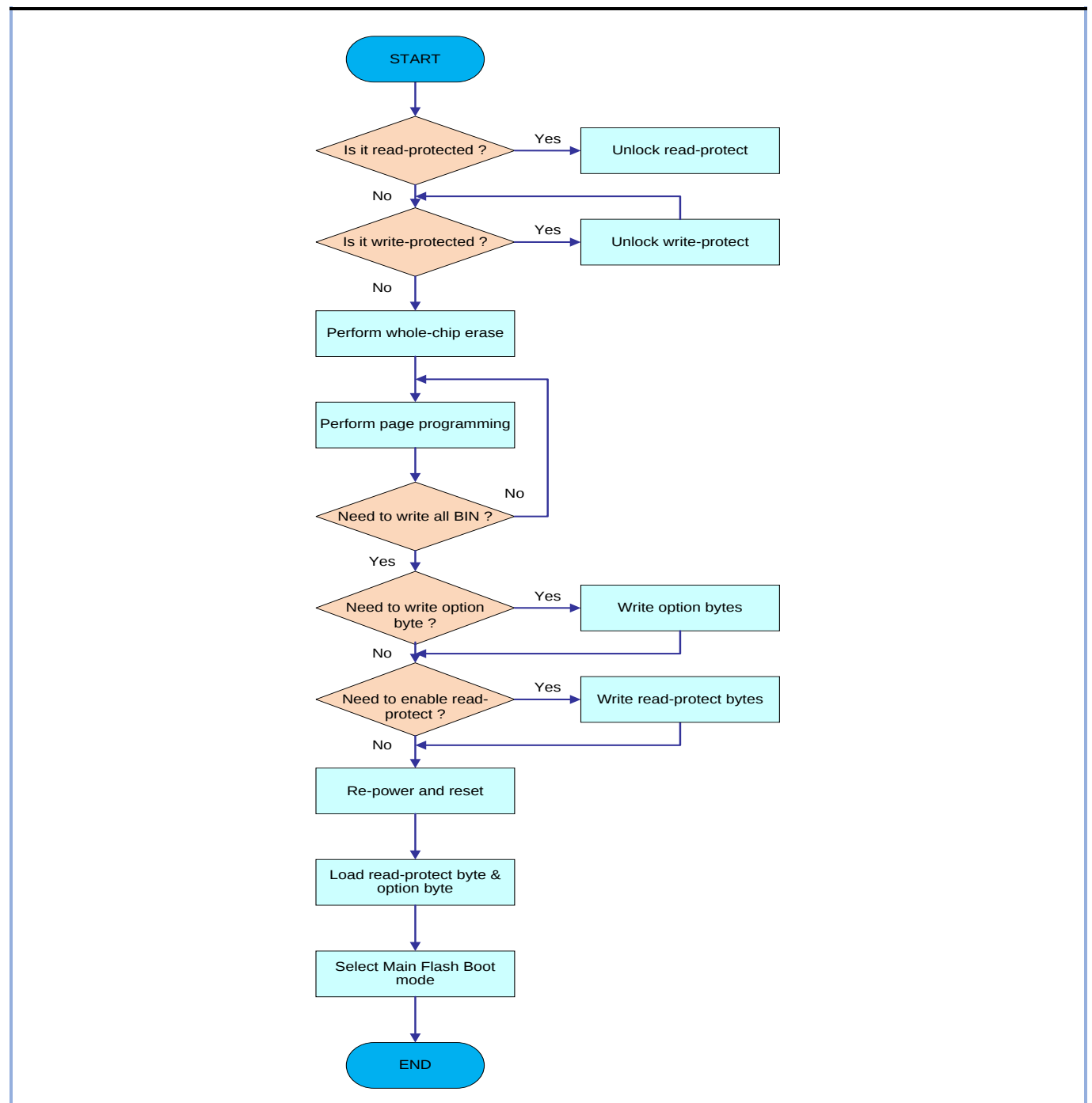
图 2-1 ISP 编程流程
