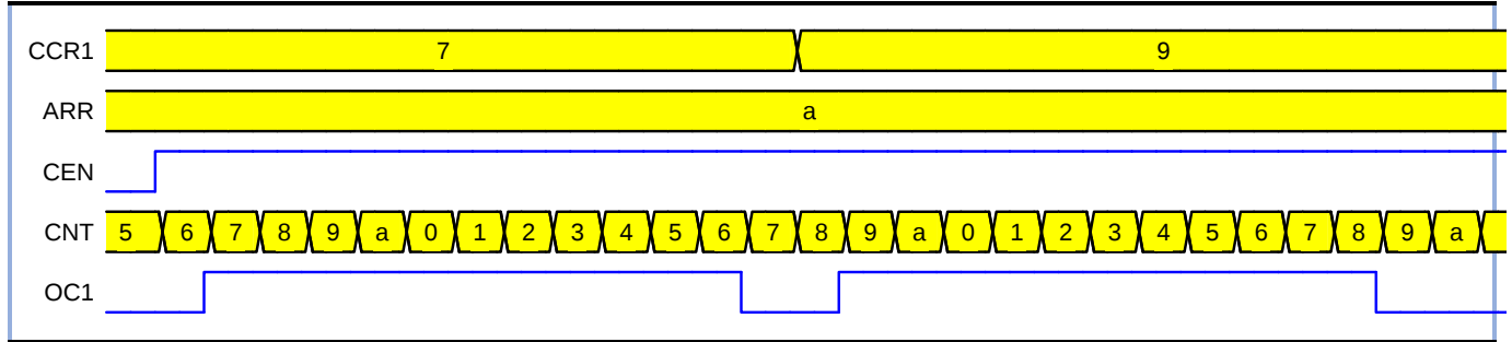
图 11-15 比较输出模式，OC1 信号在匹配时翻转
