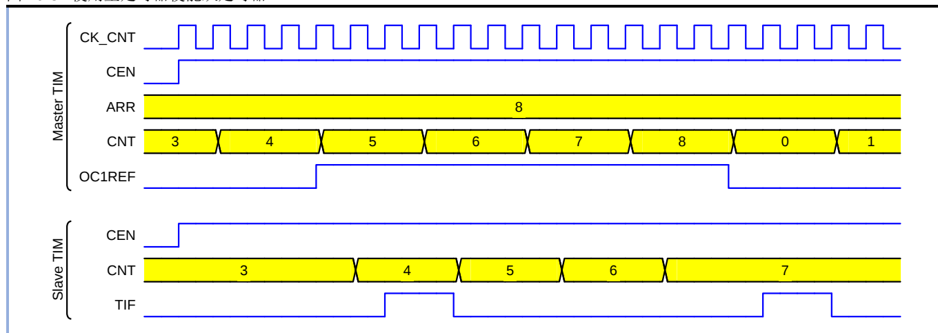
图 10-37 使用主定时器使能从定时器
