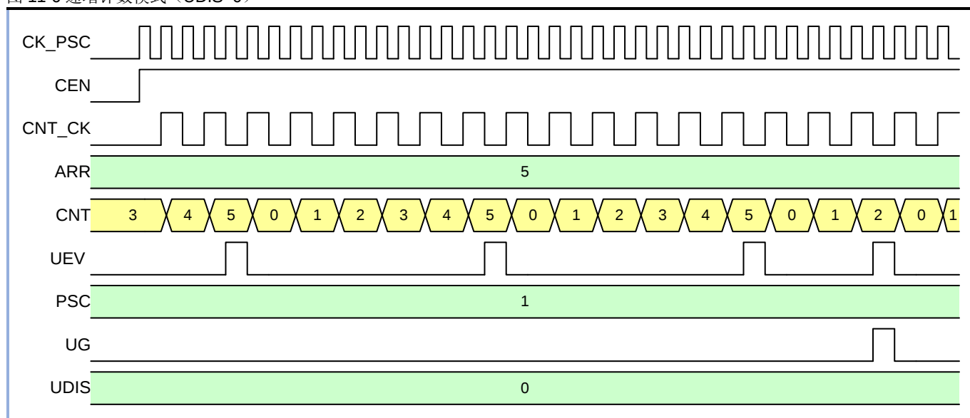
图 11-6 递增计数模式 (UDIS=0)
