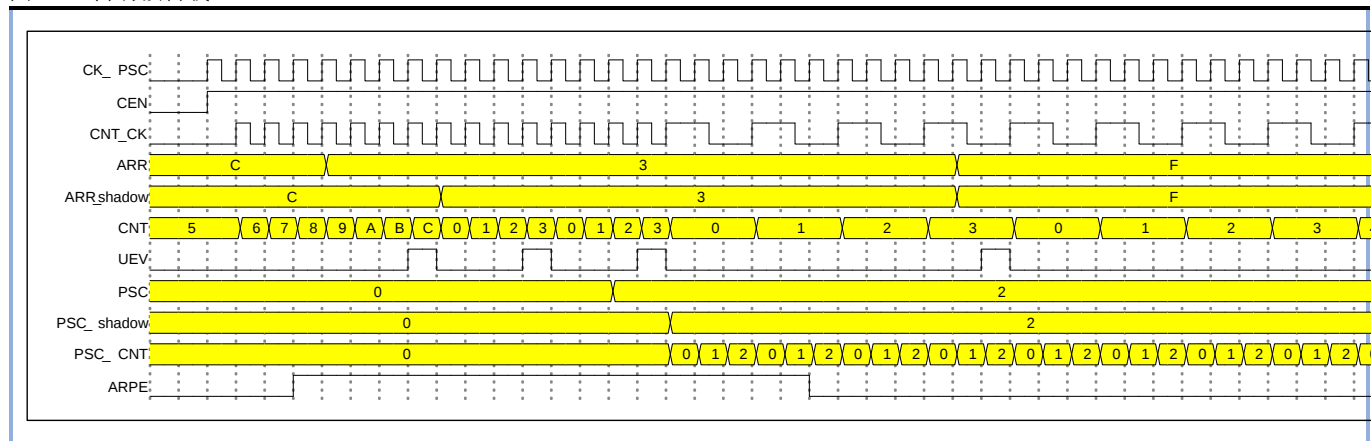
图 11-5 自动预转载
