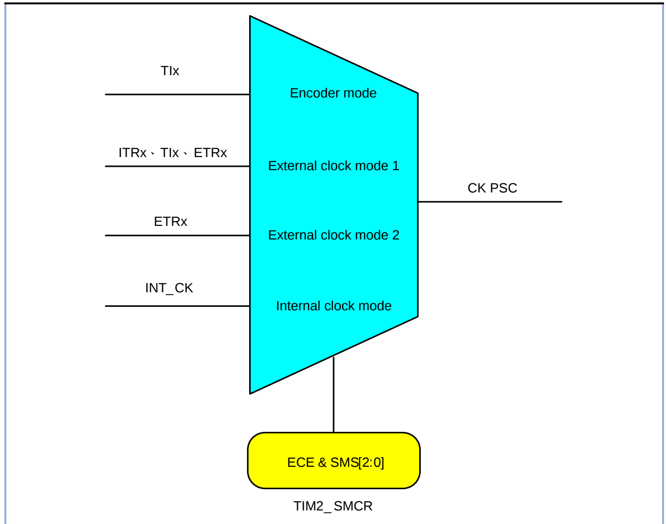
图 11-2 时钟选择
