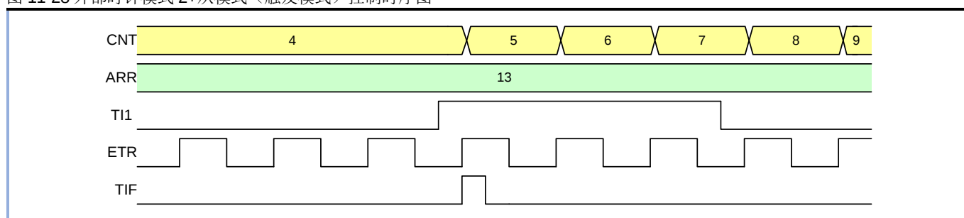
图 11-28 外部时钟模式 2+从模式（触发模式）控制时序图
