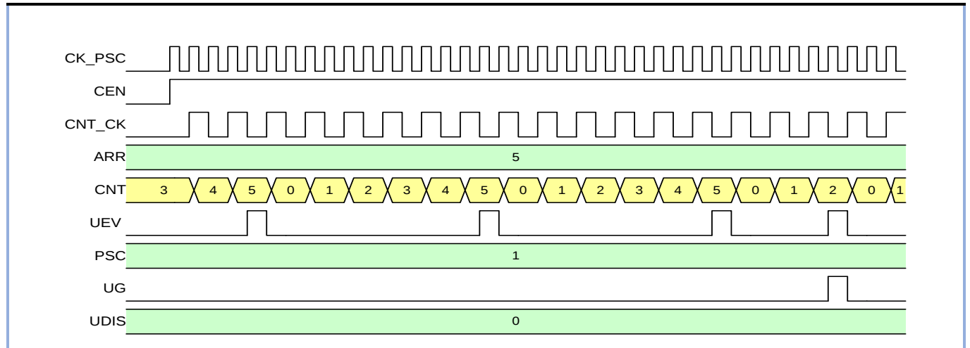
图 10-6 递增计数模式 (UDIS=0)
