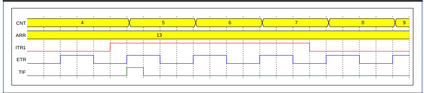
图 10-34 外部时钟模式 2+从模式(触发模式)控制时序图
