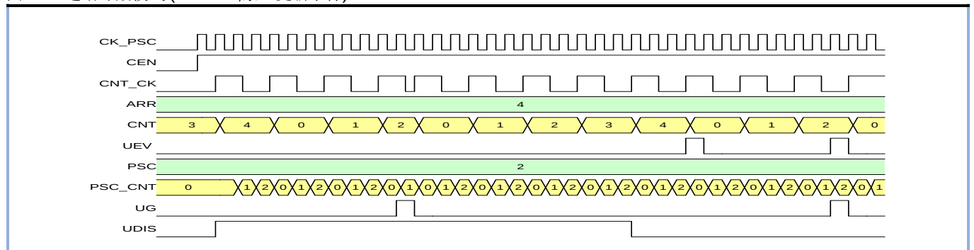
图 10-7 递增计数模式 (UDIS =1,禁止更新事件)
