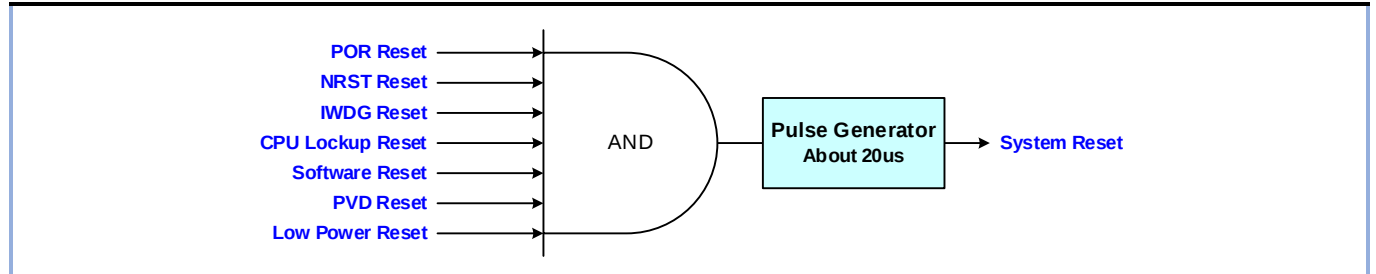
图 4-1 复位功能框图
