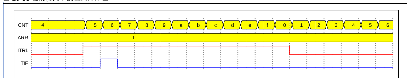
图 10-33 触发模式下的控制时序图
