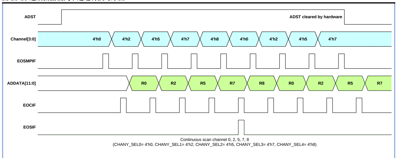
图 16-10 连续扫描模式下通道转换时序图
