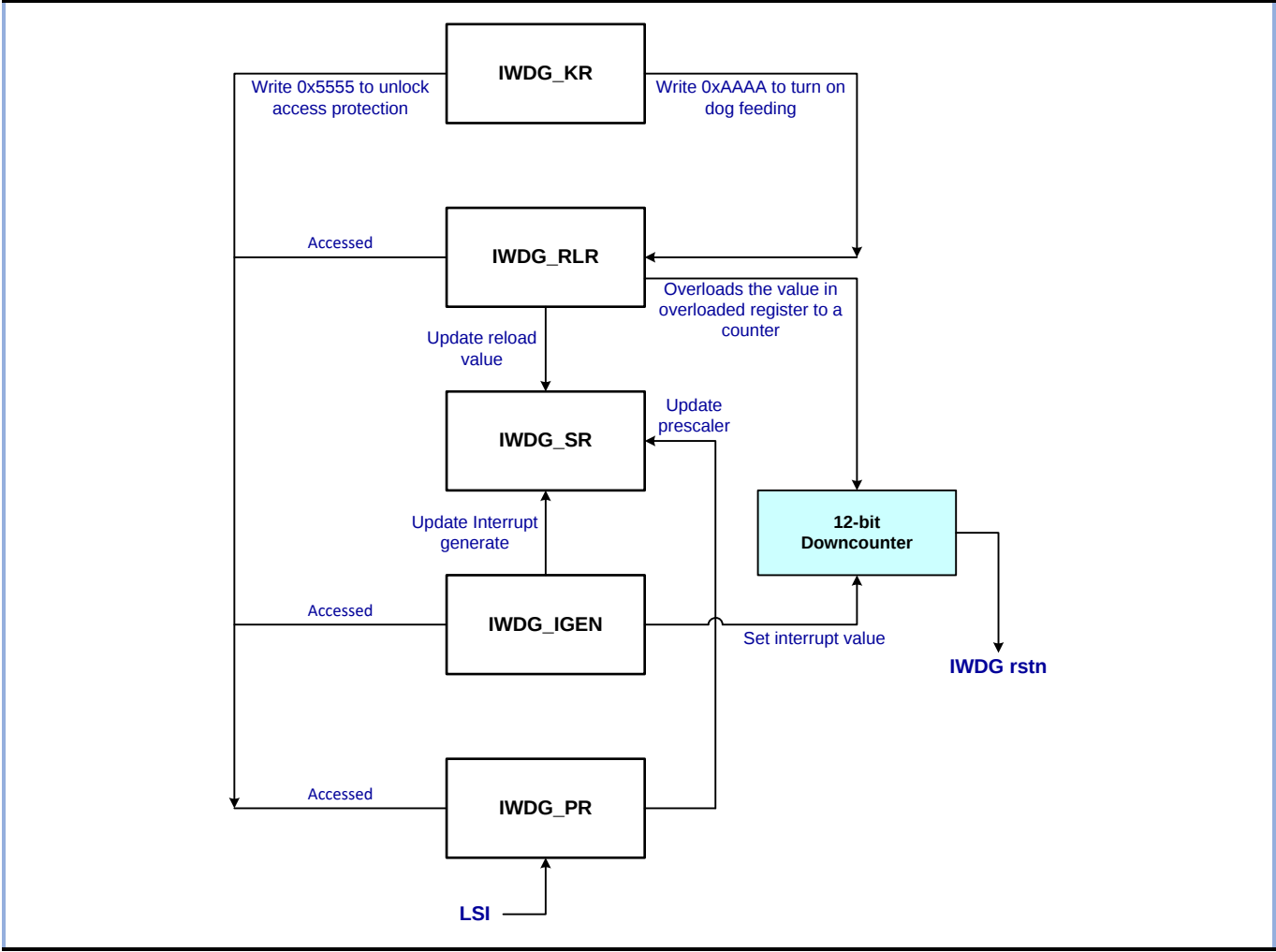
图 14-2 流程框图
