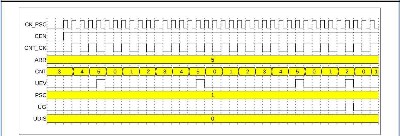
图 12-2 自动预转载
