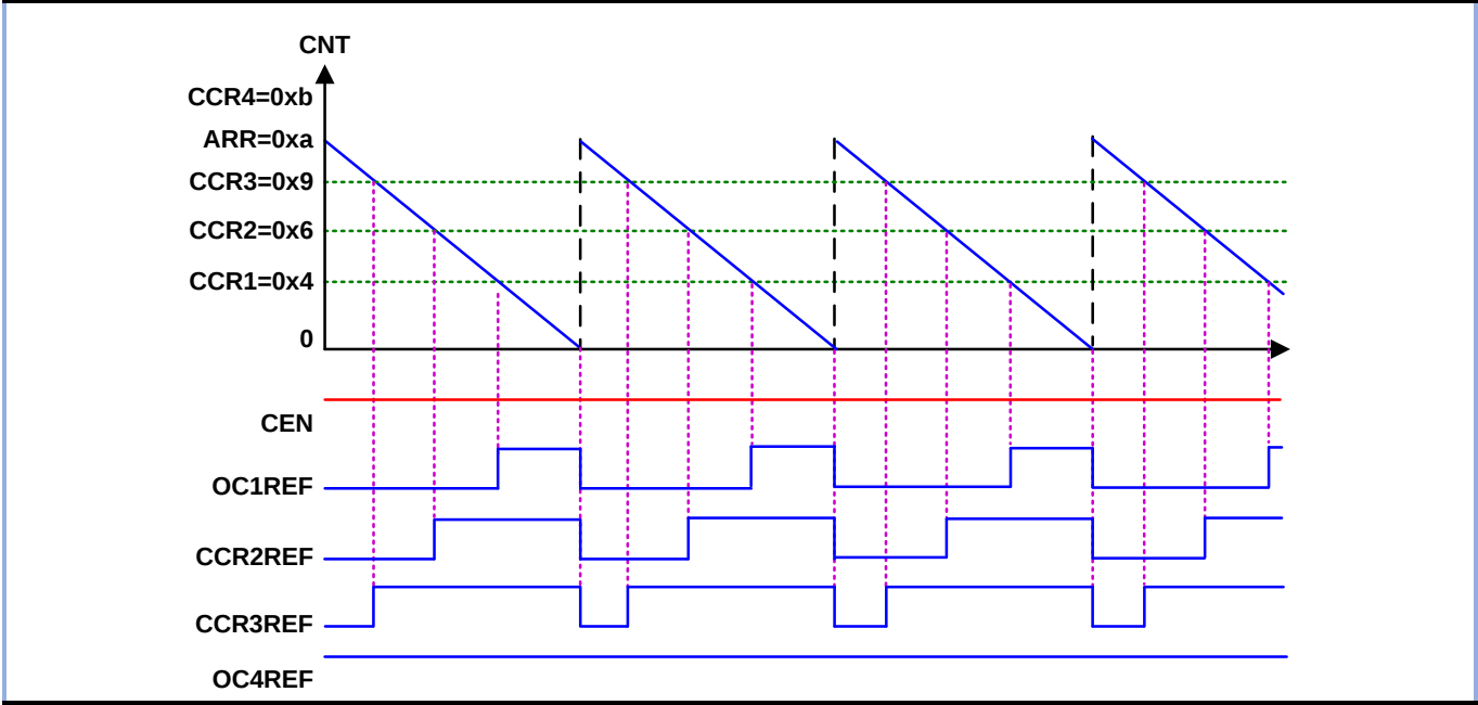
图 10-18 边沿对齐递减计数时 PWM 模式 1 的波形
