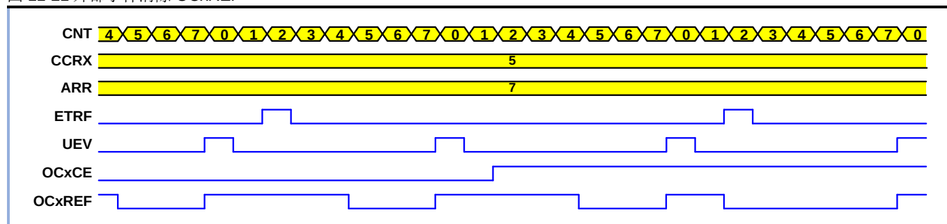
图 11-21 外部事件清除 OCxREF
