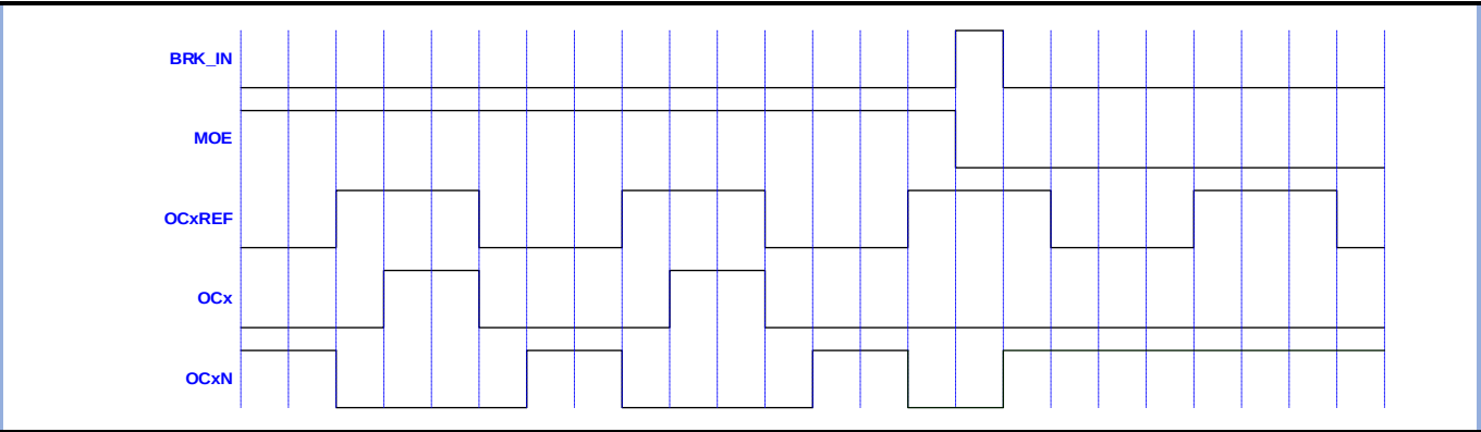
图 10-27 响应刹车输出 (OISx=1,OISxN=0)
