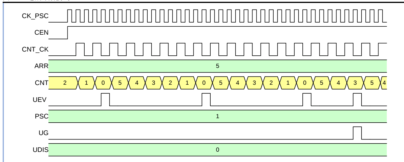
图 10-8 递减计数模式 (UDIS=0)
