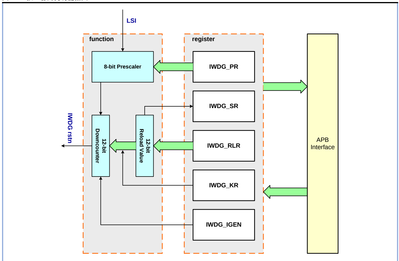
图 14-1 独立看门狗功能框图
