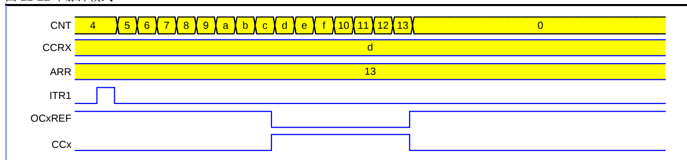
图 11-22 单脉冲模式
