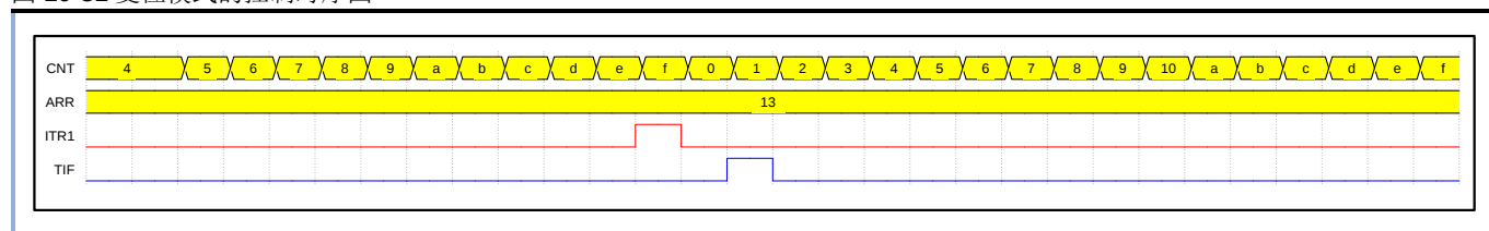
图 10-31 复位模式的控制时序图
