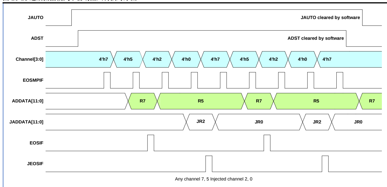
图 16-13 连续扫描模式下自动注入转换时序图
