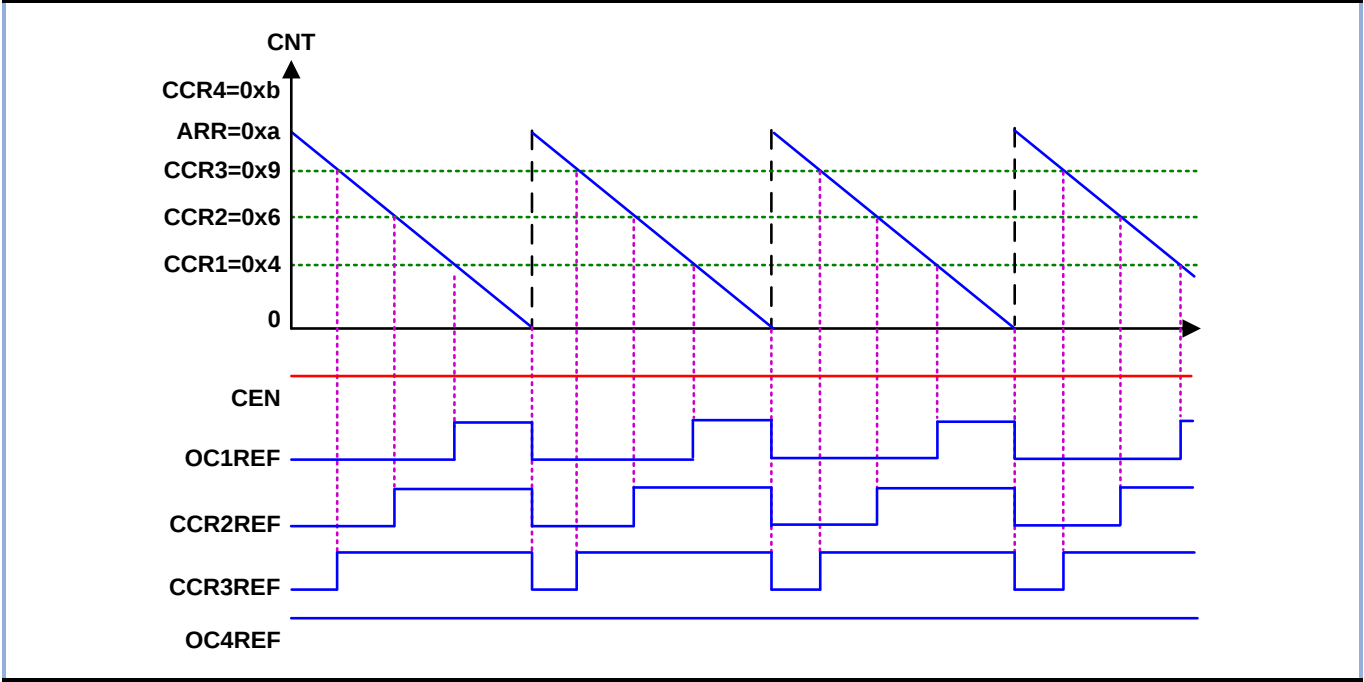
图 11-17 边沿对齐递减计数时 PWM 模式 1 的波形
