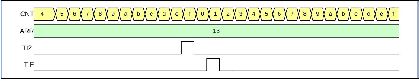
图 11-25 复位模式的控制时序图
