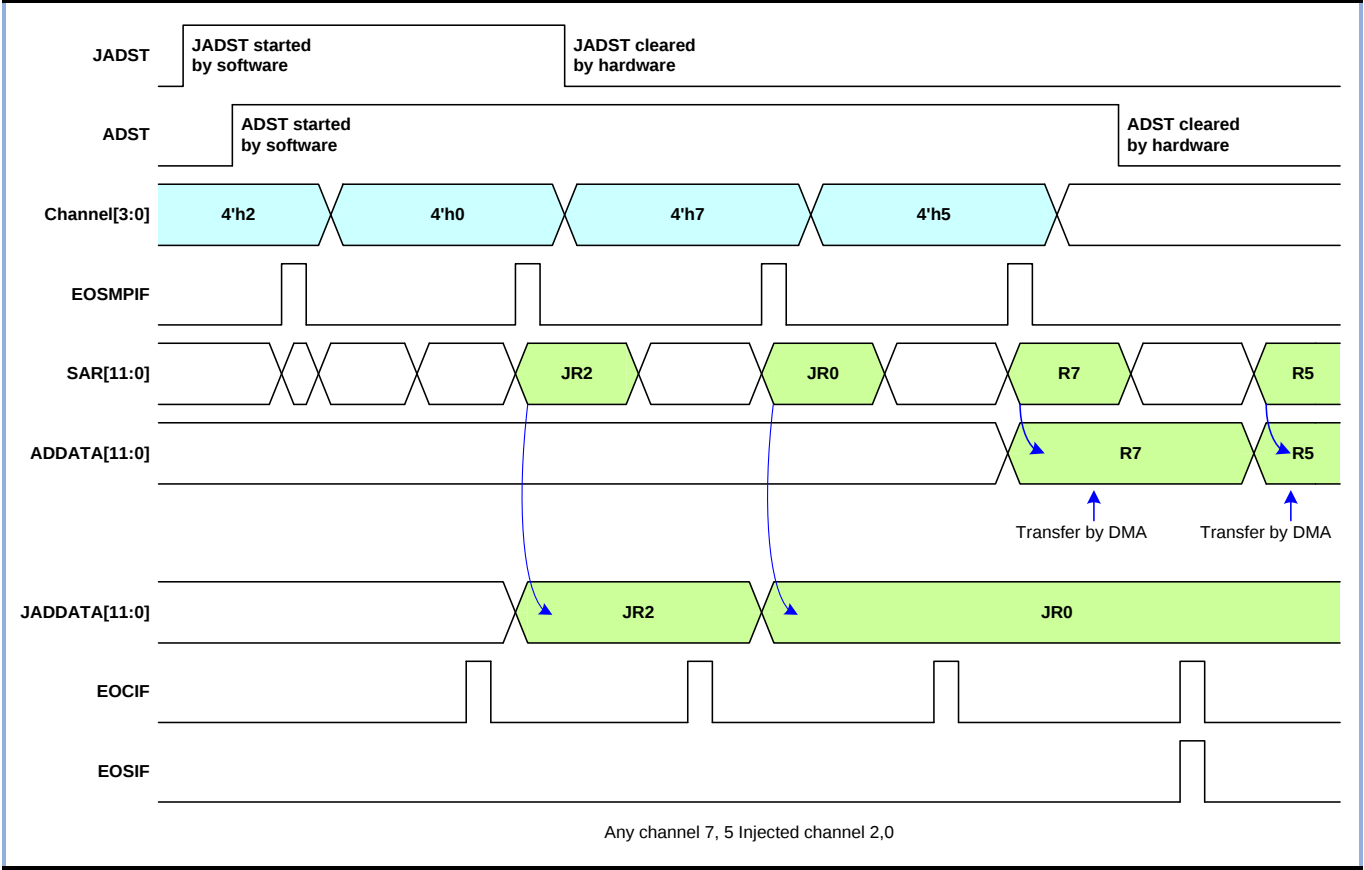
图 16-14 任意通道转换时事件注入通道转换时序图 1
