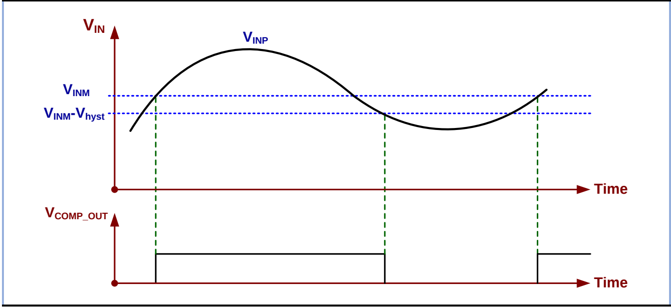
图 17-2 比较器迟滞
