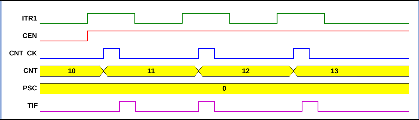
图 10-3 外部时钟模式 1 控制电路
