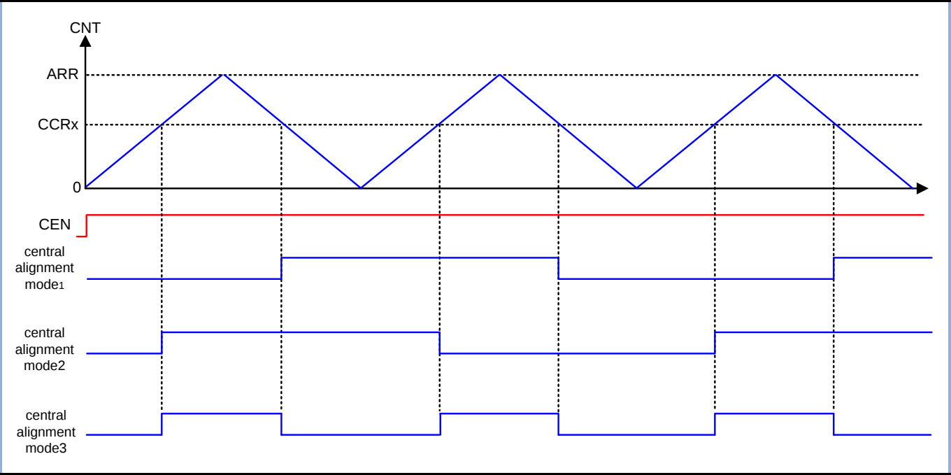
图 11-20 中央对齐模式下 CCx_SETTRGO 输出示例
