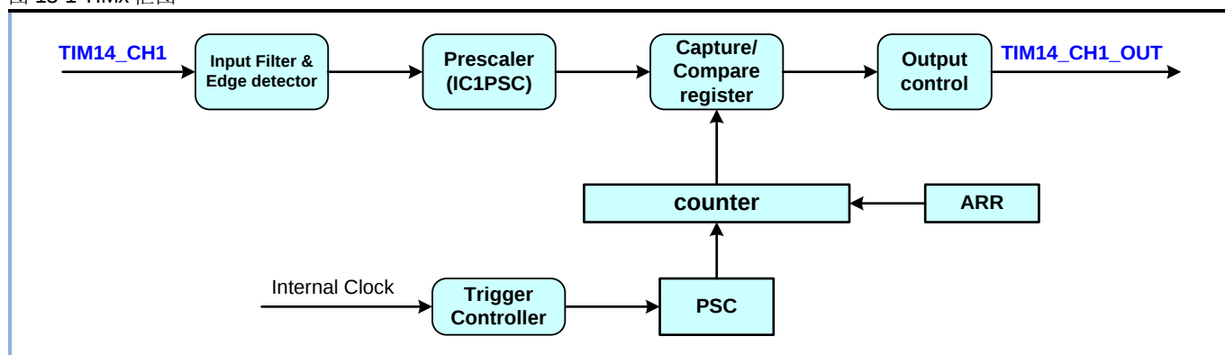
图 13-1 TIMx 框图
