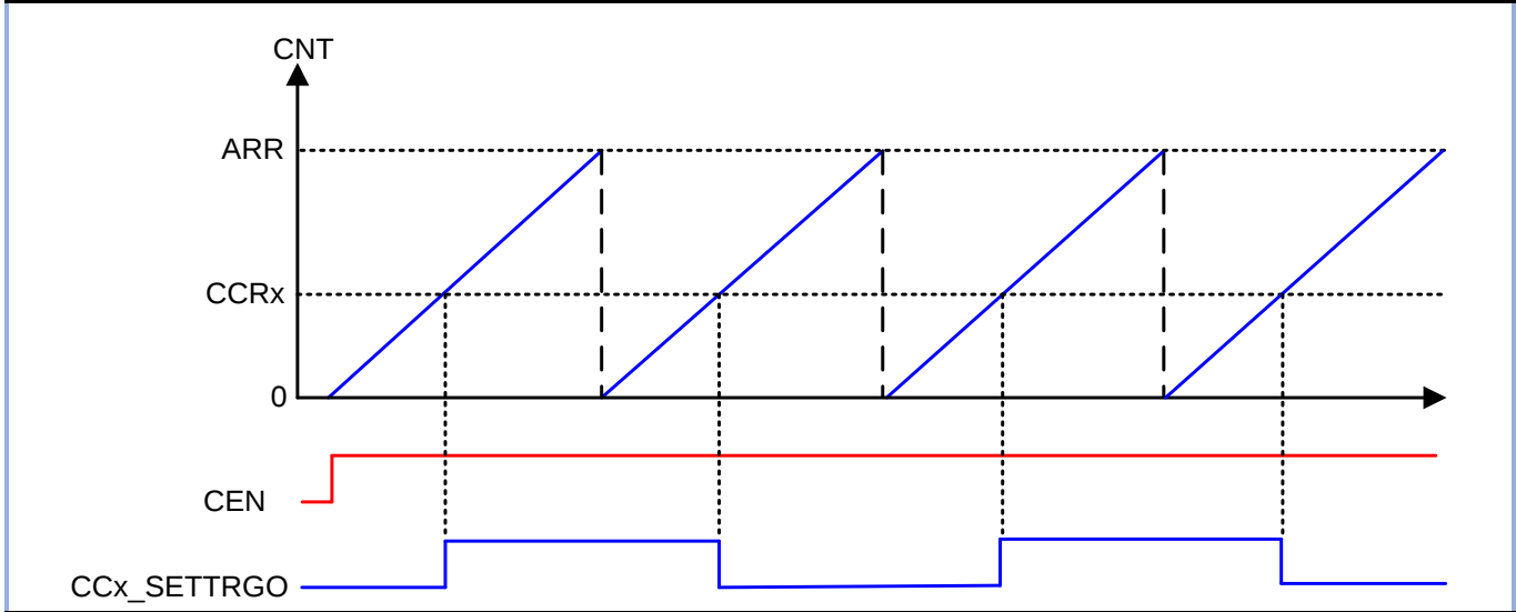
图 10-22 边沿对齐递增计数模式下 CCx_SETTRGO 输出示例
