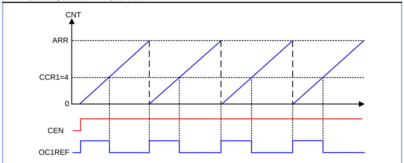
图 13-8 边沿对齐递增计数时 PWM 模式 1 的波形
