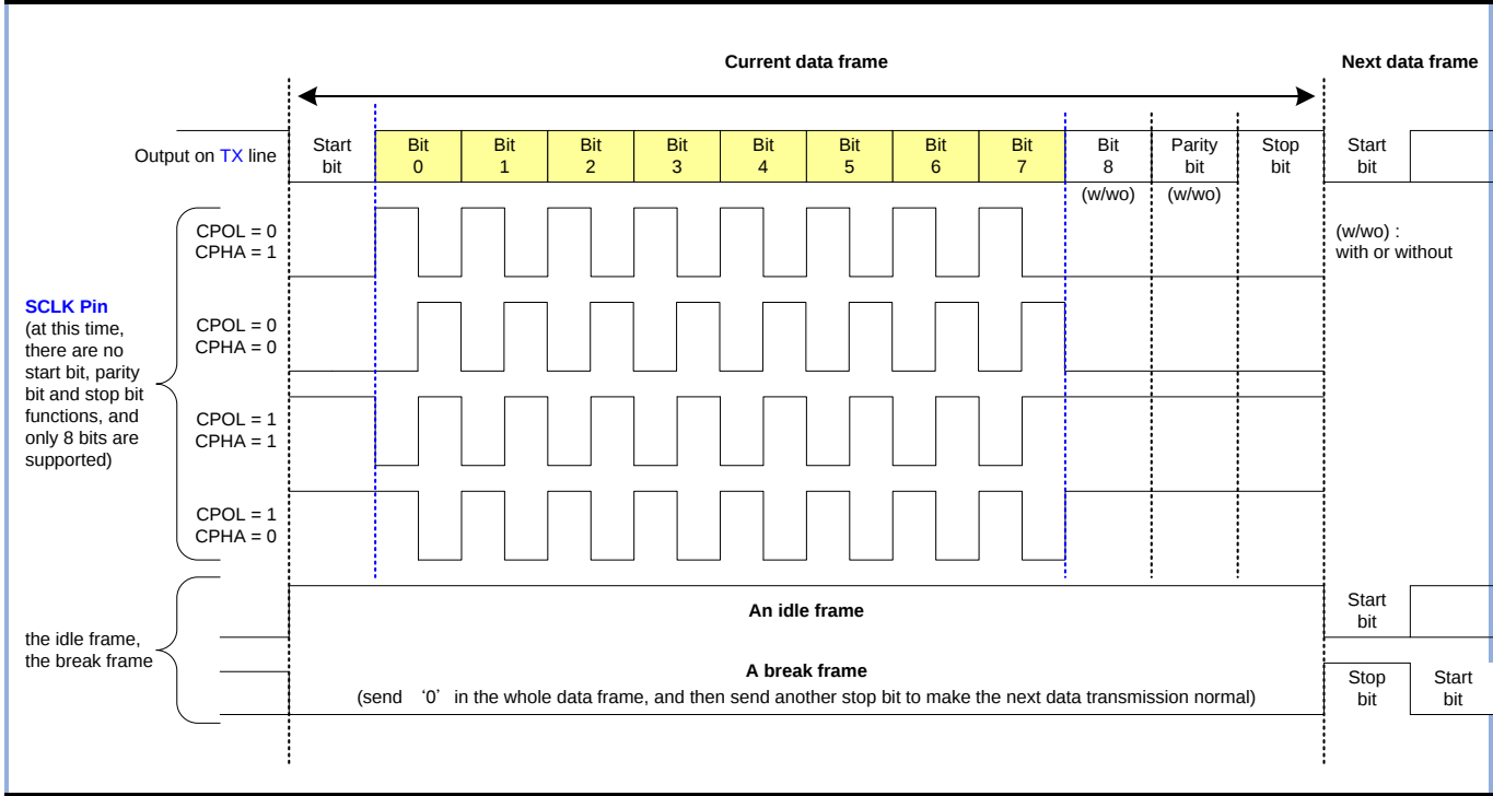
图 15-2 UART 数据帧类型示意图
