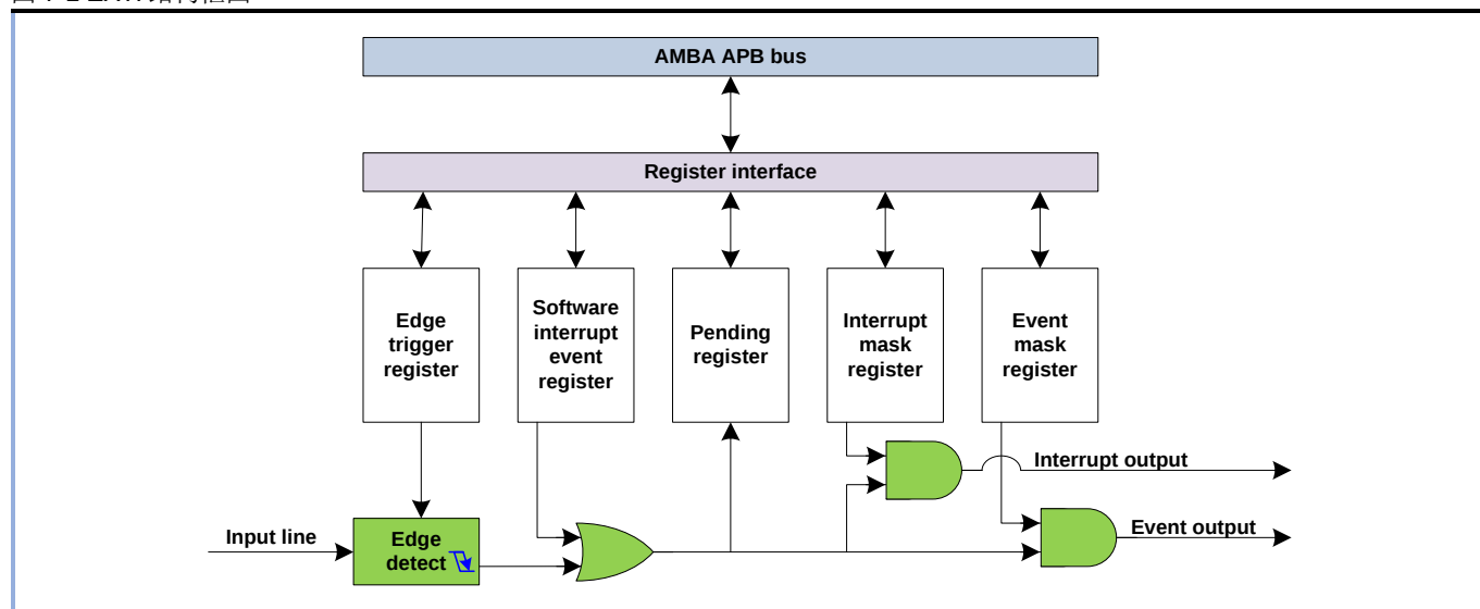
图 7-1 EXTI 结构框图
