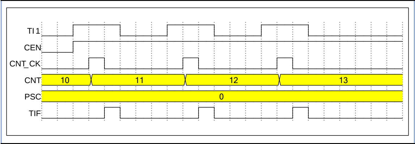
图 11-3 外部时钟模式 1 下的控制电路
