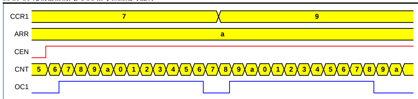
图 10-16 比较输出模式, OC1 信号在匹配时翻转
