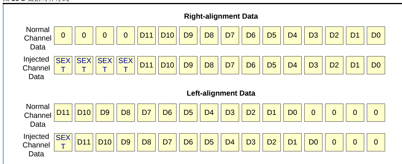
图 16-2 数据对齐方式
