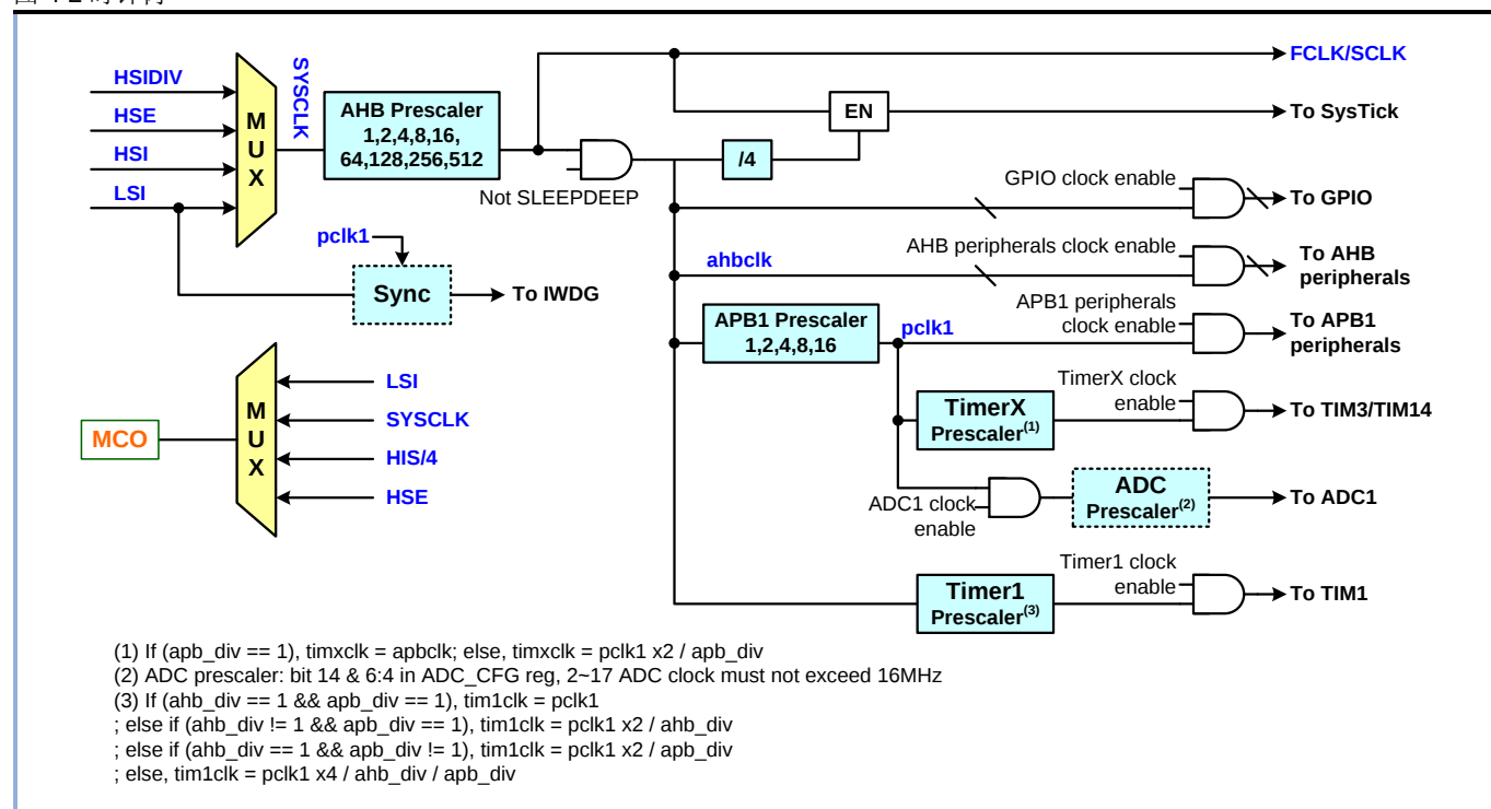
图 4-2 时钟树
