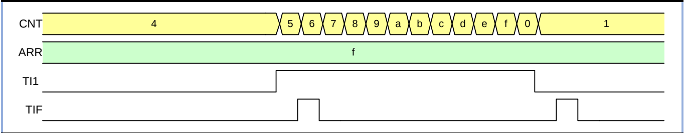
图 11-26 门控模式下的控制时序图
