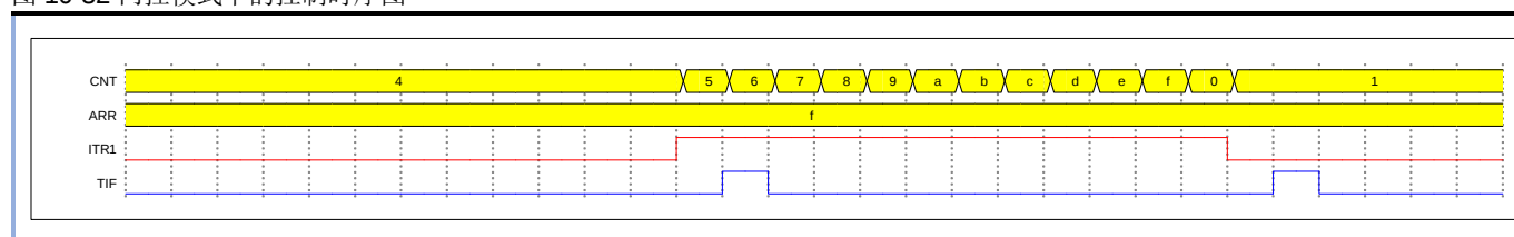
图 10-32 门控模式下的控制时序图
