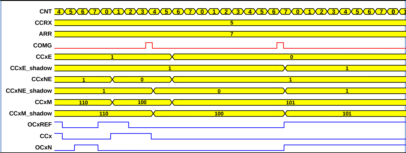
图 10-21 带 COM(OSSR = 1)的六步 PWM 示例
