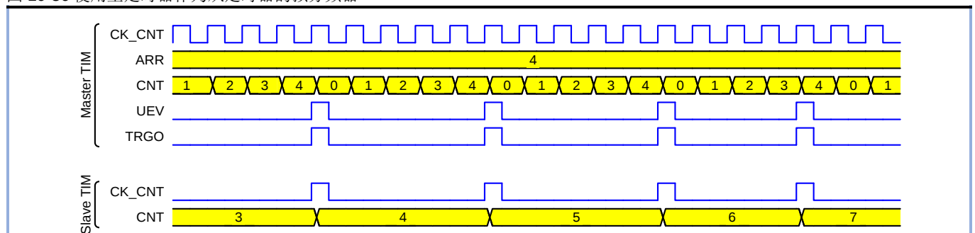
图 10-36 使用主定时器作为从定时器的预分频器
