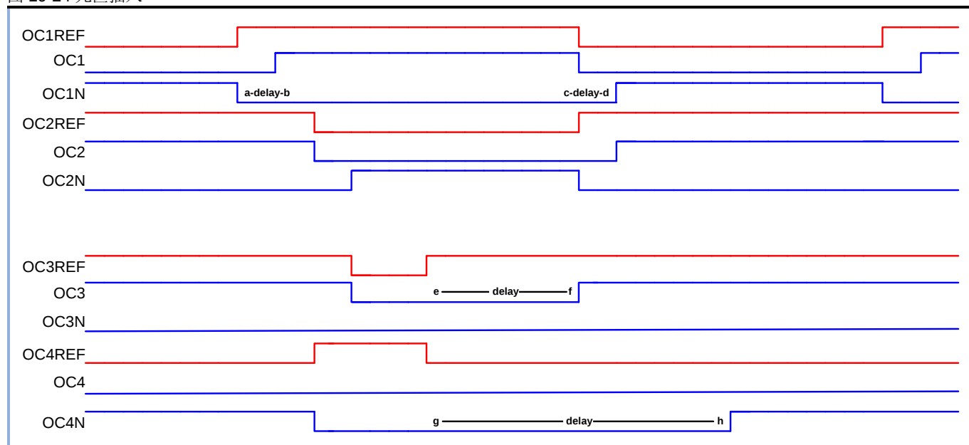
图 10-24 死区插入
