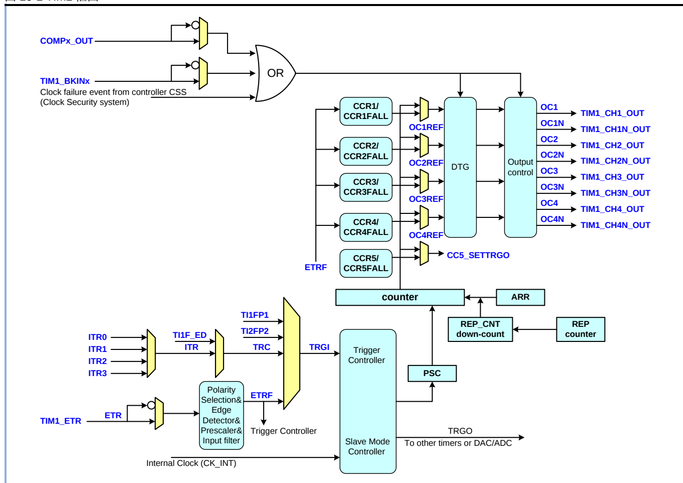
图 10-1 TIM1 框图
