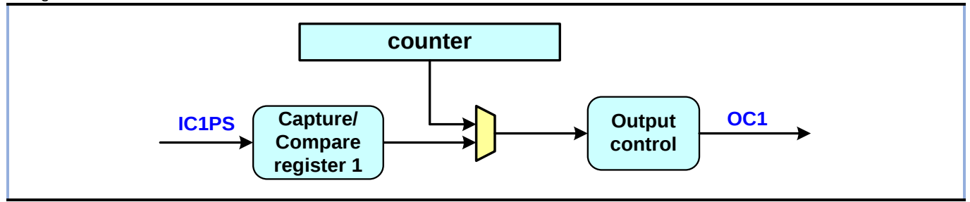
图 Figure 13-6 比较输出框图
