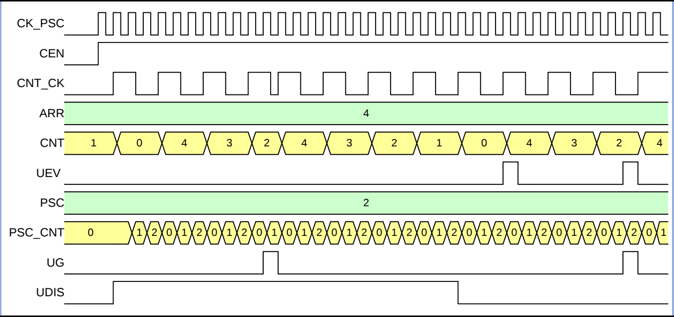
图 11-9 递减计数模式 (UDIS=1 禁止更新事件)
