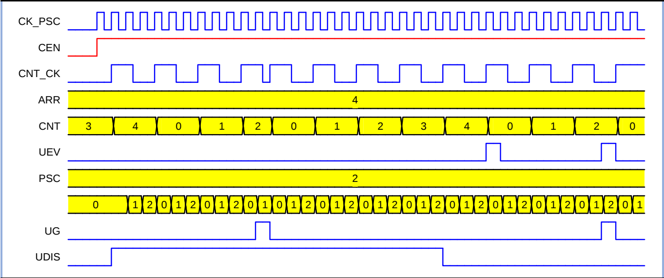
图 12-4 递增计数模式(UDIS=1 禁止产生更新事件)
