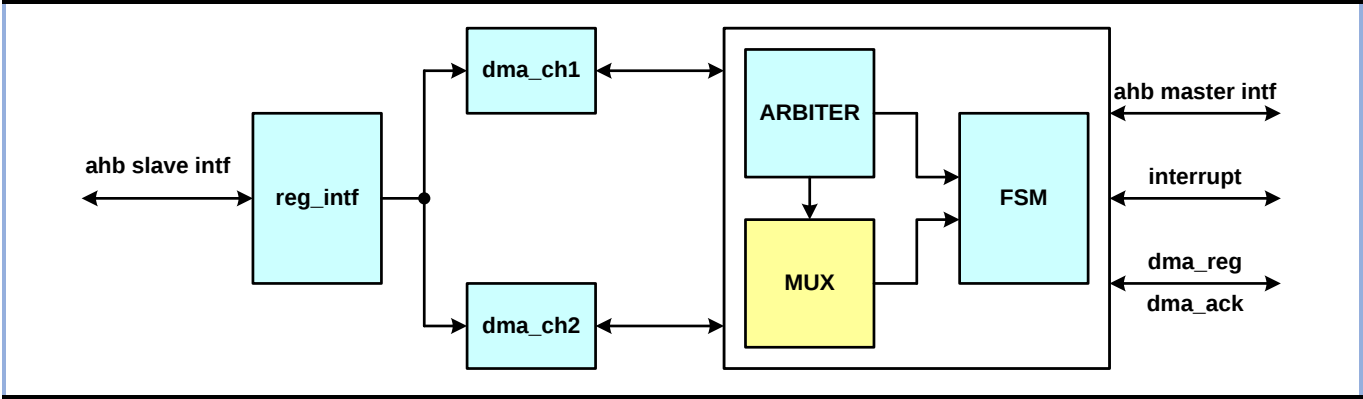
图 8-1 DMA 功能框图
