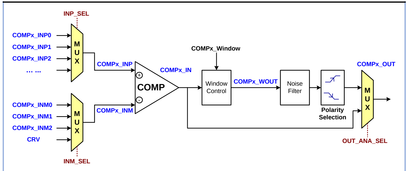
图 17-1 比较器框图
