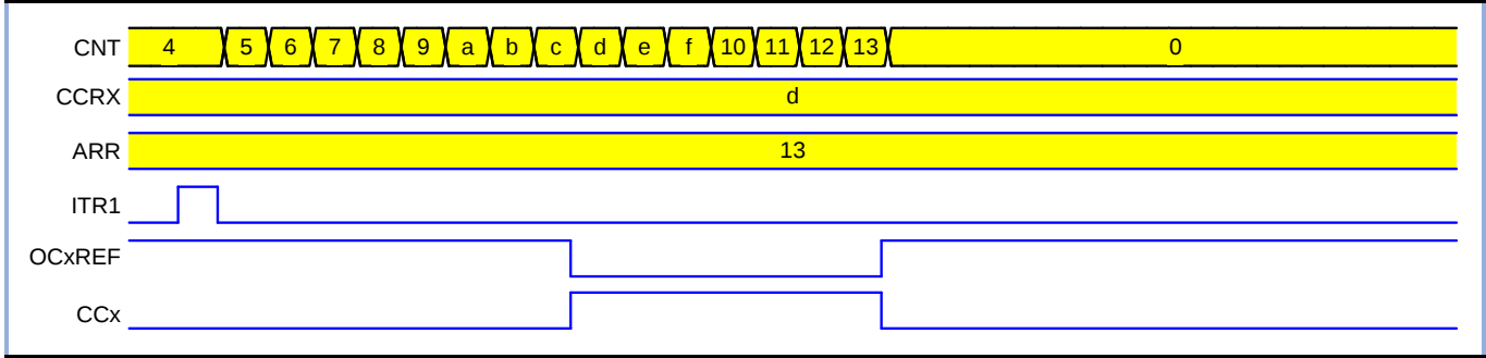
图 13-9 单脉冲模式
