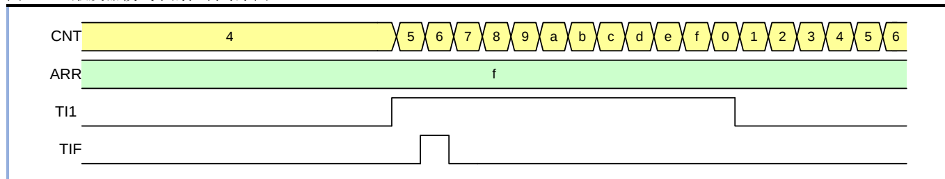
图 11-27 触发器模式下的控制时序图
