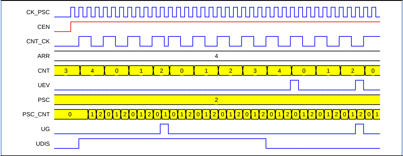
图 13-4 递增模式(UDIS =1,禁止更新事件)
