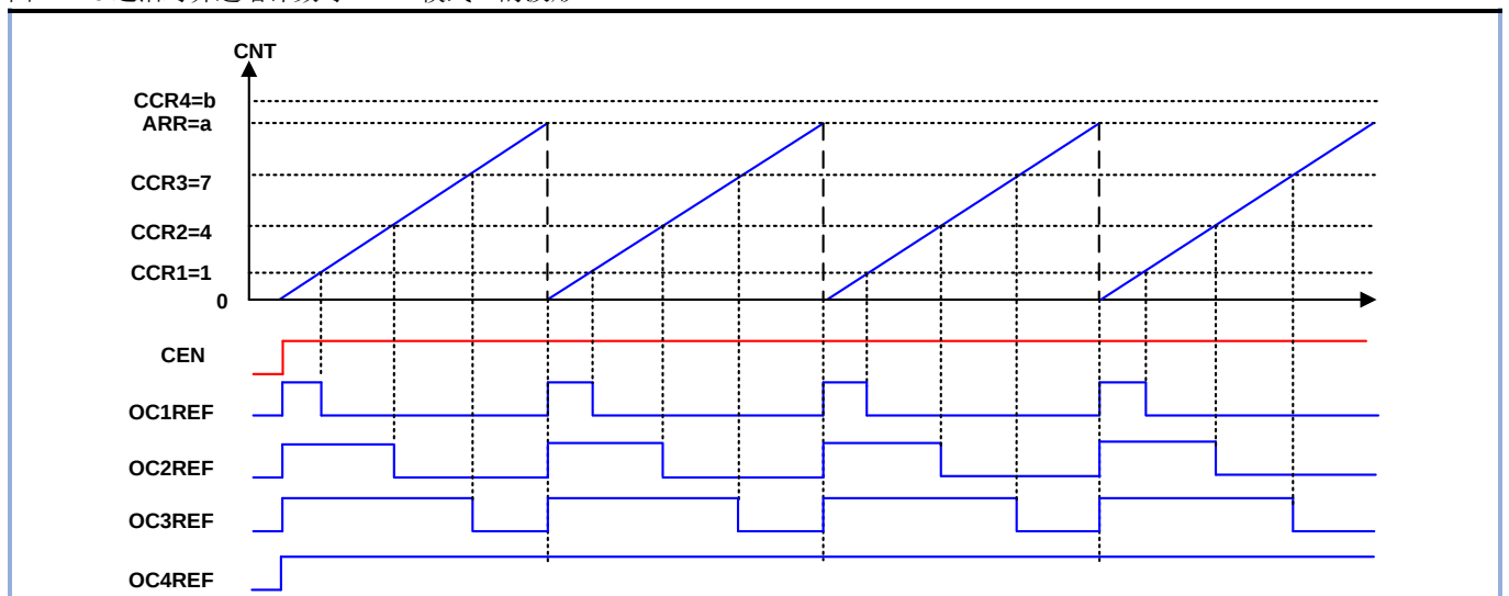
图 11-16 边沿对齐递增计数时 PWM 模式 1 的波形
