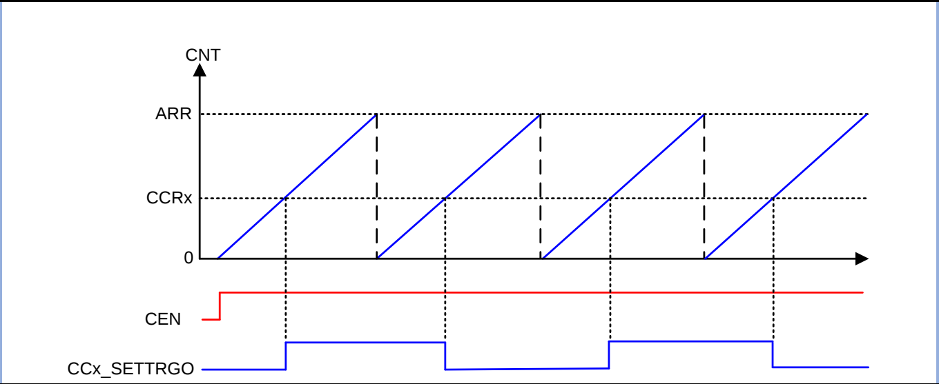
图 11-19 边沿对齐递增计数模式下 CCx_SETTRGO 输出示例
