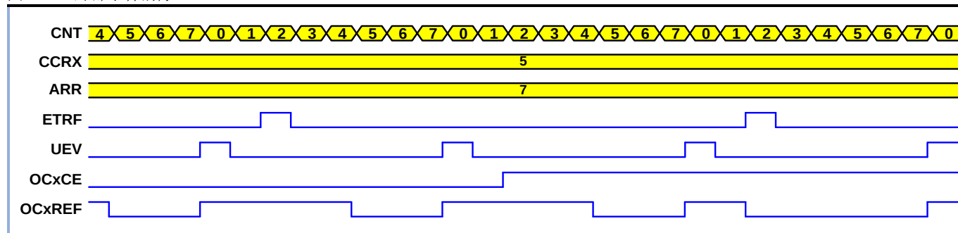
图 10-29 外部事件清除 OCxREF
