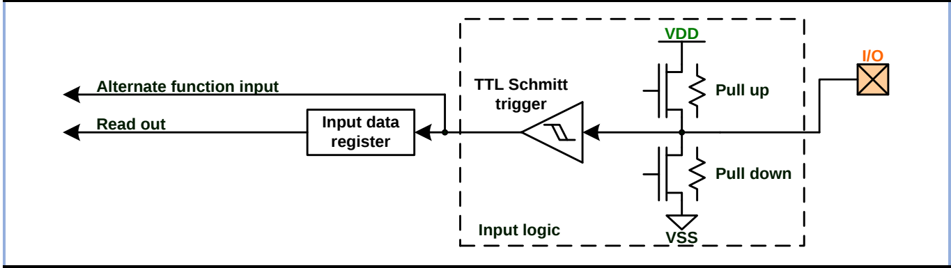
图 9-2 输入浮空/上拉/下拉配置
