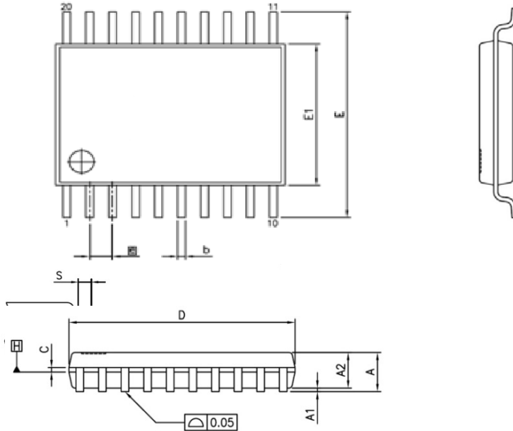
图 35-2. TSSOP-20 6.5 x 4.4mm, 0.65mm 封装尺寸
