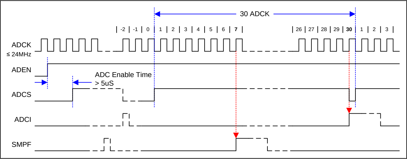
图 26–3. ADC 转换时序
