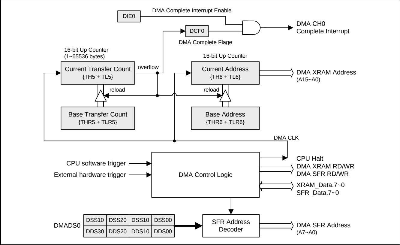
图 8-2. DMA 结构
