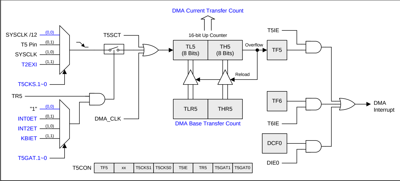
图 8-4.定时器 5 结构
