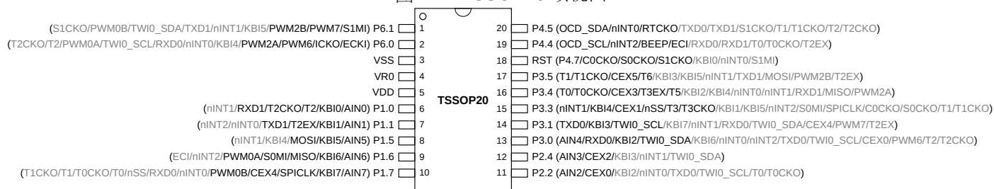
图 4-2. TSSOP20 顶视图
