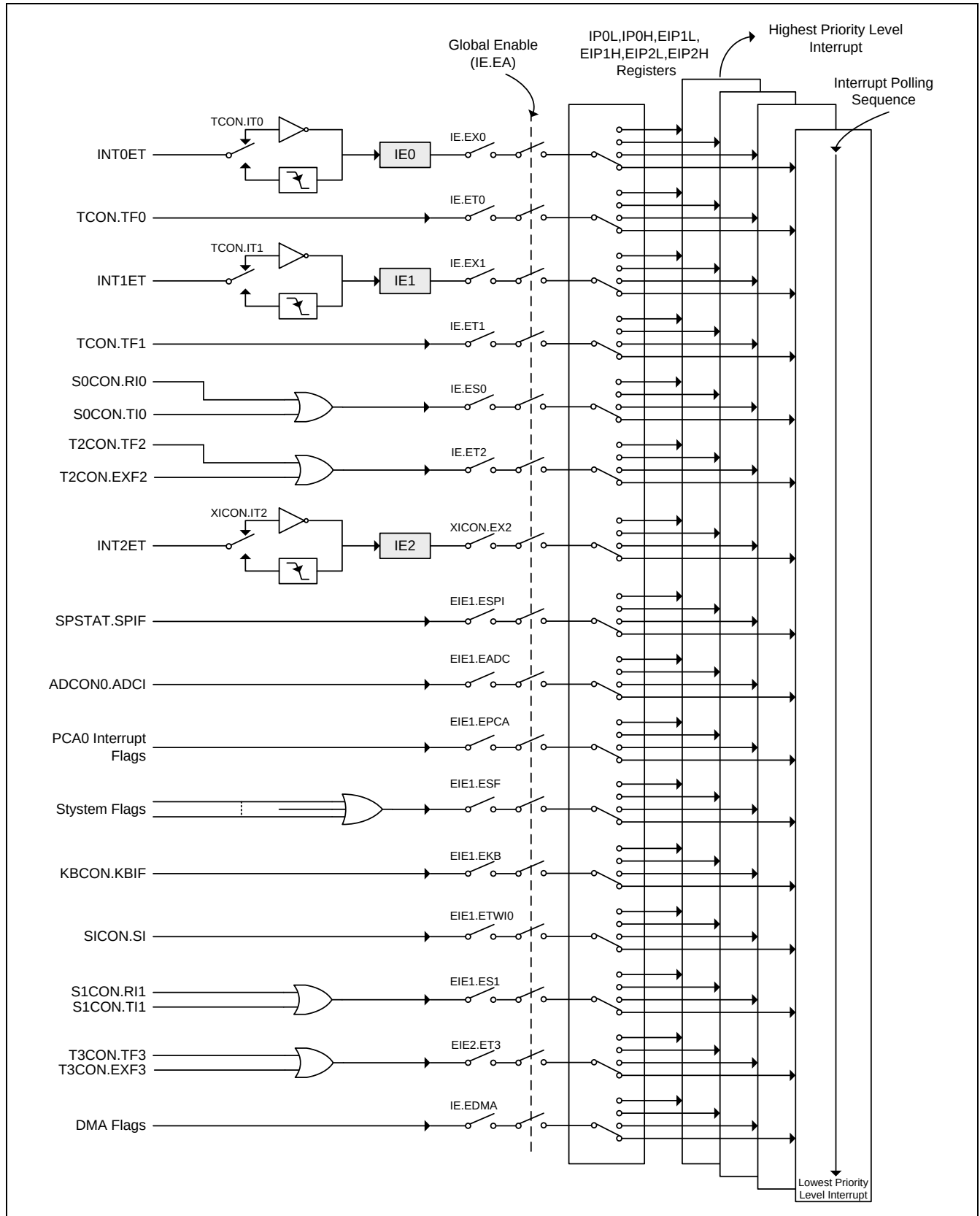
图 15-1.中断系统
