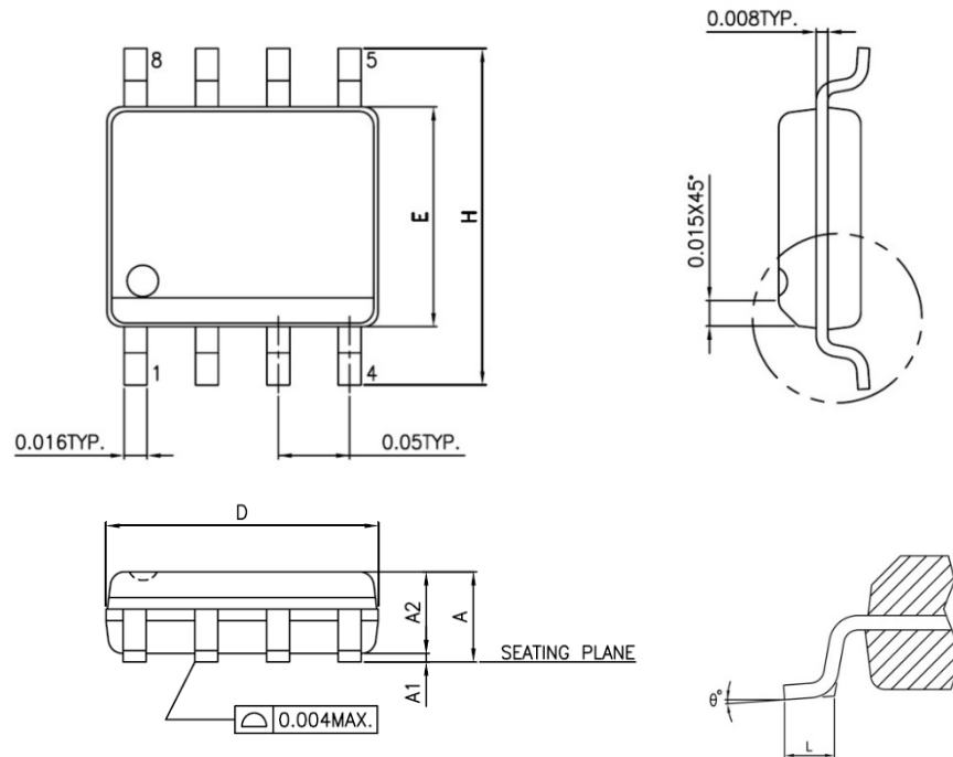
图 35-4. SOP-8 (150 mil) 封装尺寸
