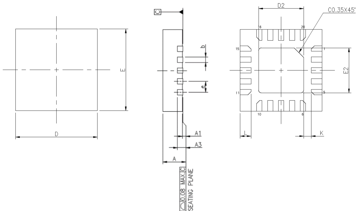
图 35-3. QFN-20 (3x3x0.75mm)封装尺寸
