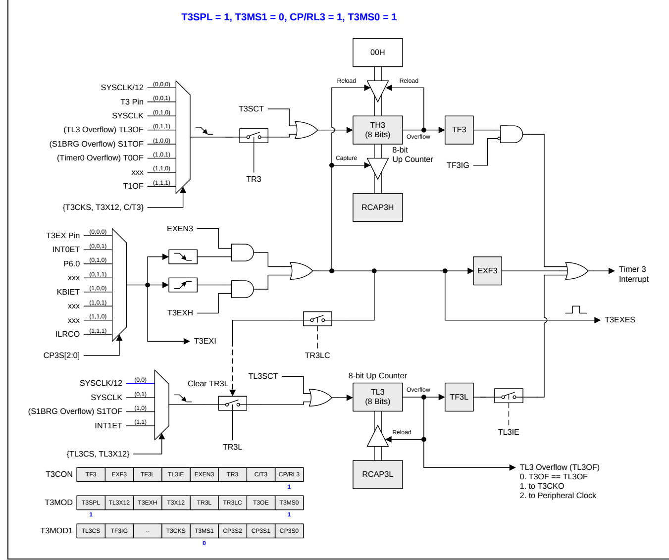
图 16-34.分立定时器 3 模式 3 结构(捕捉带自动清零 TH3)
