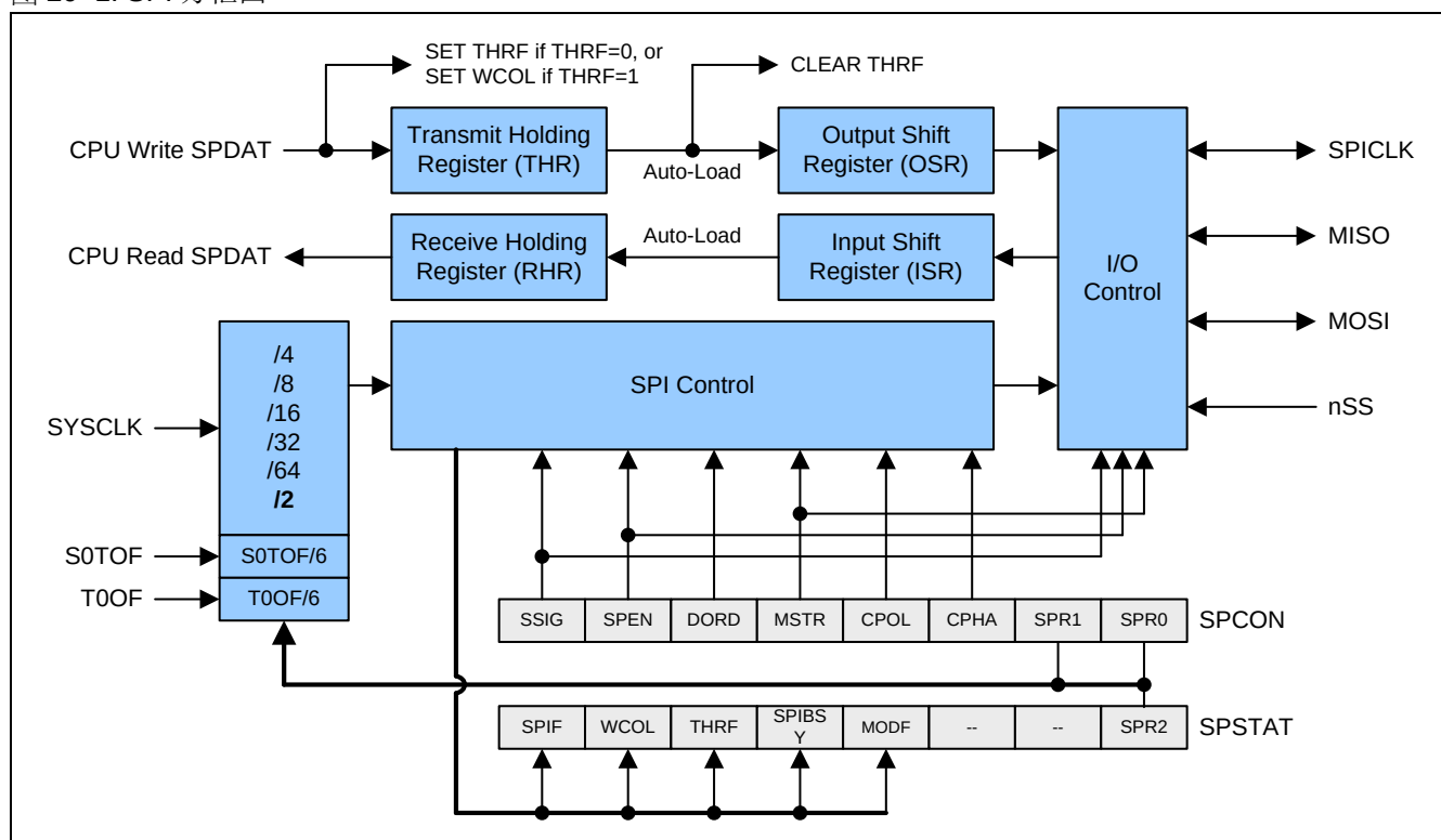
图 20-1. SPI 方框图
