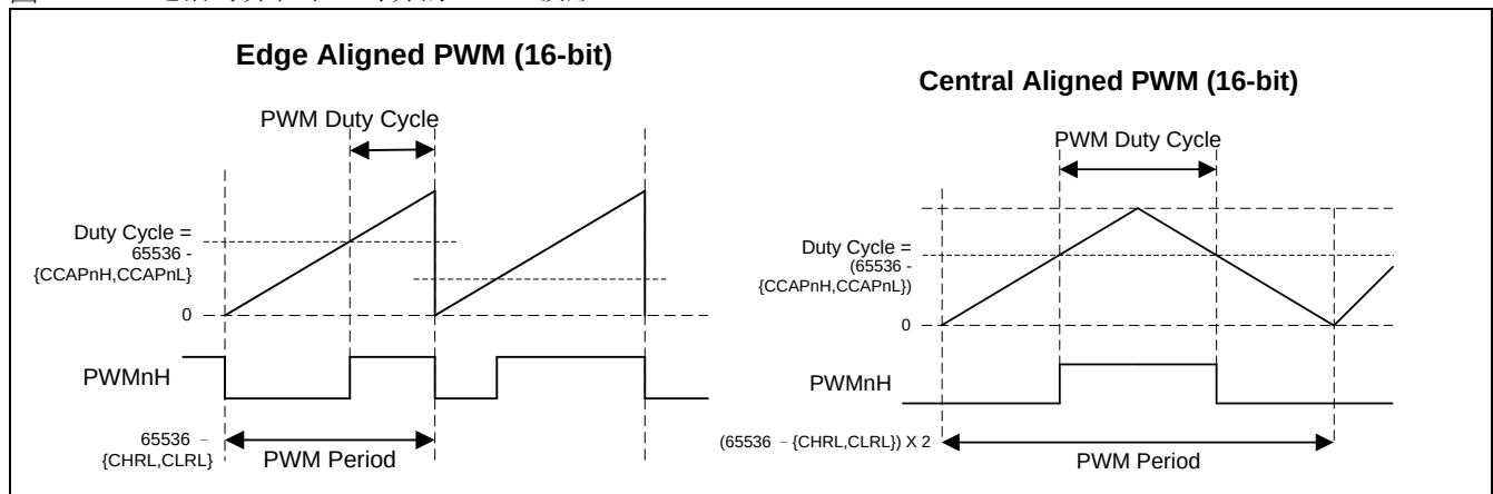
图 17-16. 边沿对齐和中心对齐的 PWM 波形
