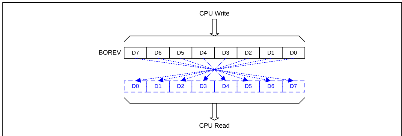
图 25-2. BOREV 结构
