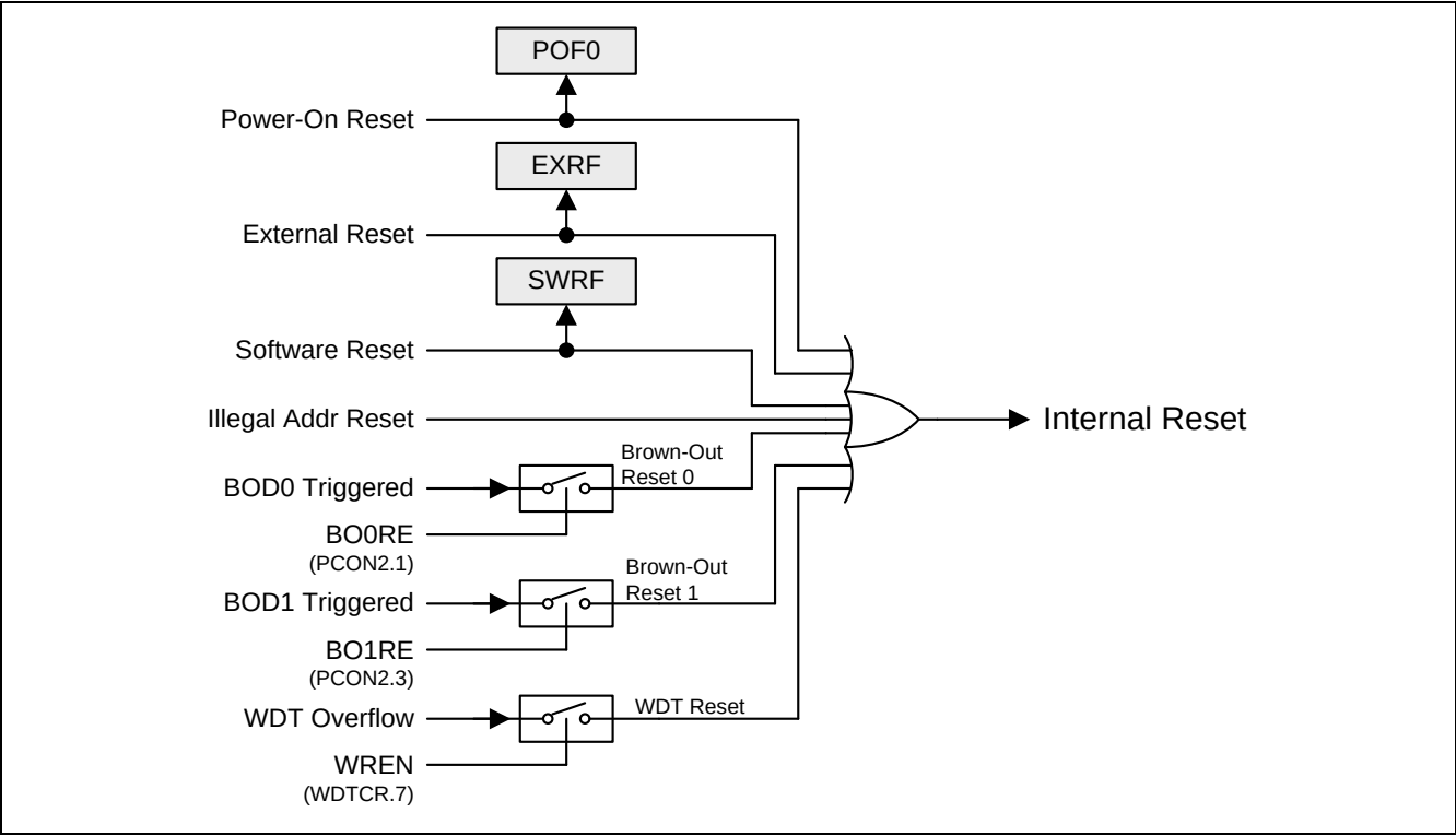
图 12-1.系统复位源
