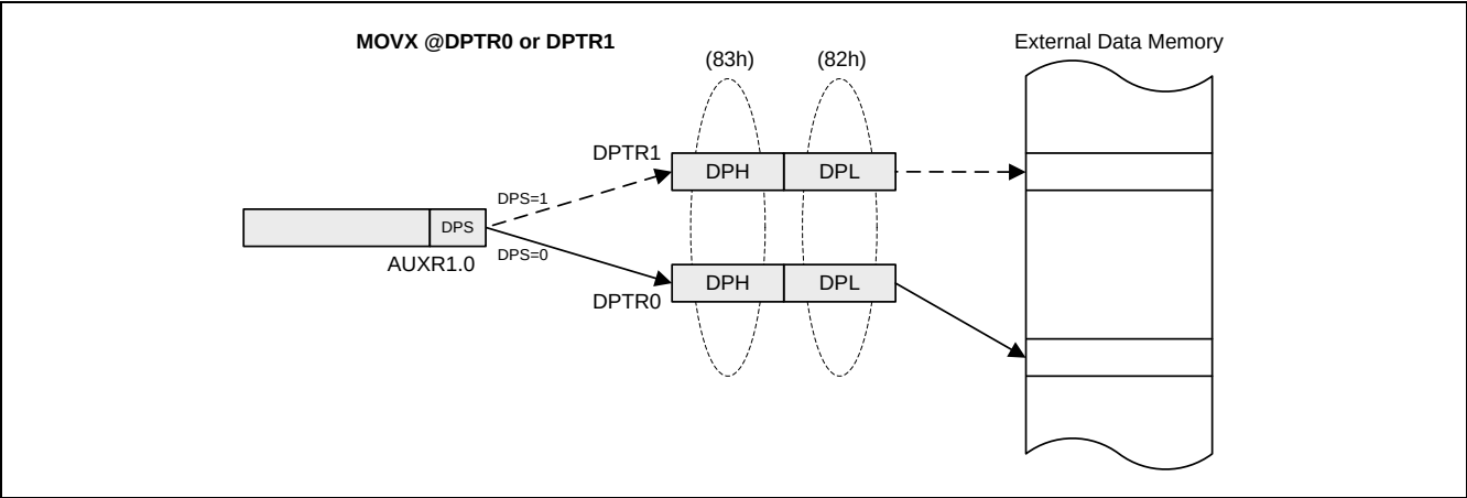
图 7-1. 双 DPTR 结构
