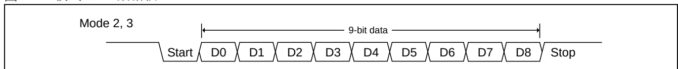
图 18-2.模式 2, 3 数据帧
