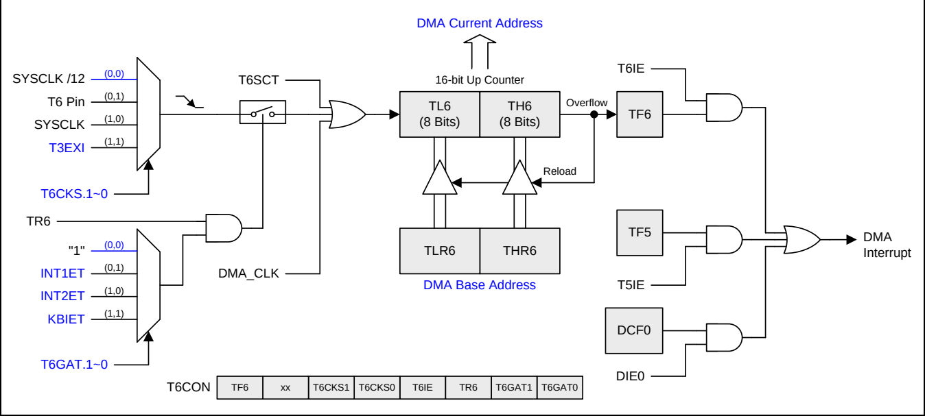
图 8-5.定时器 6 结构
