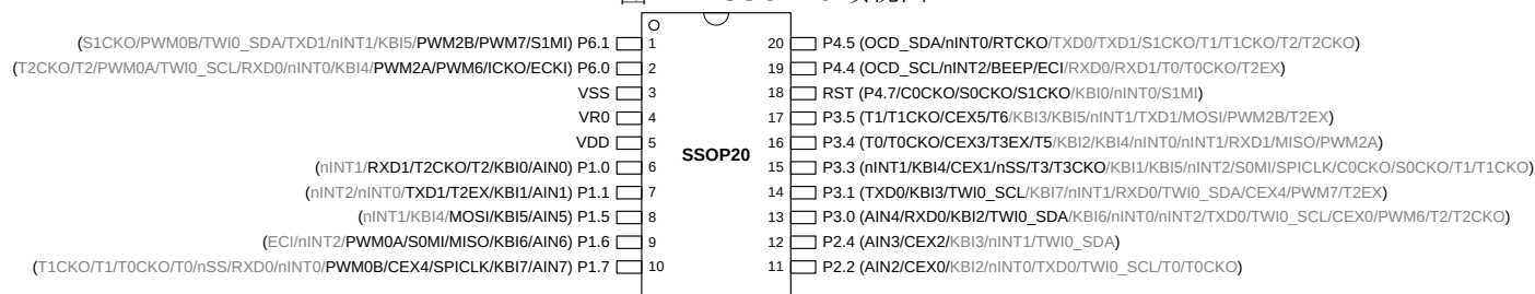
图 4-1. SSOP20 顶视图
