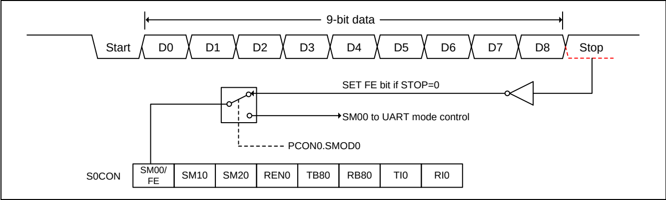
图 18-7.UART0 帧错误侦测
