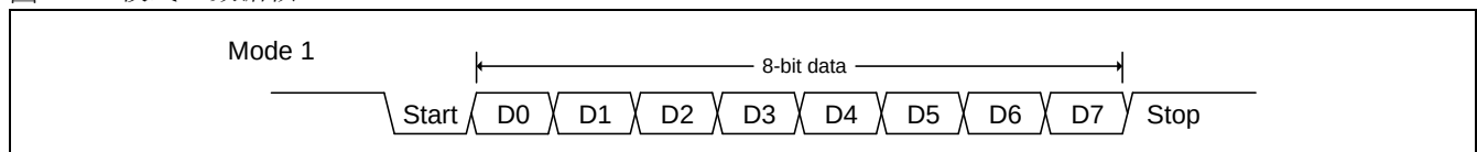
图 18-1.模式 1 数据帧
