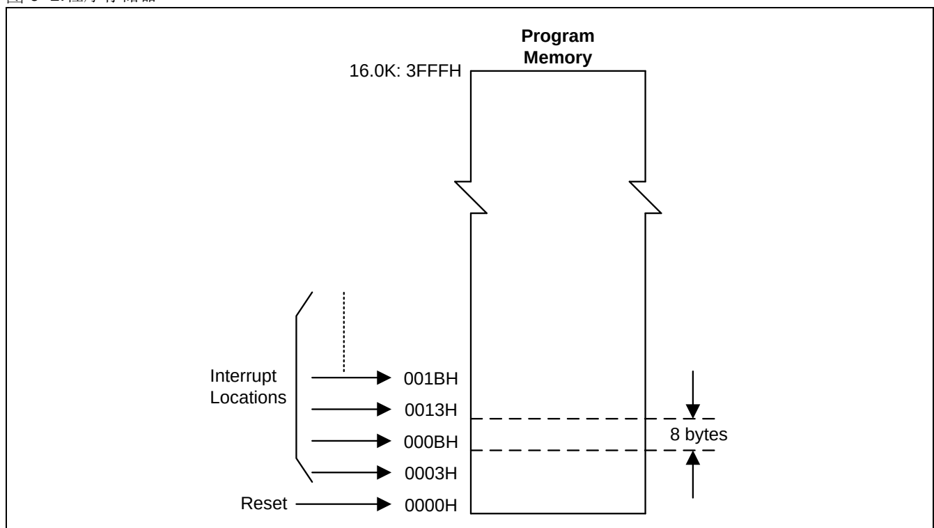
图 6-1. 程序存储器
