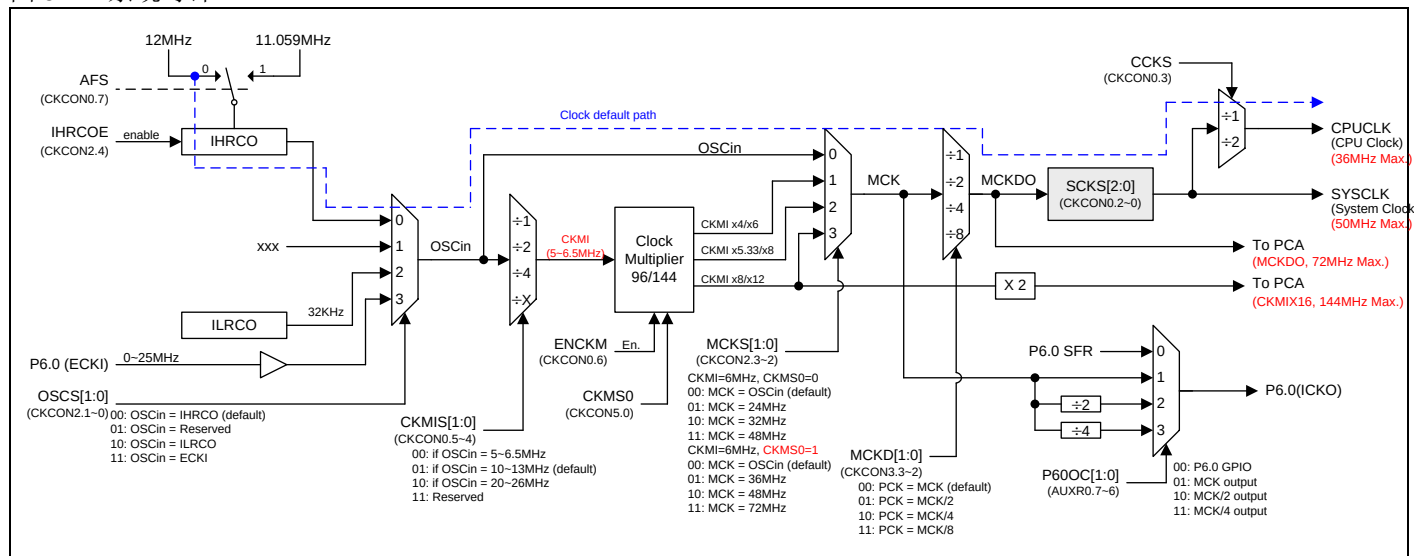
图 9-1. 系统时钟
