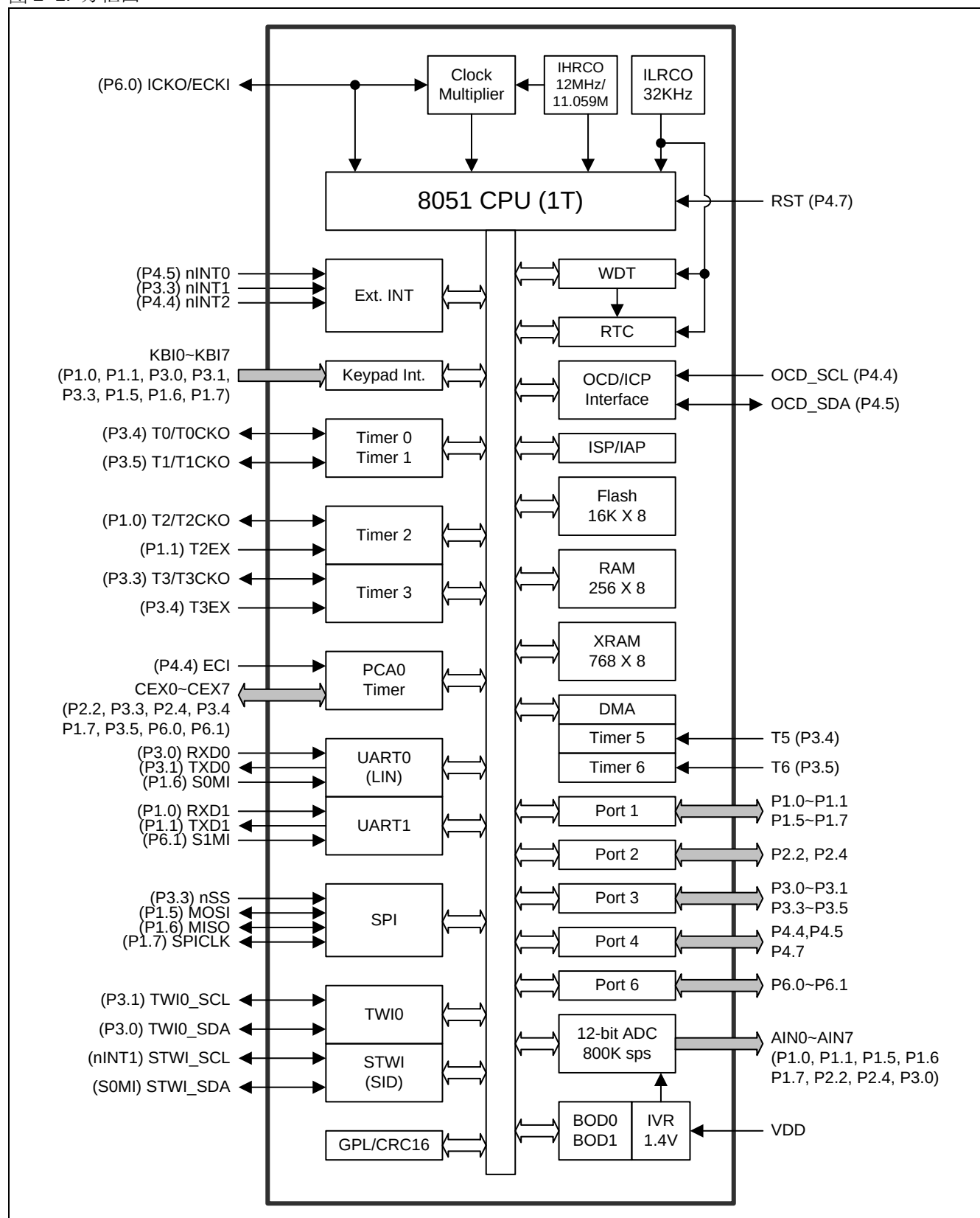
图 2-1. 方框图
