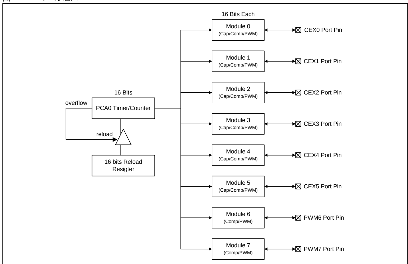
图 17-1. PCA 方框图
