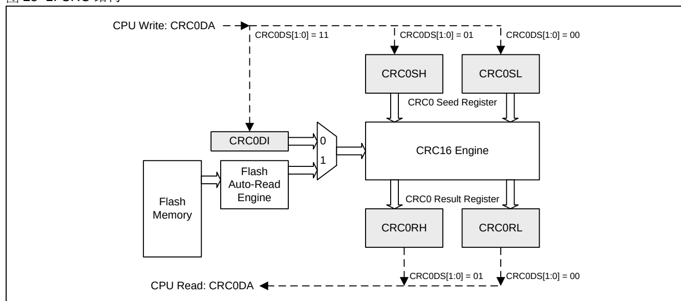
图 25-1. CRC 结构
