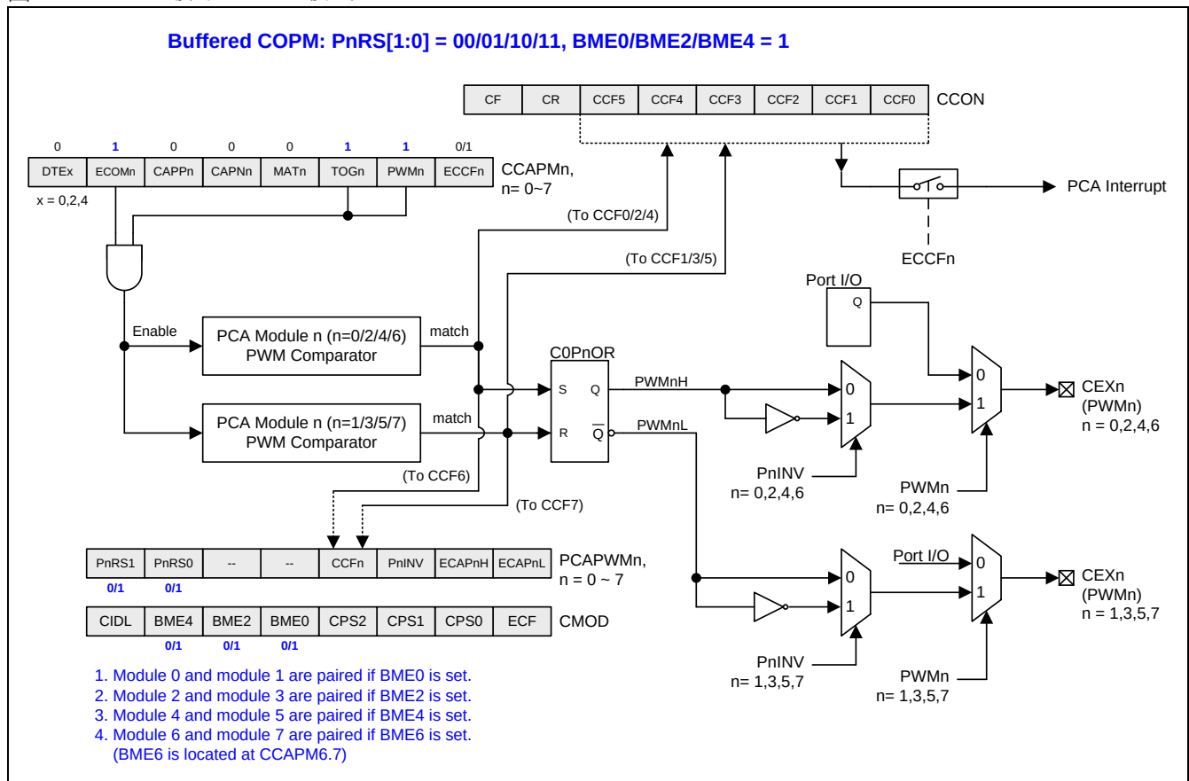
图 17-13. PCA 缓冲 COPM 模式
