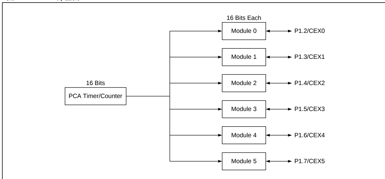
图 14-1. PCA 方框图
