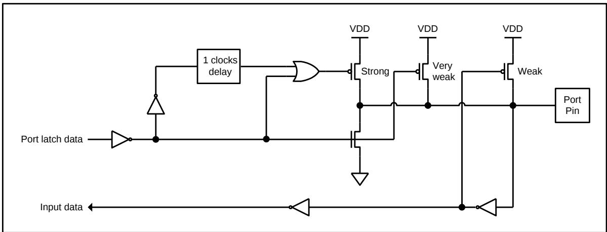
图 9-1 准双向 I/O
