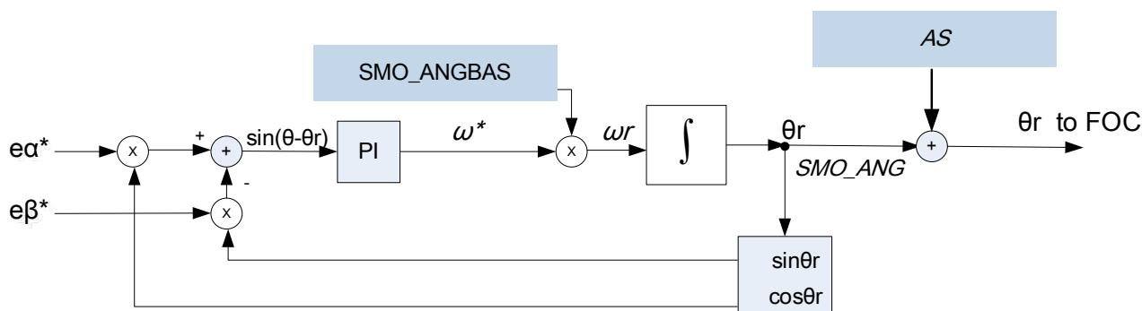
图 25.5.3 : PLL 架构
