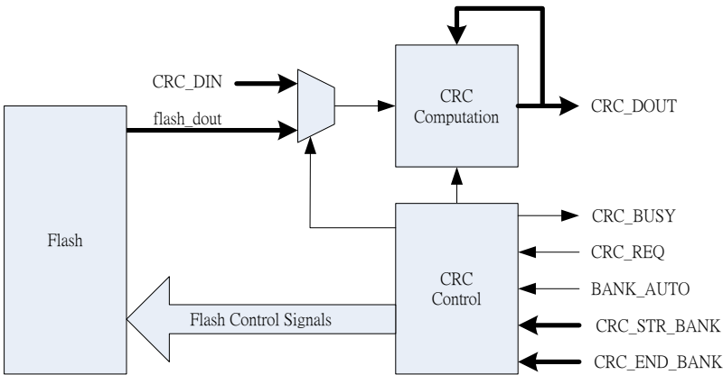
图 21.2 : 字节和 Flash 块 CRC 计算架构
