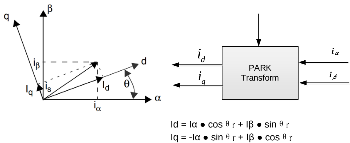
图 25.2.3 : Park 变换
