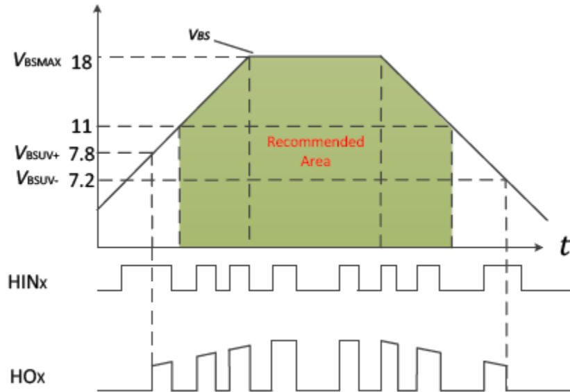
图 27.2.1 VBS 电源 UVLO 工作区域
