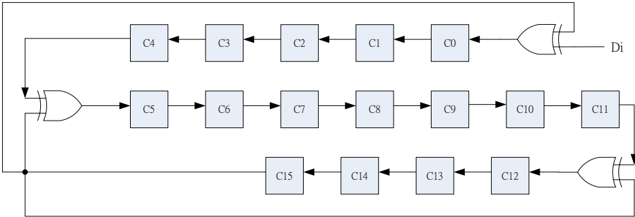
图 21.1 : CRC16-CCITT 的通用 LSFR 体系结构
