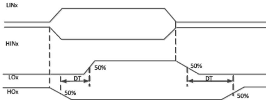
图 27.5.1 死区时间
