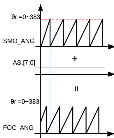
图 25.5.4 : 角度补偿
