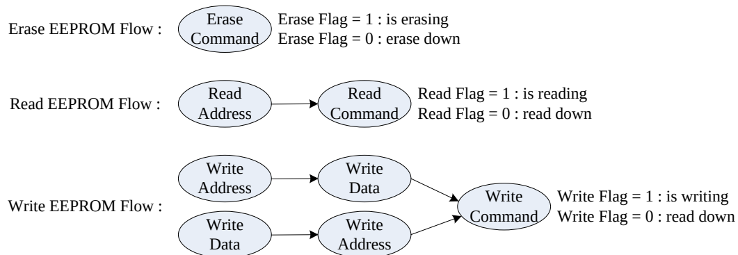
图 17.1 : EEPROM 擦除，读和写控制流程
