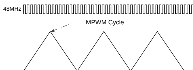
图 25.6.6：电机 PWM 向上向下定时器
