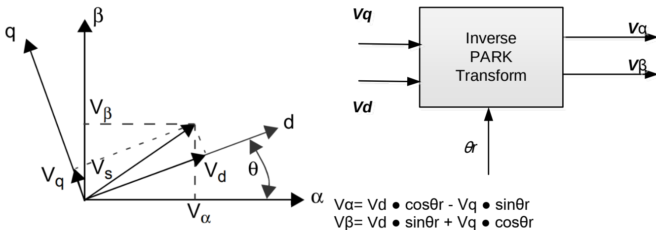
图 25.4.2：PARK 逆变换
