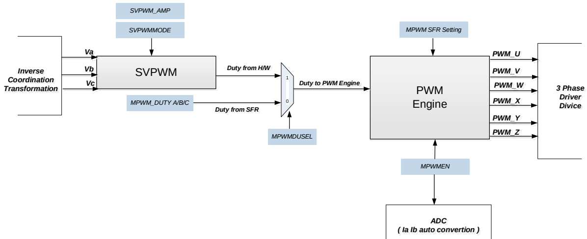
图 25.6.1 : SVPWM 引擎模块框图
