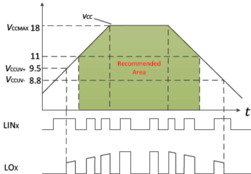
图 27.1.1. VCC15 电源 UVLO 工作区域
