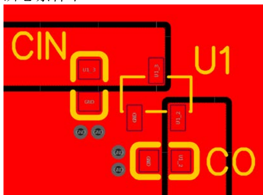
SOT233 PCB
