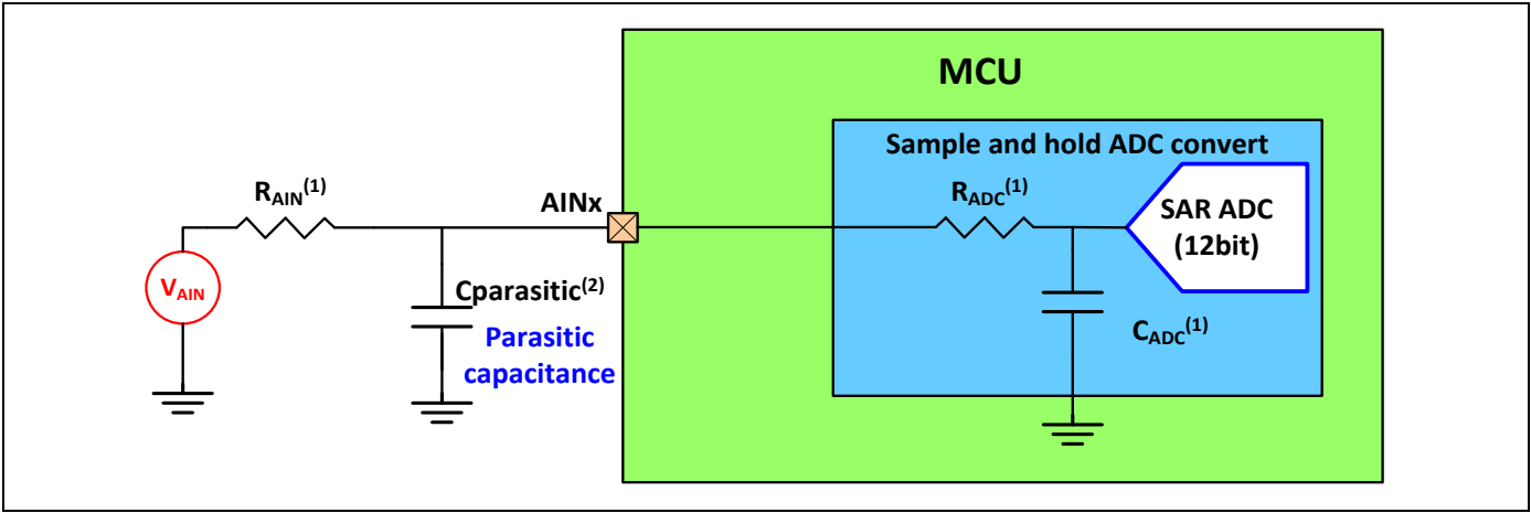
图 14 使用 ADC 的典型连接图
