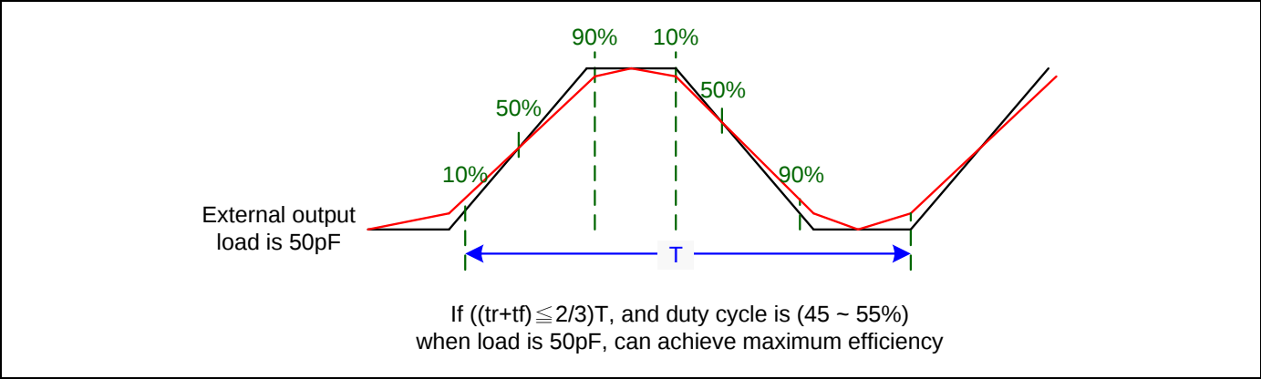
图 11 输入和输出交流特性定义
