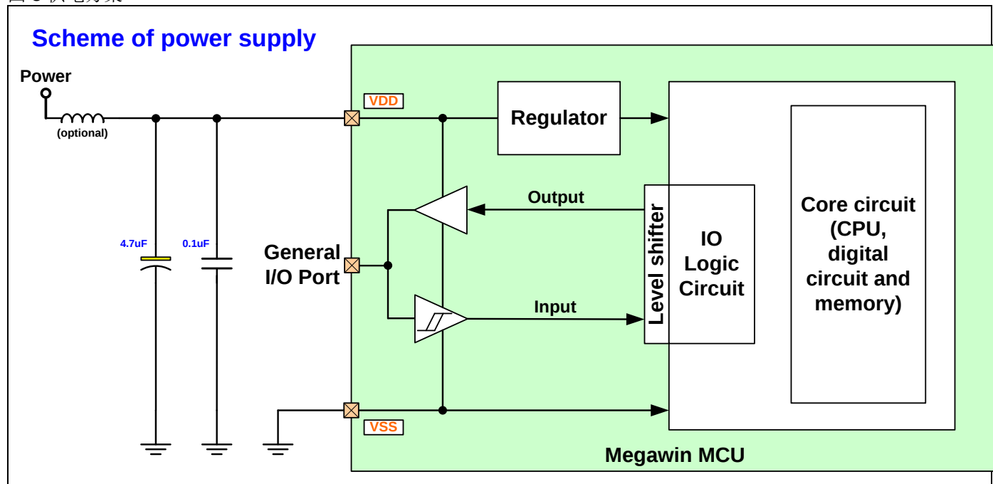
图 8 供电方案
