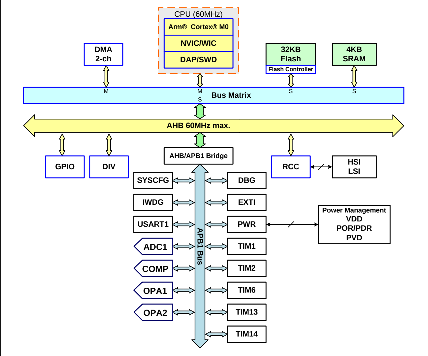
图 1 方框图
