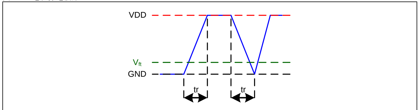
图 10 上电和掉电波形
