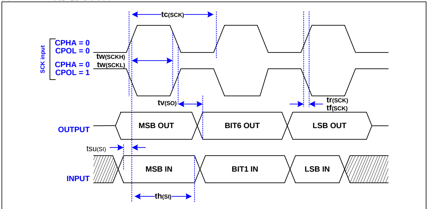
图 13 USART 同步模式时序图
