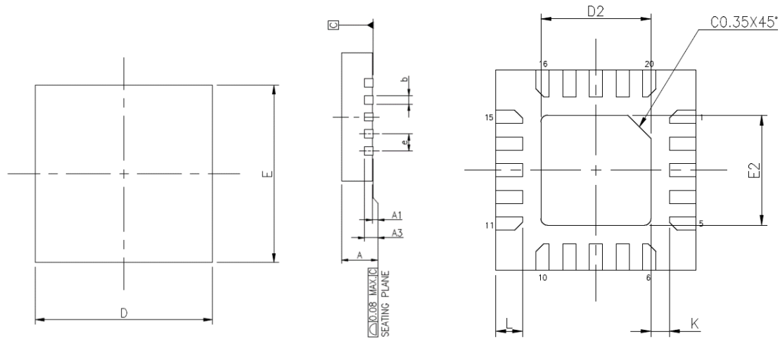
图 18 QFN-20 (3mm X 3mm X 0.75mm)
