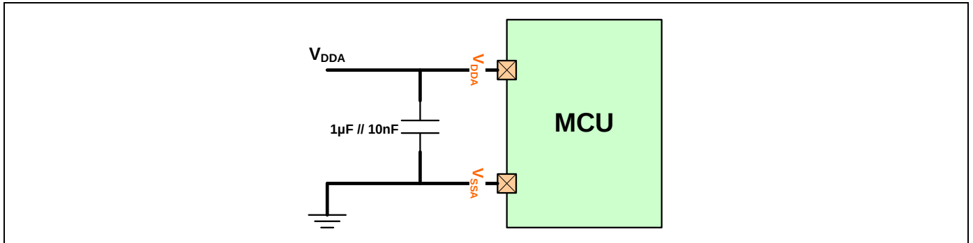
图 15 供电电源和参考电源去耦线路
