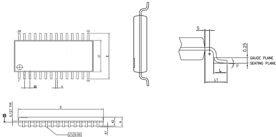
图 17 TSSOP28 (173mil) (9.7x4.4x1.0)
