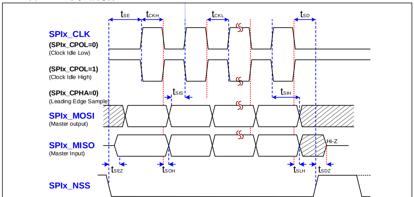
图 8-3. SPI 从机时序波形
