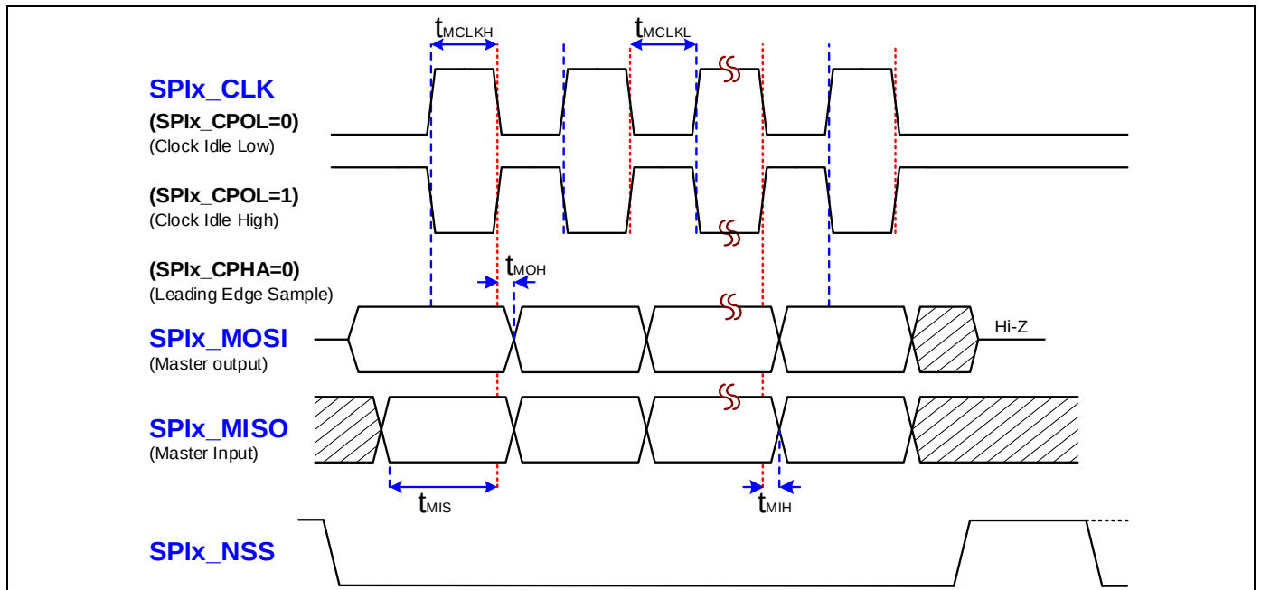
图 8-2. SPI 主机时序波形
