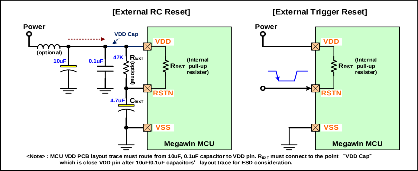
图 7-2. 复位电路
