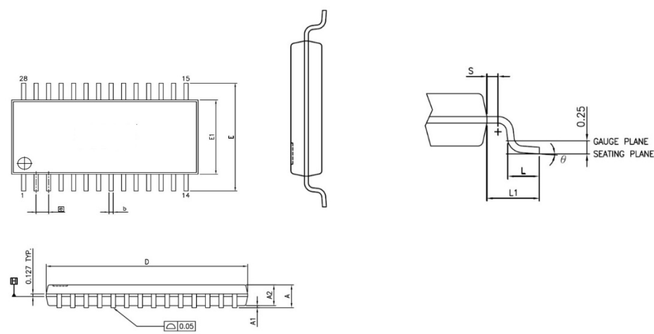
图 15 TSSOP28, 28 脚低剖面方形扁平封装图
