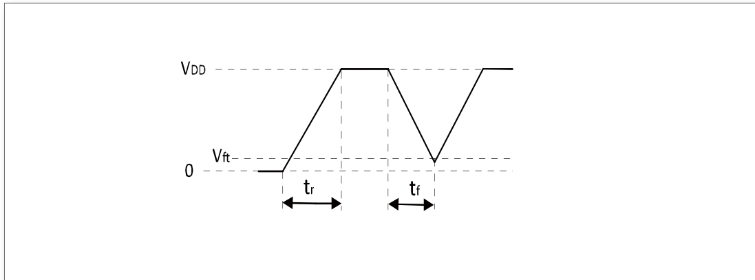
图 9 上电与掉电波形
