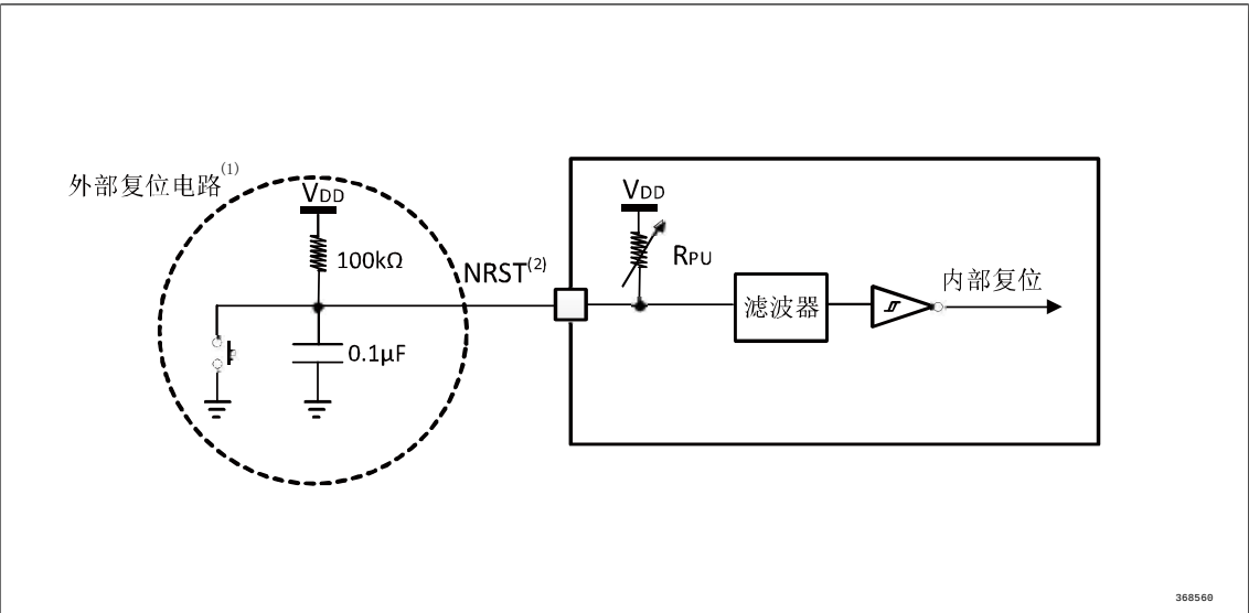
图 11 建议的 NRST 引脚保护
