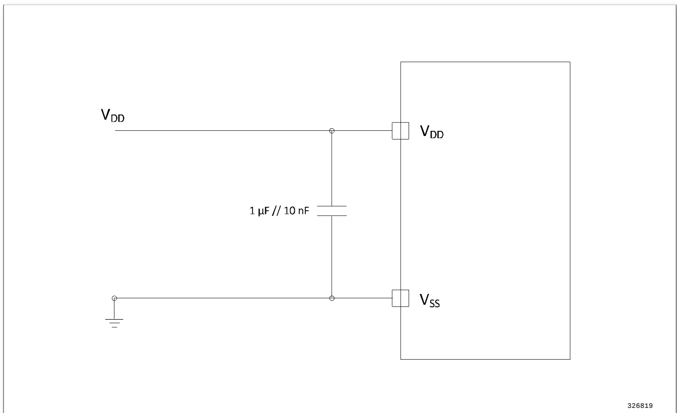
图 14 供电电源和参考电源去耦线路
