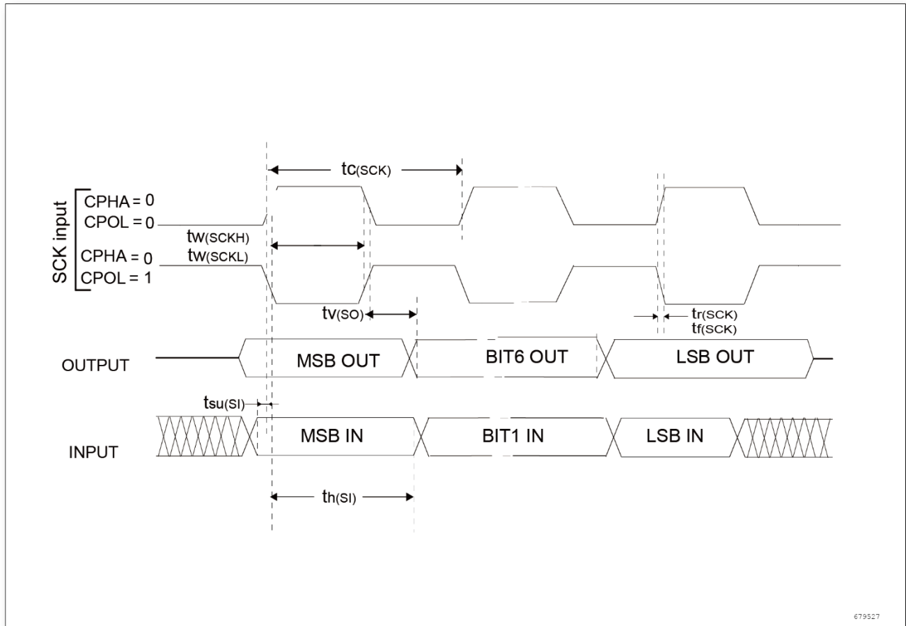
图 12 USART 同步模式时序图
