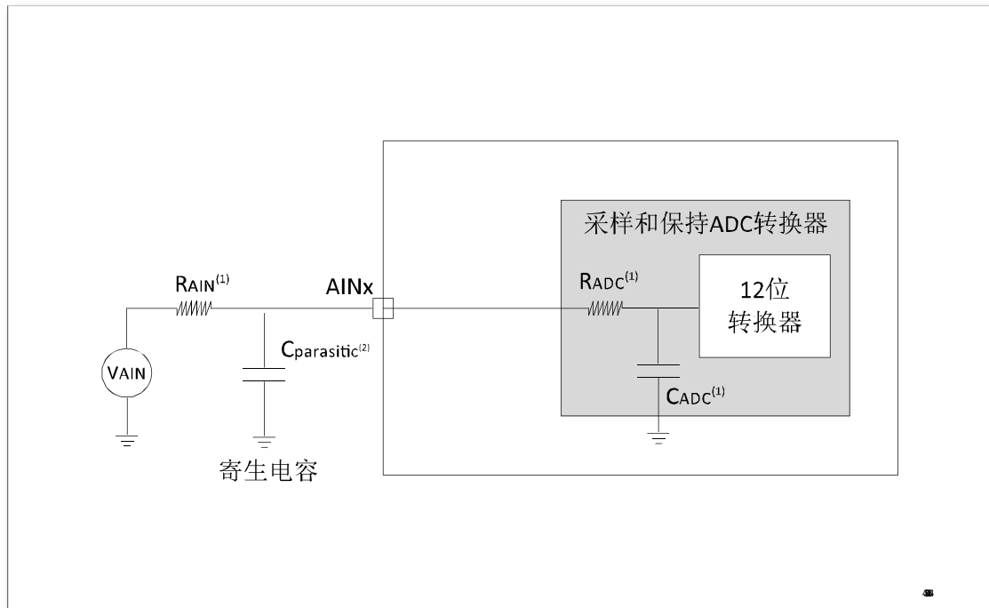
图 13 使用 ADC 典型的连接图
