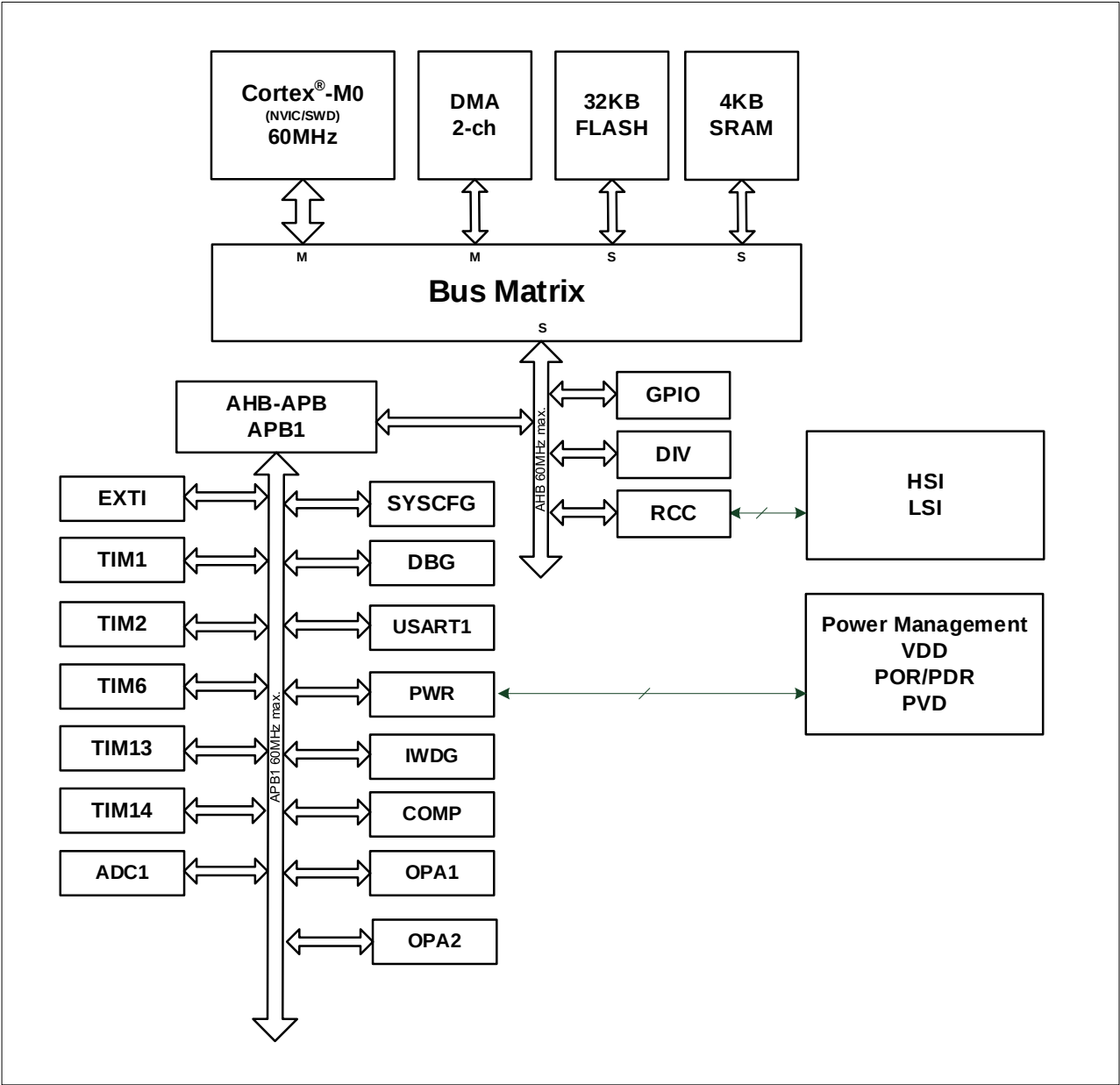
图1 模块框图
