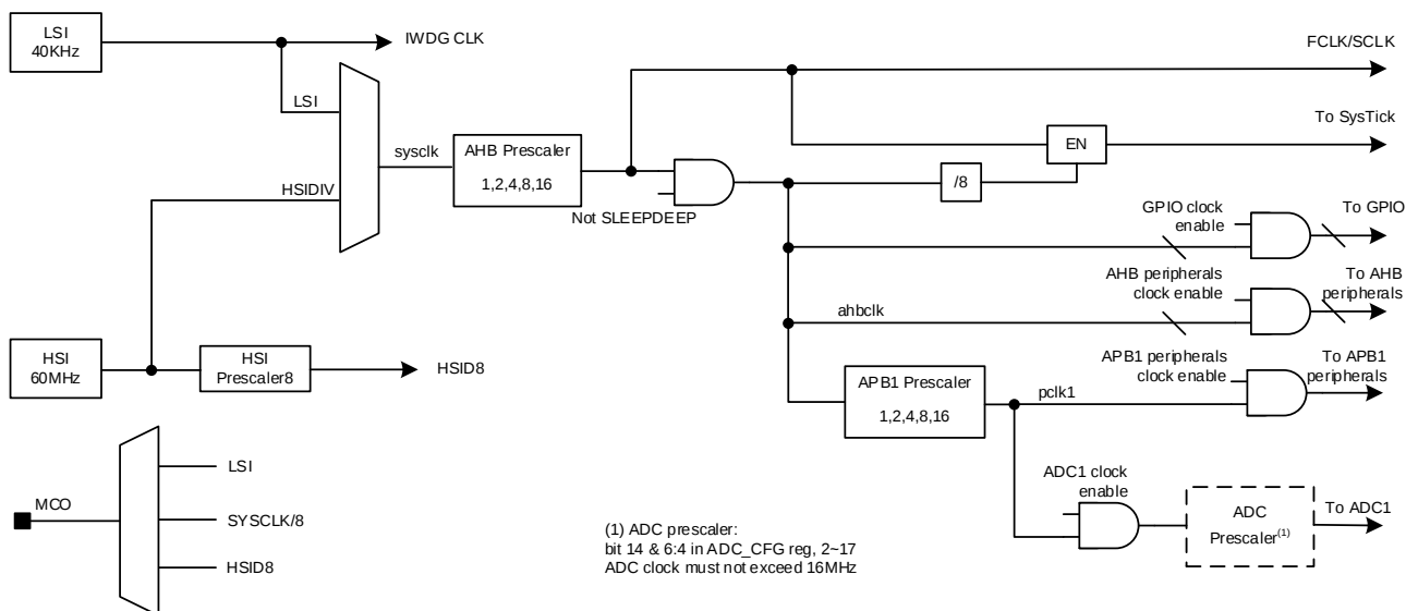
图2 时钟树
