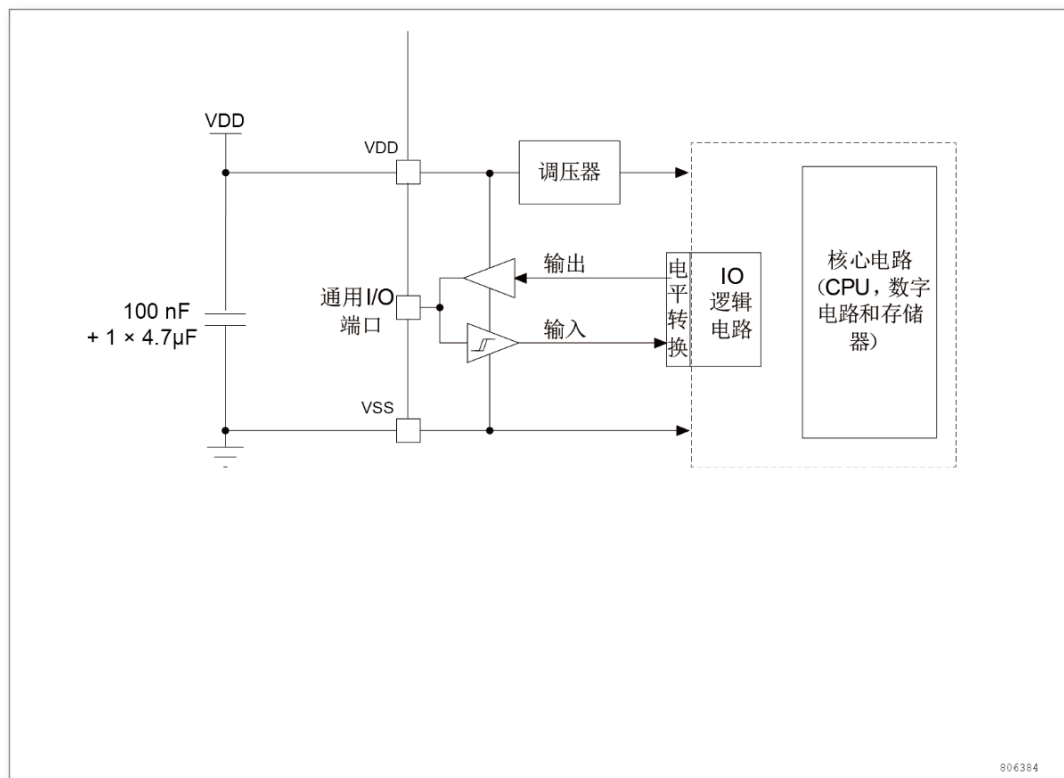
图 7 供电方案
