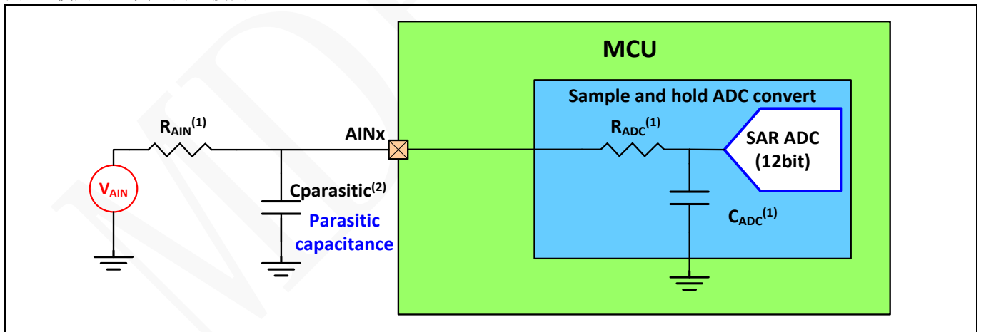
图 15 使用ADC典型的连接图
