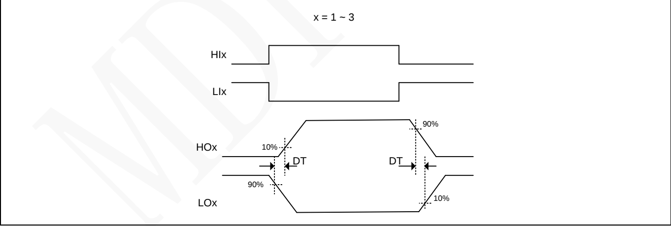
图 10 死区时间波形图
