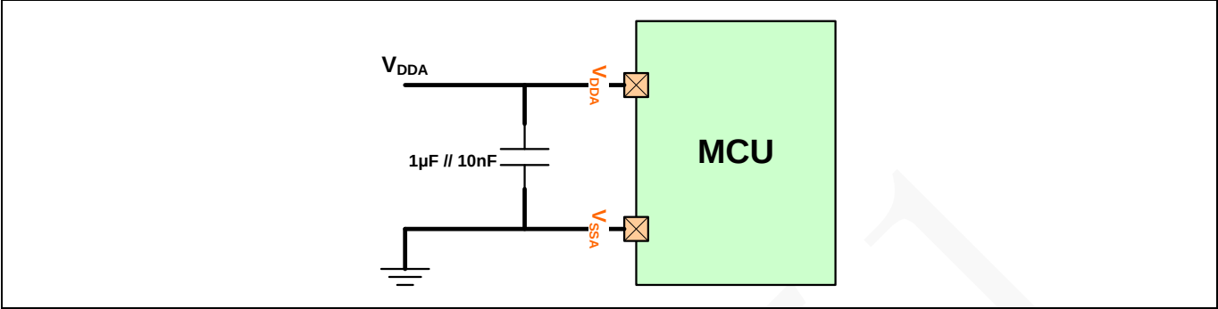
图 16 电源和参考电源去耦电路
