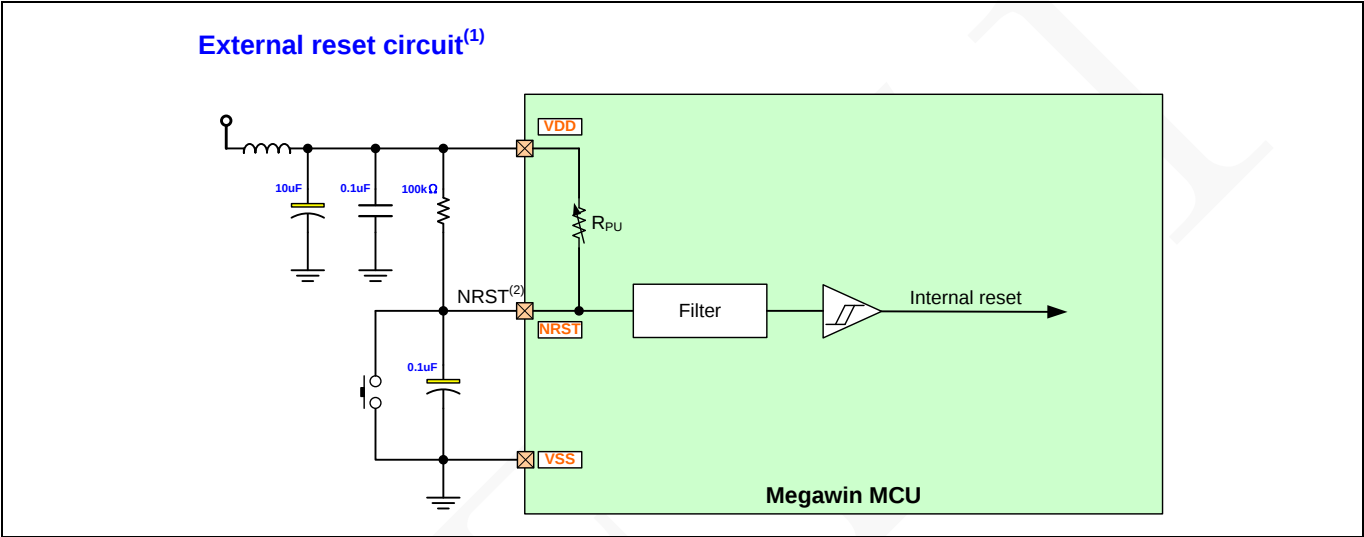
图 13 NRST引脚保护建议
