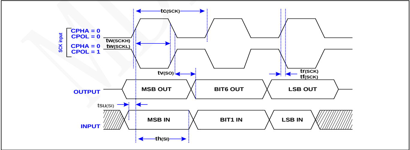
图 14 USART 同步时序
