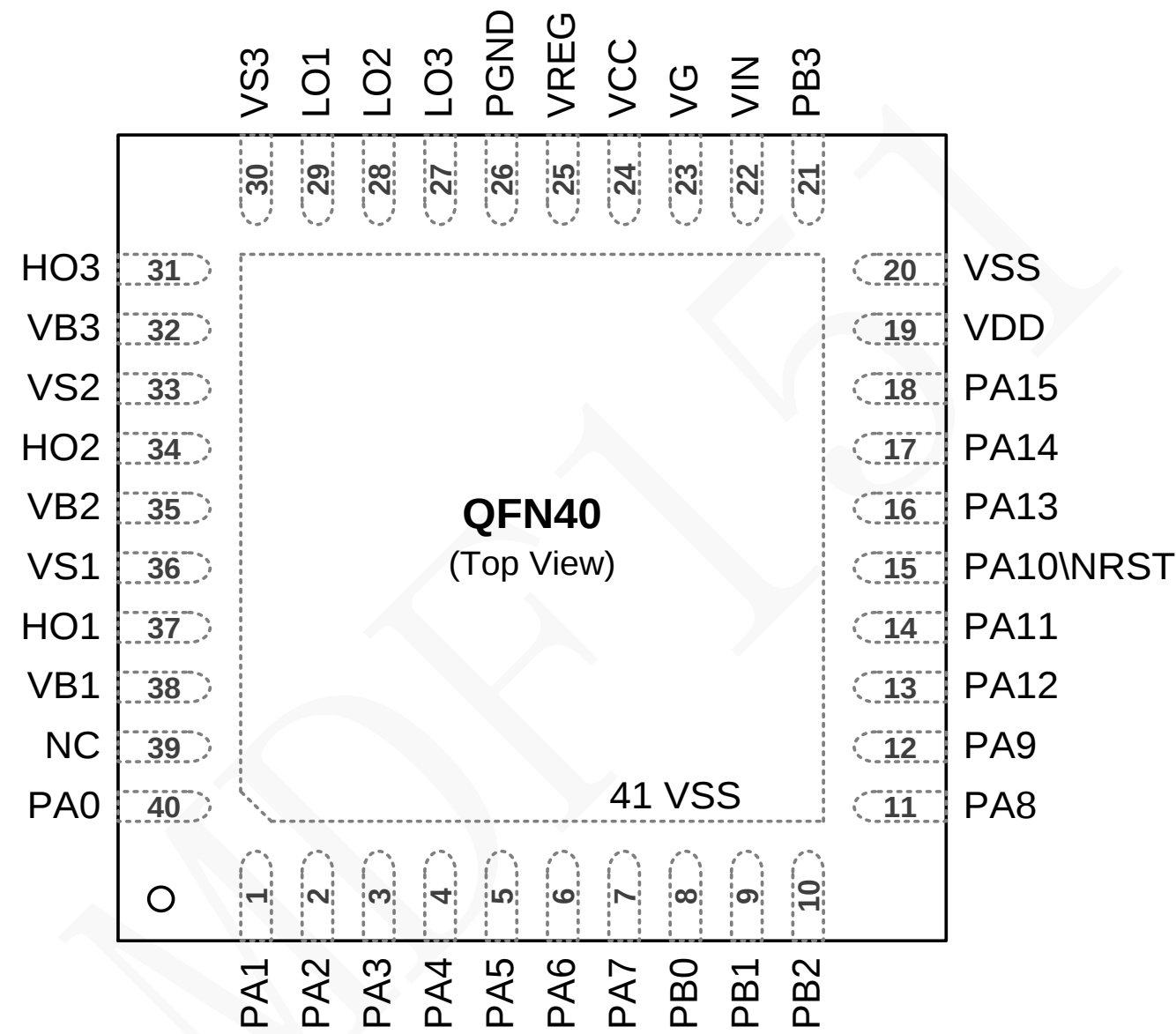
图 4 QFN40 引脚分布
