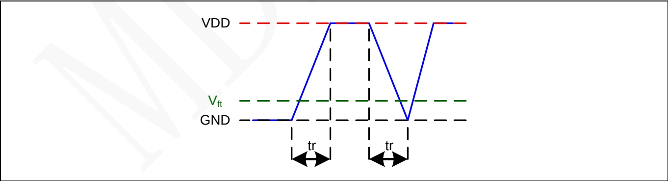
图 11 上电和掉电波形
