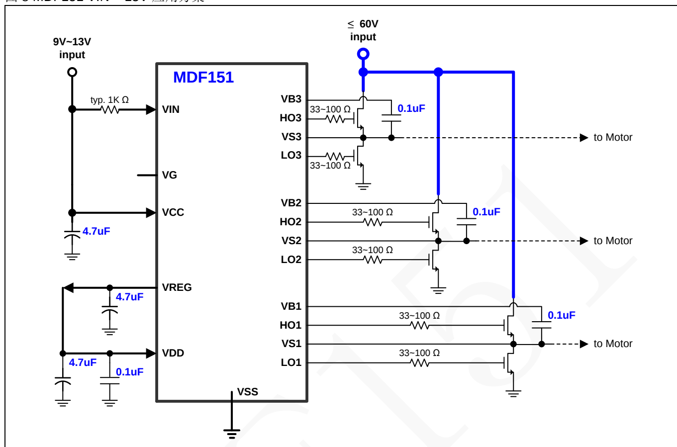
图 8 MDF151 VIN &lt; 13V 应用方案
