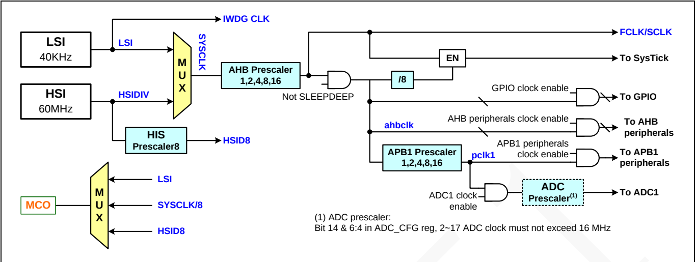
图 3 时钟树
