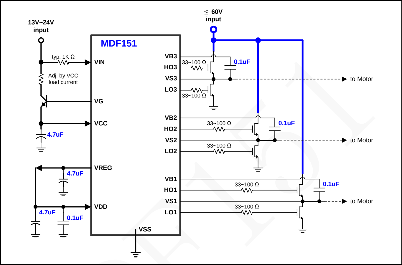
图 7 MDF151 VIN > 13V 应用方案
