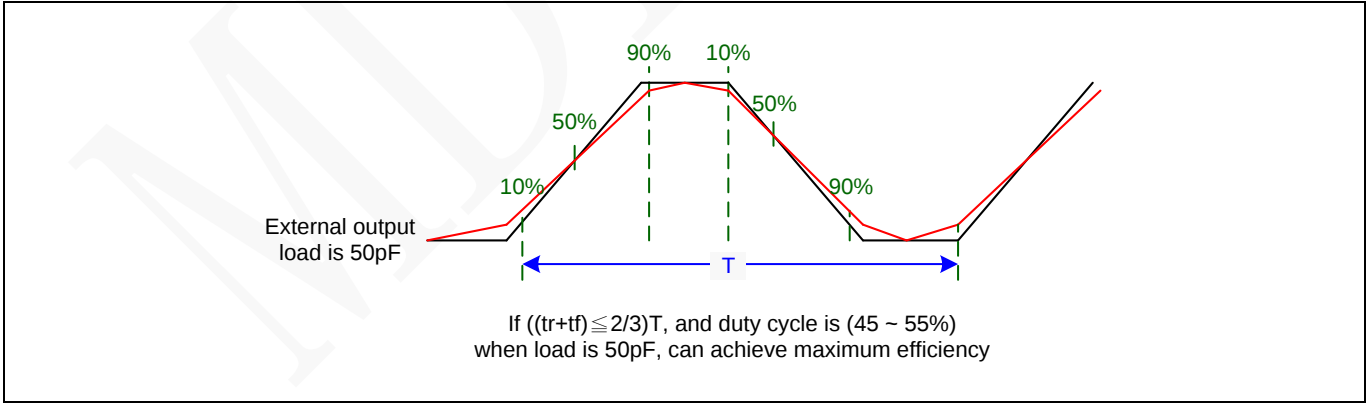
图 12 输入/输出交流特性定义
