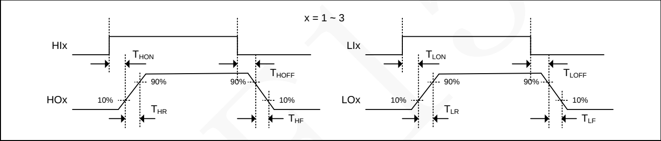
图 9 预驱输出波形图
