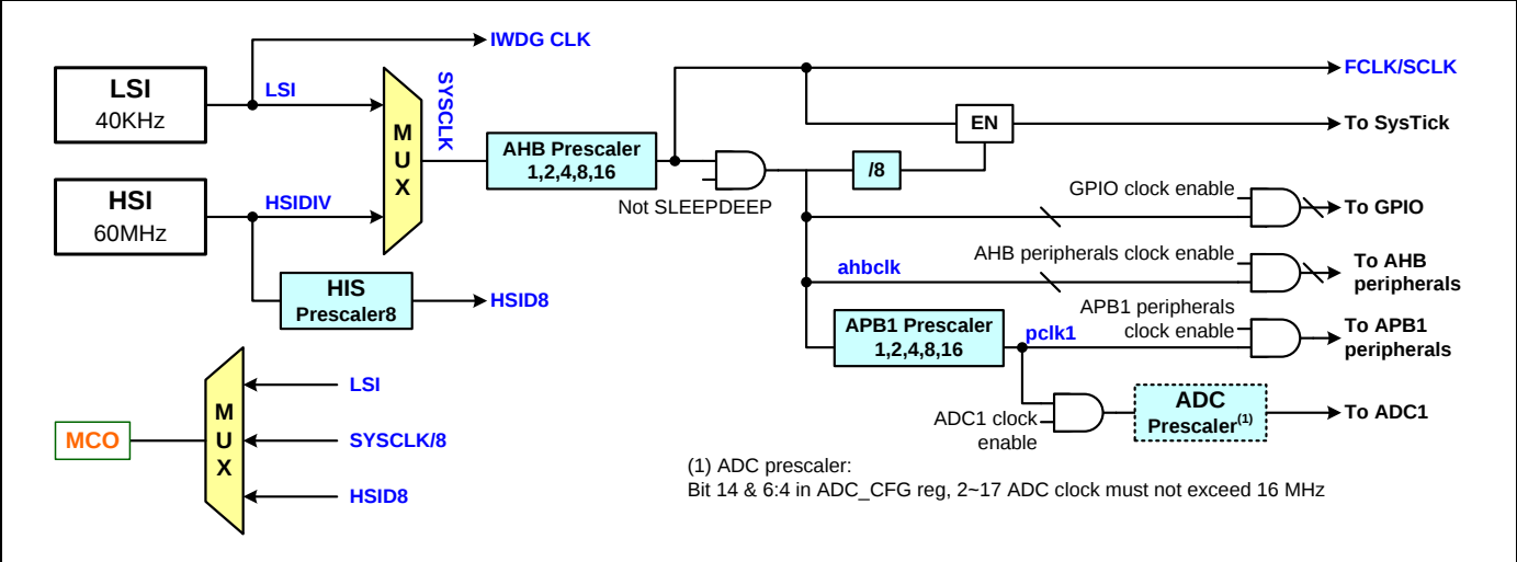
图 2 时钟树
