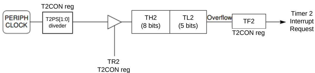
图 13.4.12 定时器 2 模式 0
