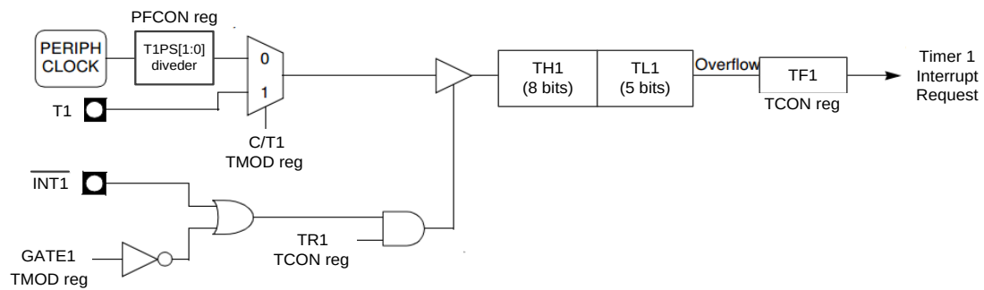
图 13.4.9 定时器 1 模式 0
