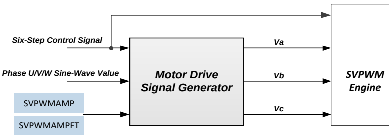
图 19.5.1：电机驱动信号发生器架构
