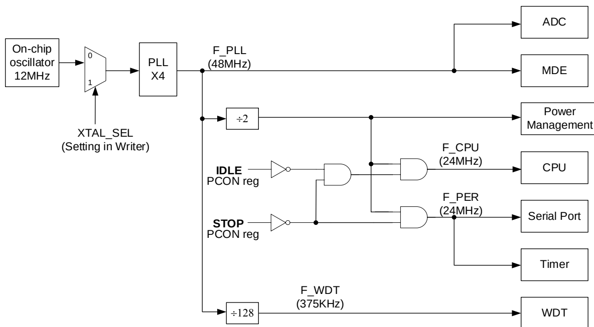
图 13.3 时钟结构
