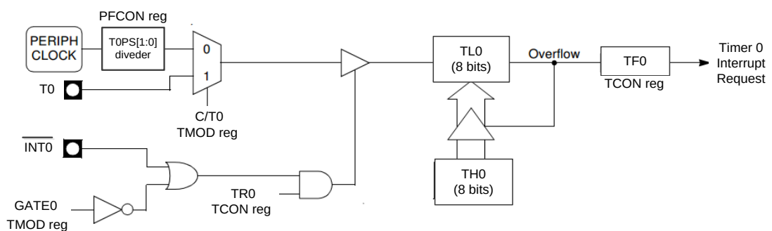
图 13.4.7 定时器0 模式 2
