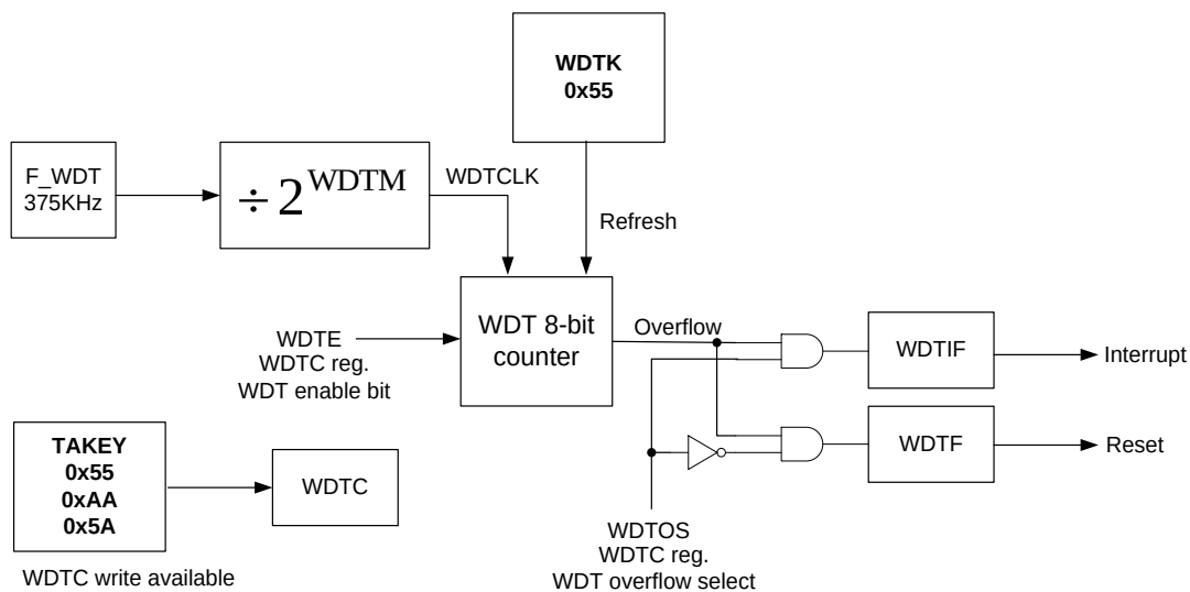
图 13.5 看门狗定时器
