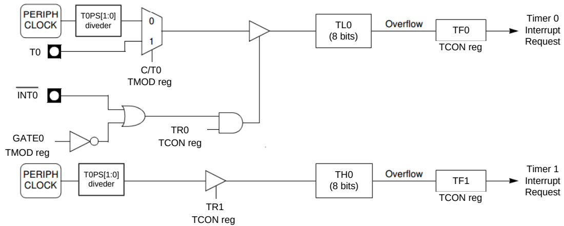
图 13.4.8 定时器 0 模式 3
