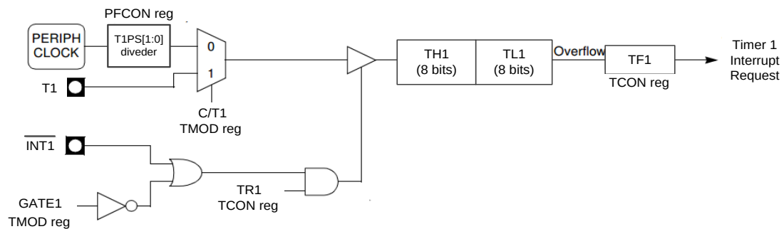
图 13-4.10 定时器 1 模式 1
