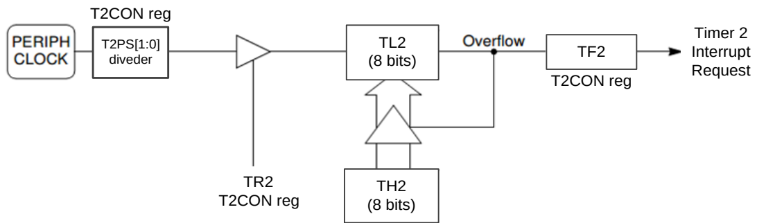
图 13.4.14 定时器 2 模式 2
