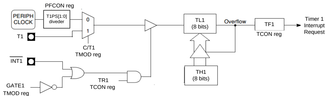
图 13.4.11 定时器 1 模式 2
