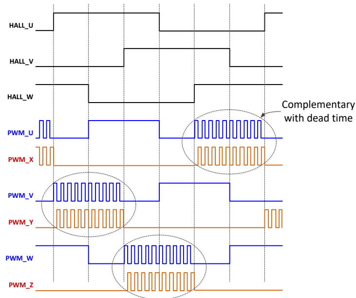
图 19.6.6：单极 PWM 开关
