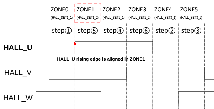
图 19.3.4 Hall_U 上升沿对齐在 ZONE1.
