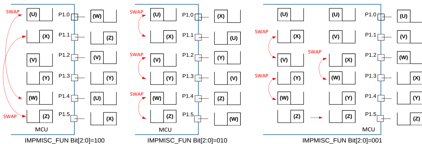
图 19.6.9 : PWM 引脚交换
