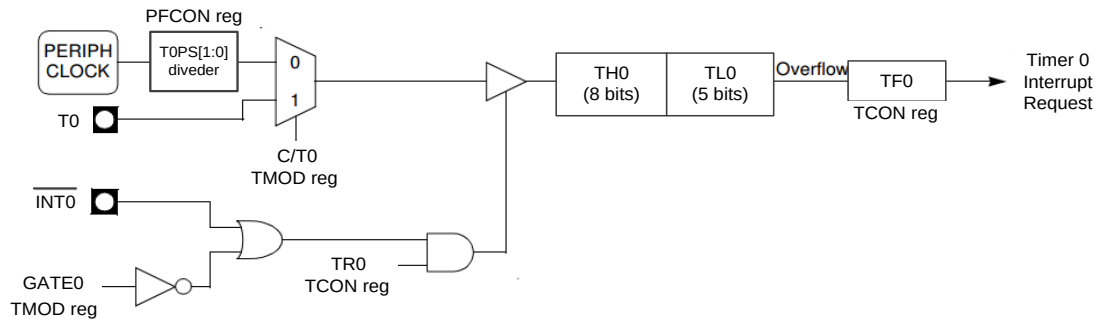
图 13.4.5 定时器 0 模式 0
