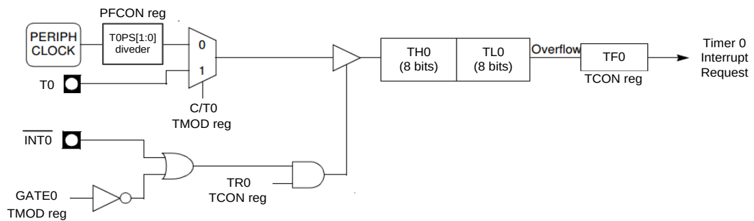
图 13.4.6 定时器 0 模式 1
