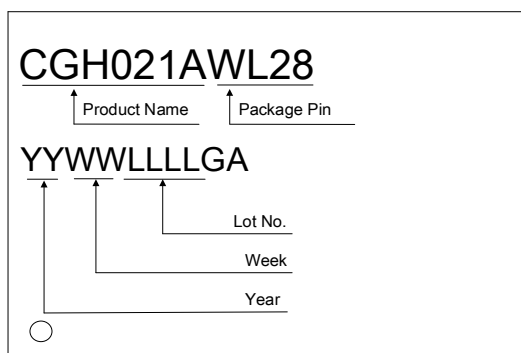
图 22.1 标准丝印 (w/o 代码) SSOP28W 209mil
