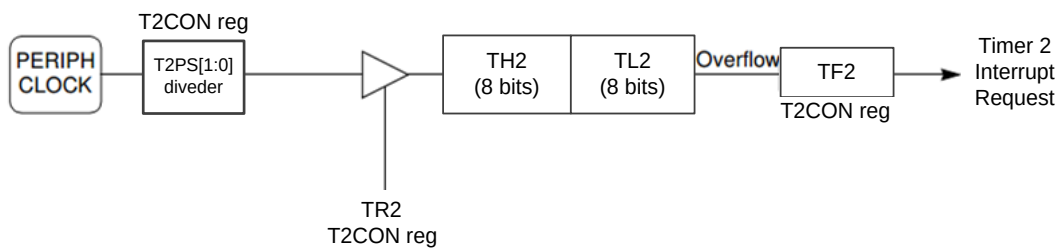
图 13.4.13 定时器 2 模式 1
