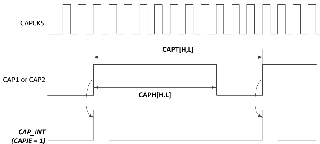
图 16.1 捕获
