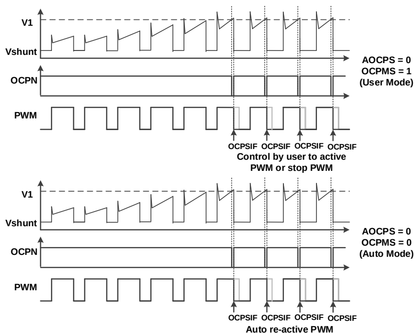
图 19.7.2：数字 OCP 短路发生和 PWM 输出
