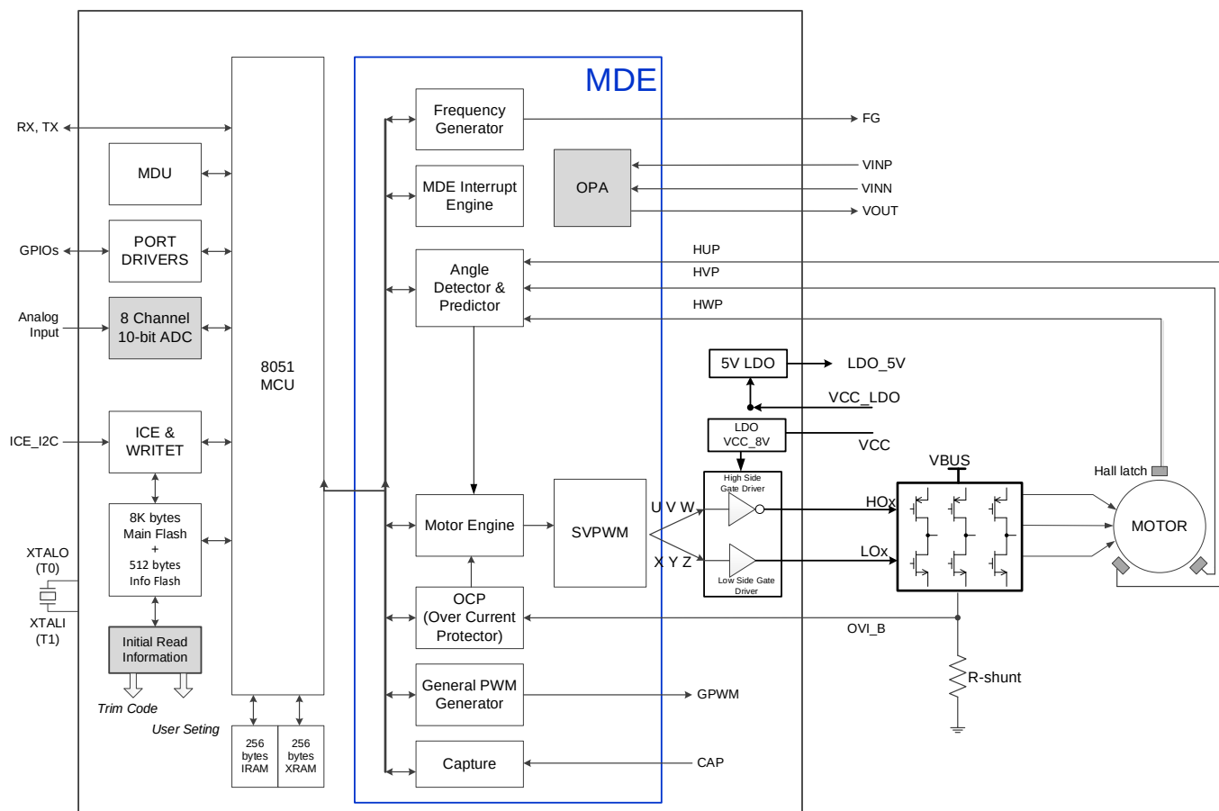
图 2.1 CGH021A BLDC 电机控制器模块图
