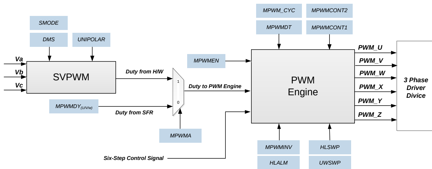
图 19.6.1 : SVPWM 引擎模块架构
