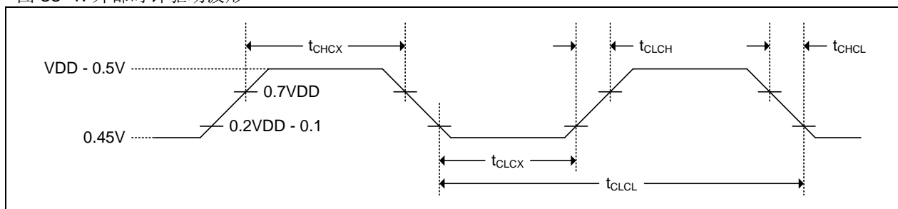
图 33-1. 外部时钟驱动波形
