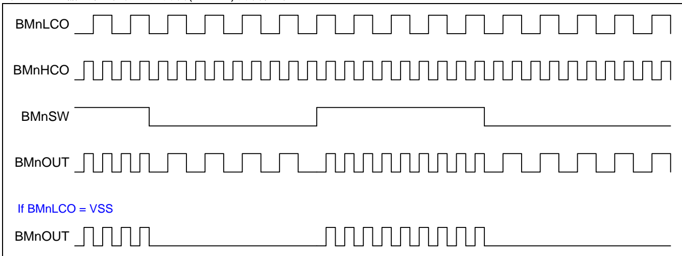
图 24-1. 输出信号中止和调制(OBMn)调制信号
