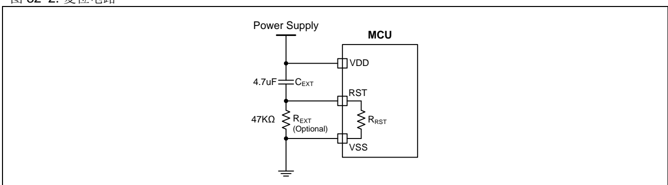
图 32-2. 复位电路
