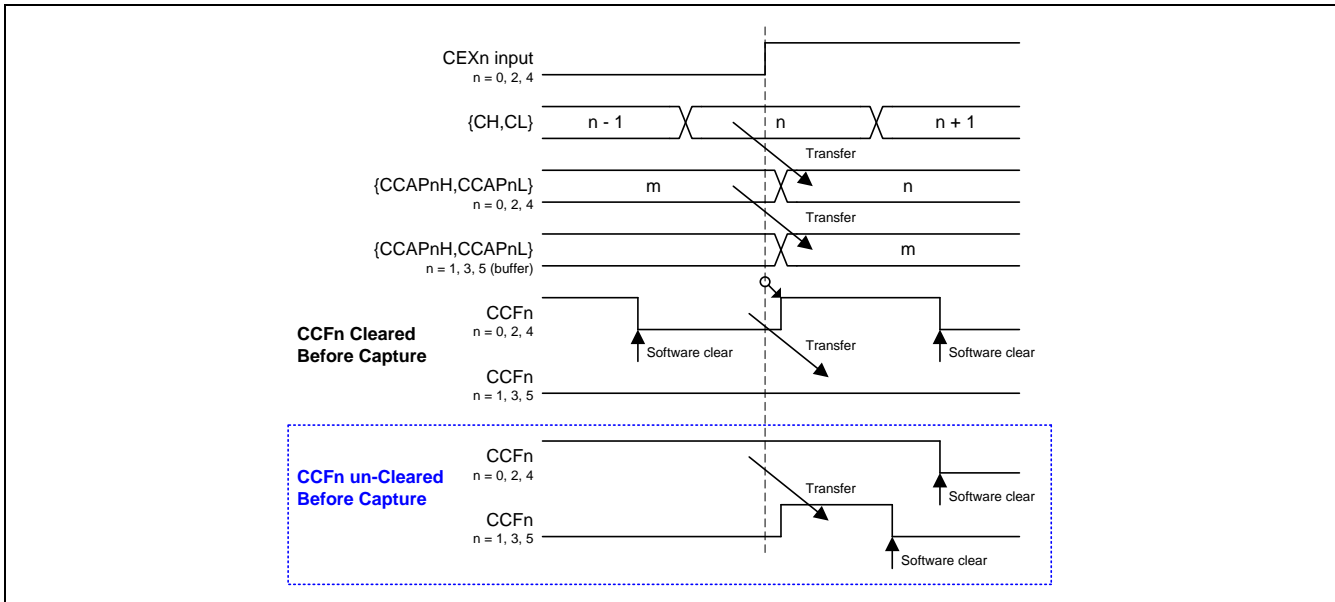
图 16-6. PCA0 缓冲捕获模式波形
