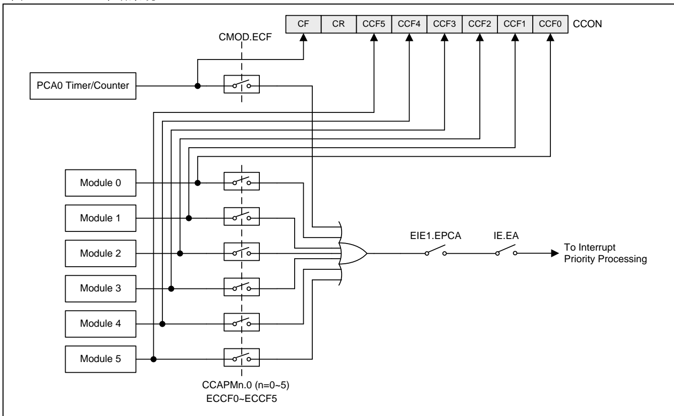
图 16-3. PCA0 中断系统
