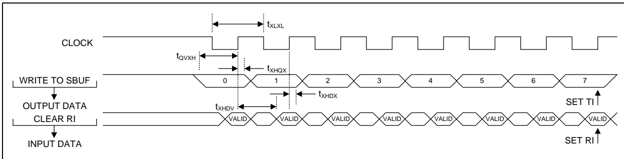
图 33-2. 移位寄存器模式时序波形
