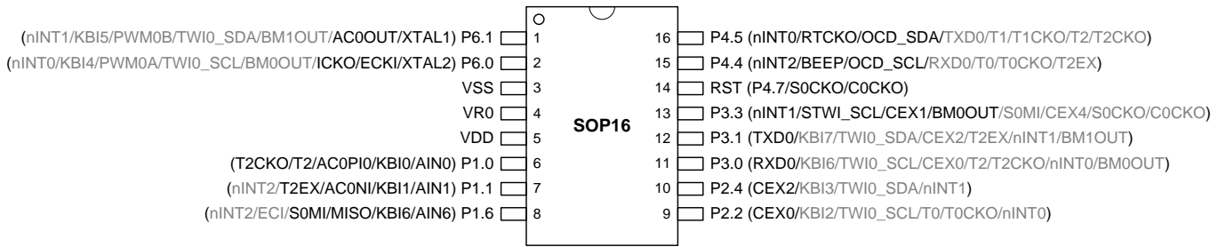
图 4-4. SOP16 顶视图
