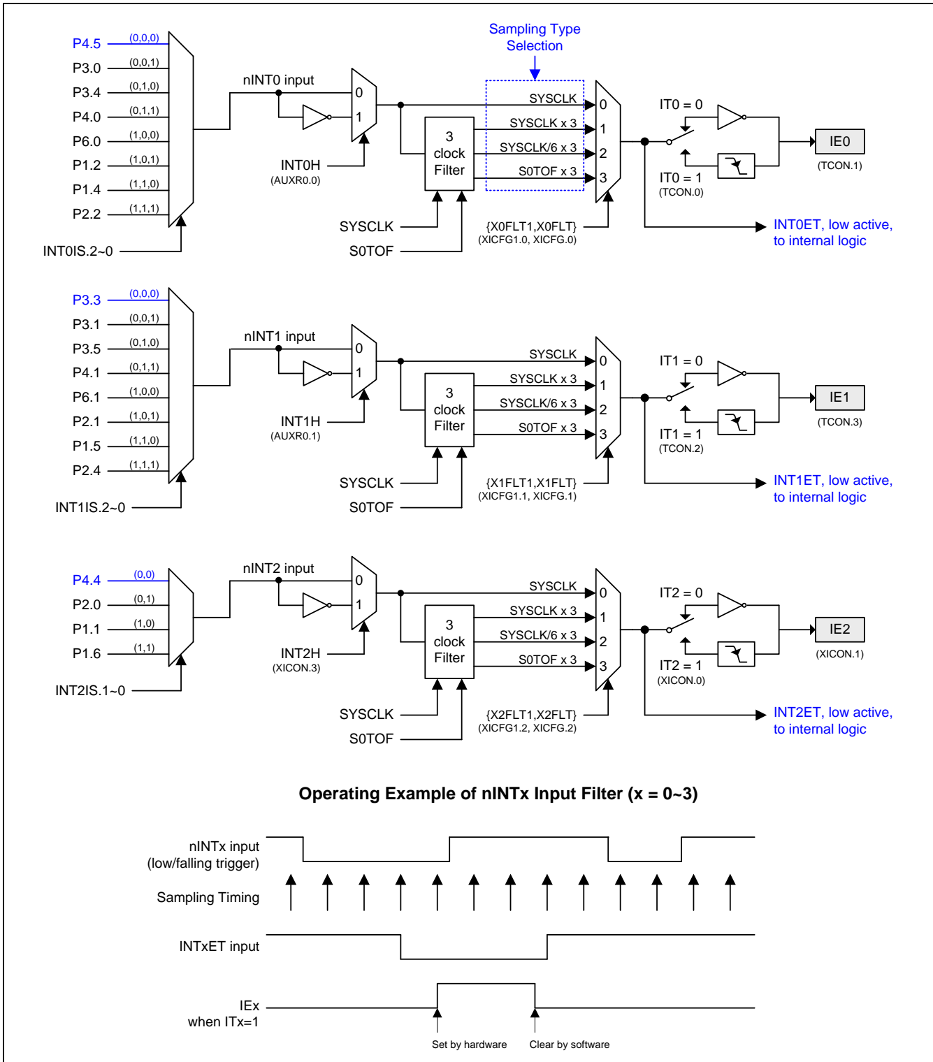
图 14-2. nINT0~2端口引脚选择结构
