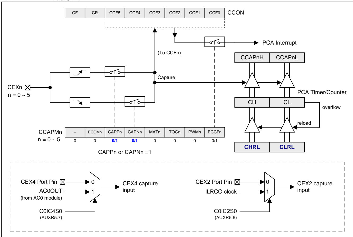
图 16-4. PCA0 捕获模式
