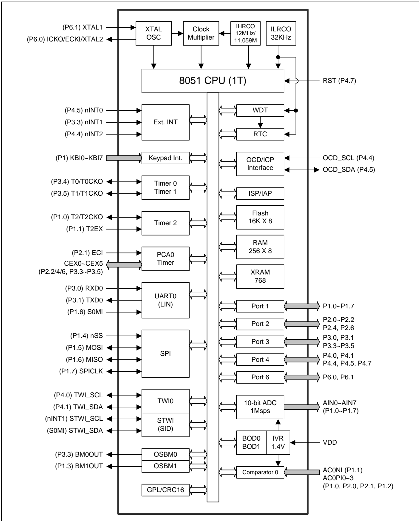
图 2-1. 方框图
