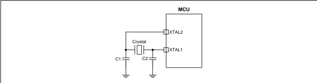
图 32-3. XTAL 振荡电路
