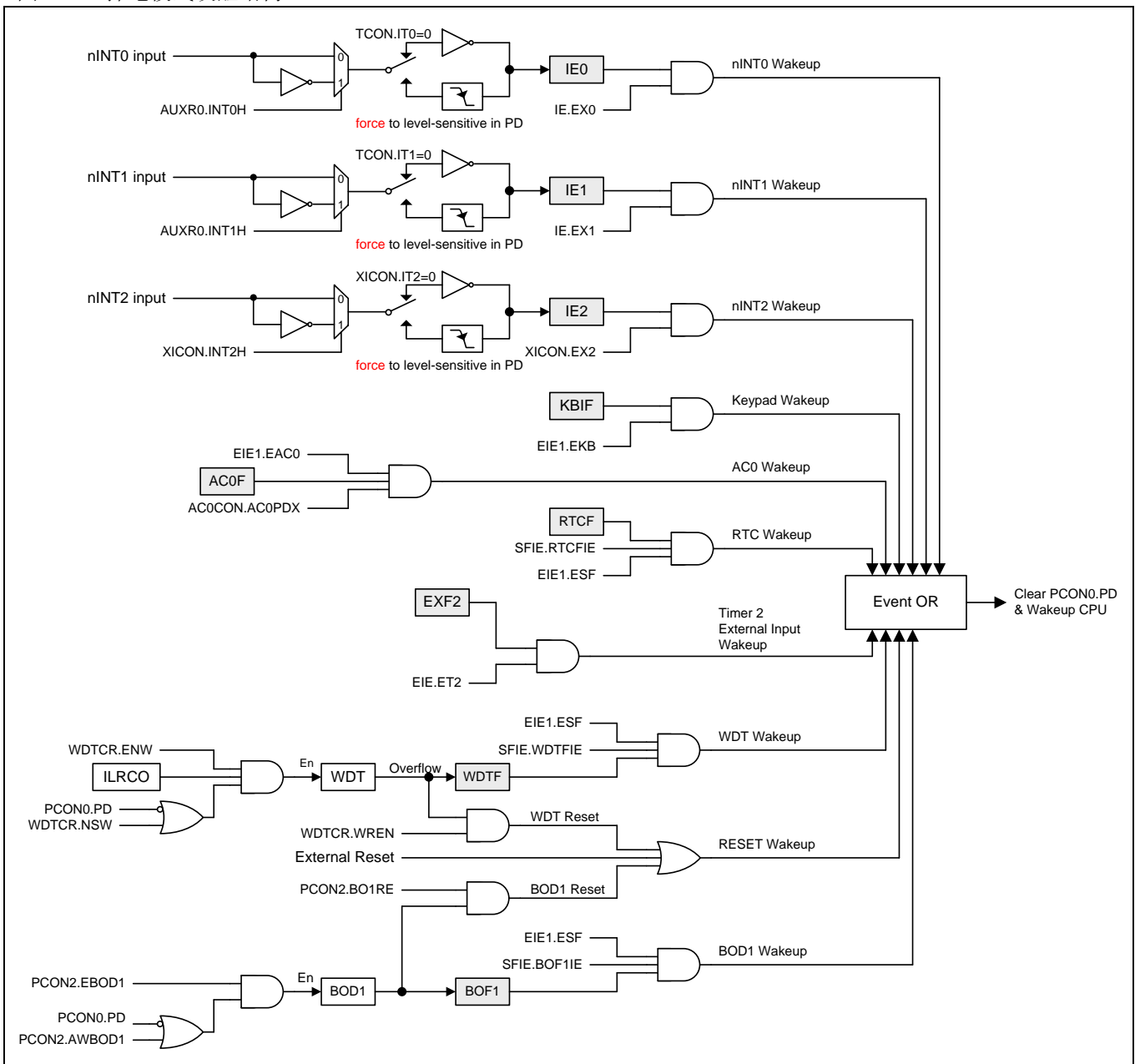
图 12-2. 掉电模式唤醒结构
