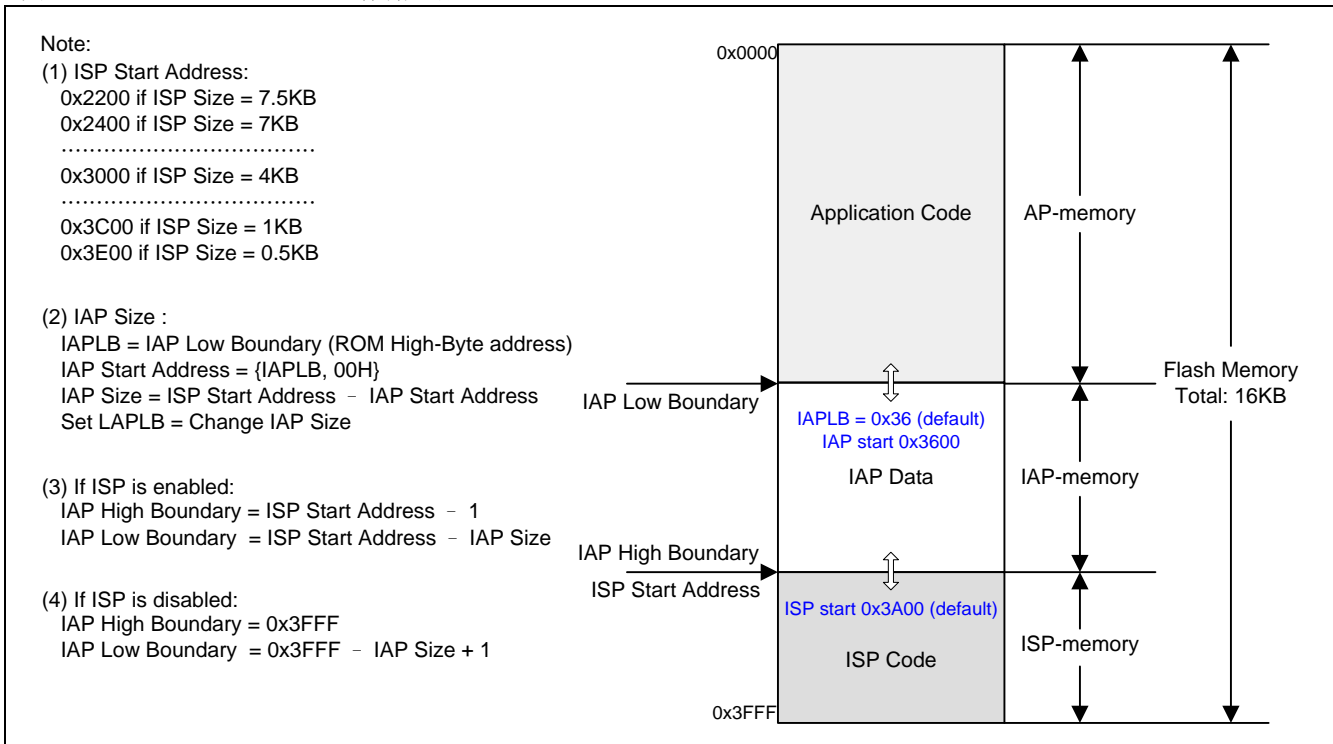
图 28-1. MG82F6D16 Flash 存储器配置
