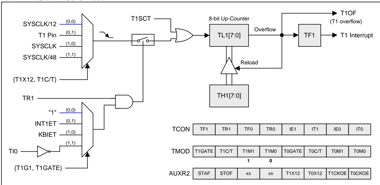
图 15-6. 定时器 1 模式 2 结构
