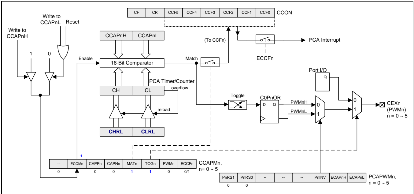
图 16-8. PCA0 高速输出模式
