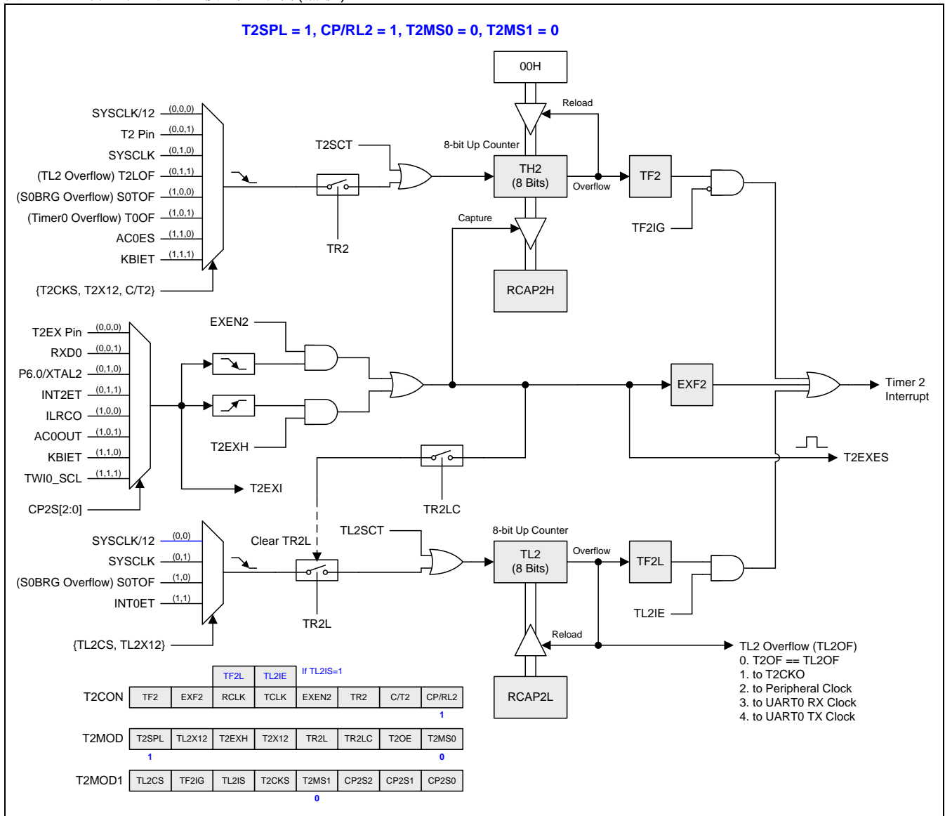
图 15-18. 分立定时器 2 模式 2 结构(捕获)
