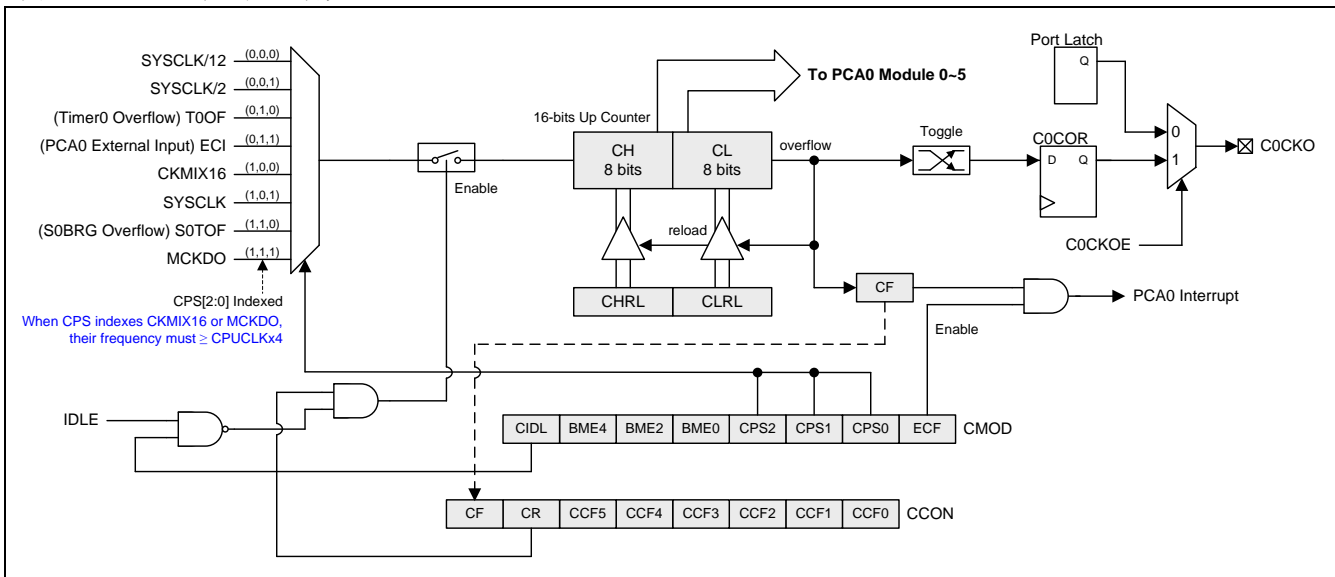
图 16-2. PCA0 定时器/计数器
