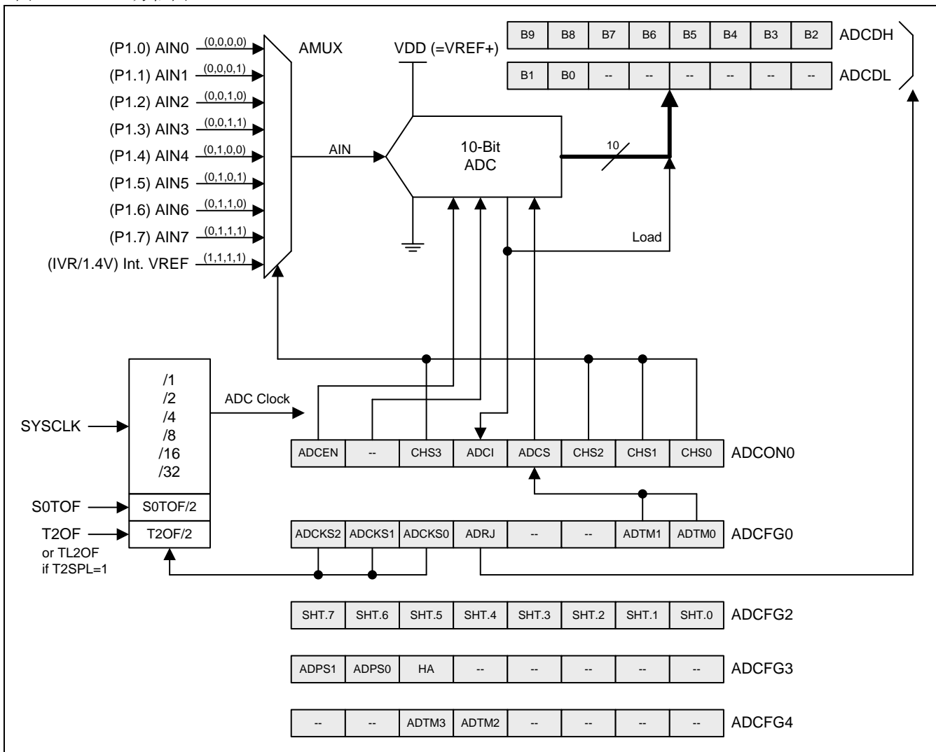
图 25-1. ADC 方框图
