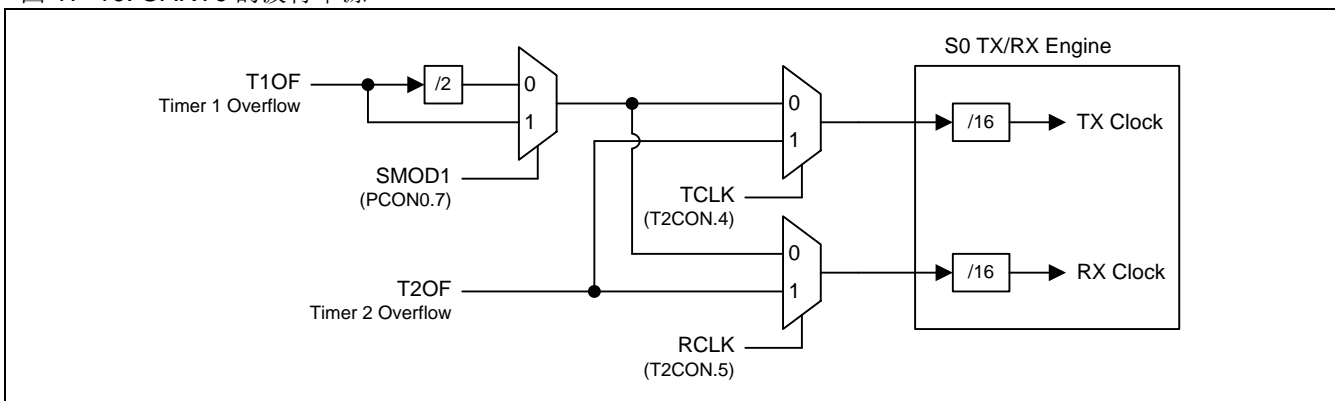
图 17-10. UART0 的波特率源
