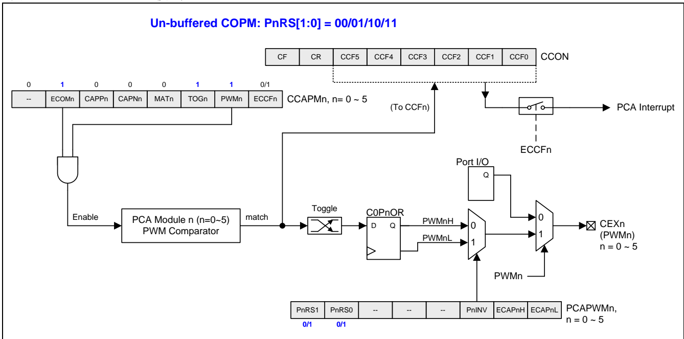
图 16-12. PCA0 COPM 模式
