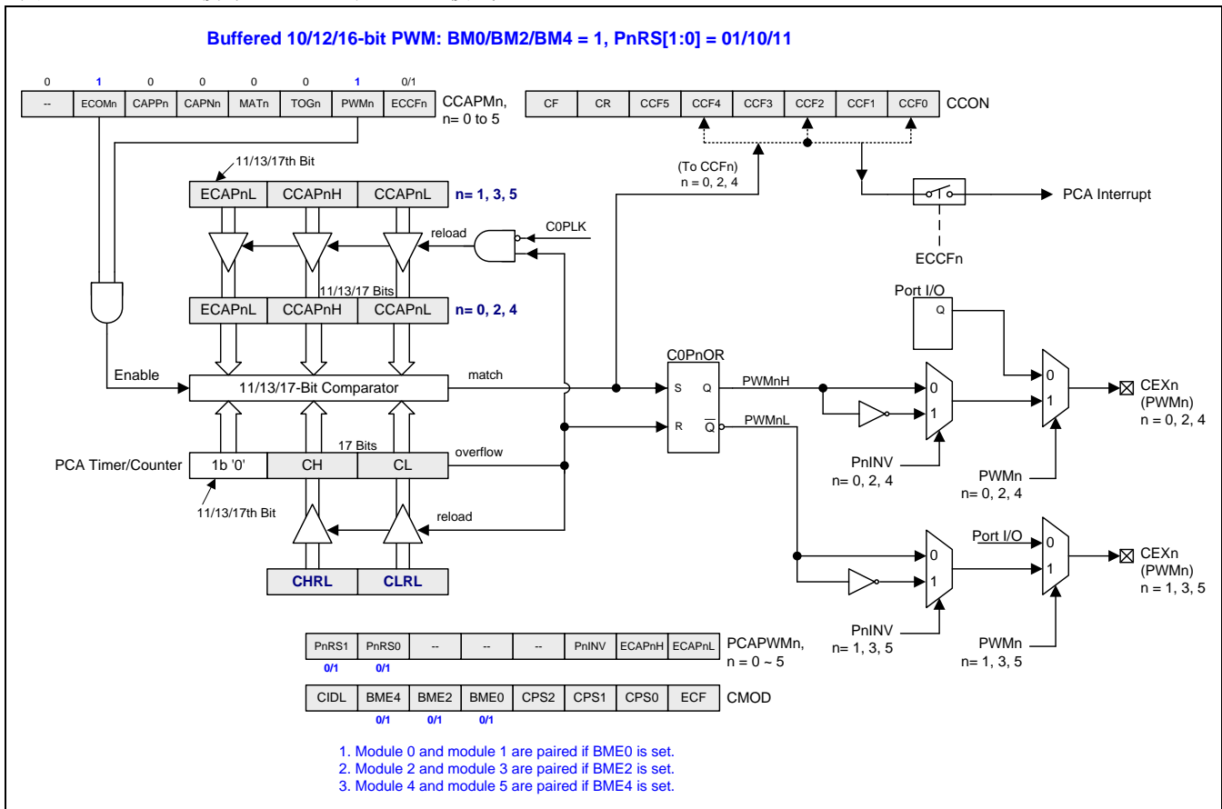
图 16-11. PCA0 缓冲 10/12/16 位 PWM 模式
