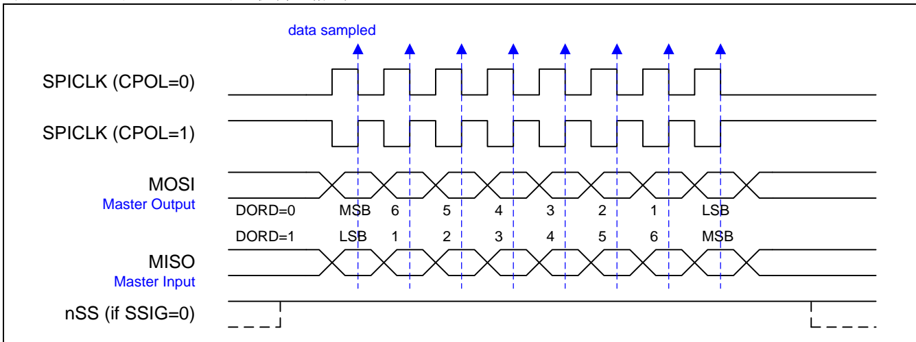
图 18-9. SPI 在 CPHA=1 时主机传送格式
