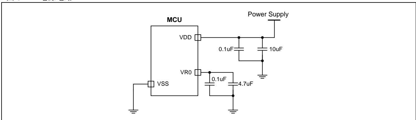
图 32-1. 电源电路
