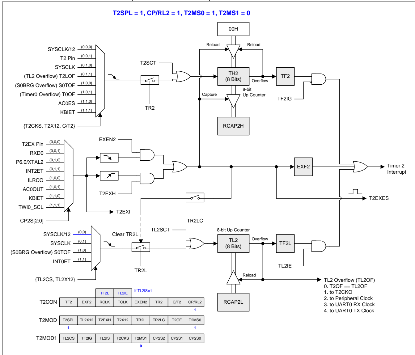
图 15-19. 分立定时器 2 模式 3 结构(捕获带自动清零 TH2)
