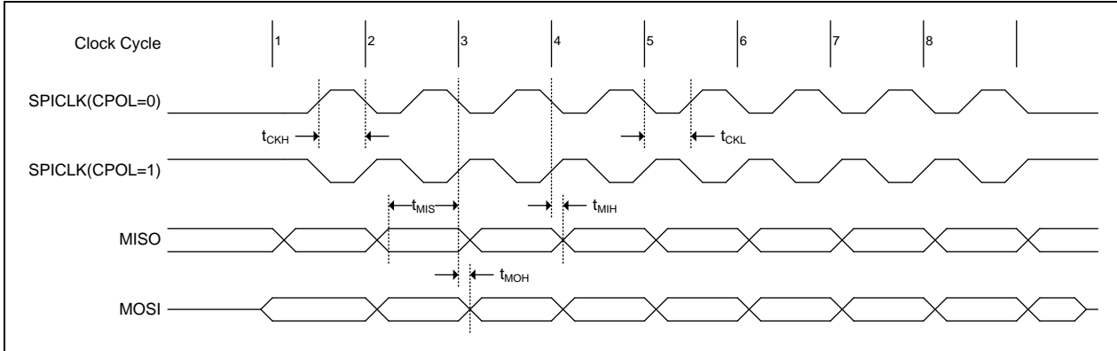
图 33-3. CPHA=0 时 SPI 主机传送波形
