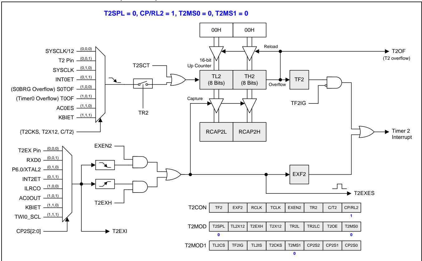
图 15-14. 定时器 2 模式 2 结构(捕获模式)
