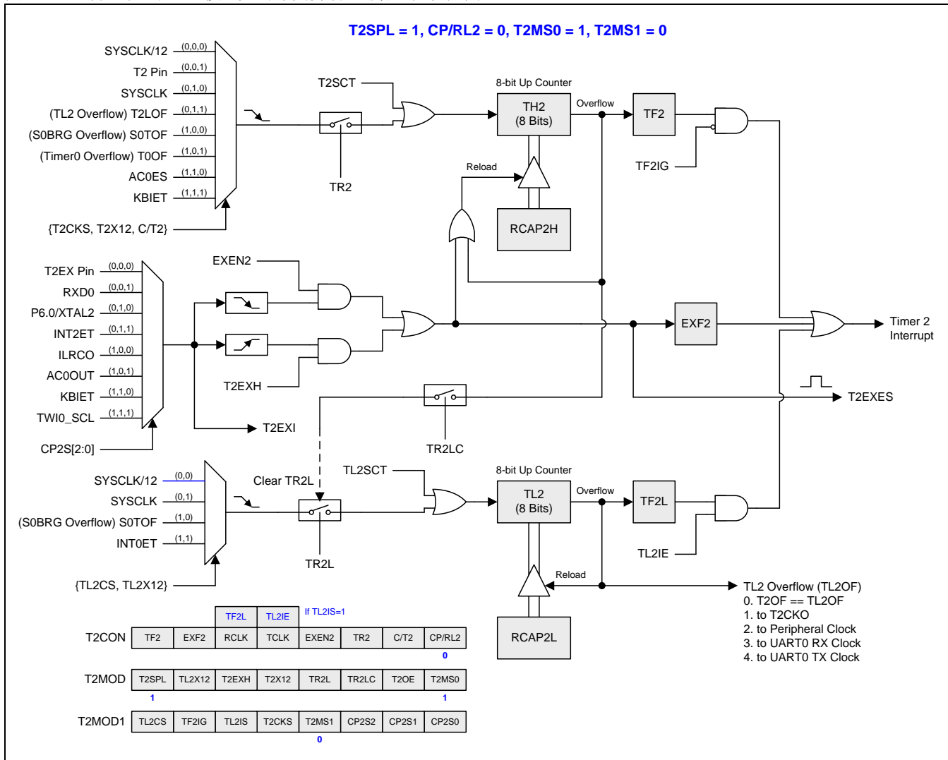
图 15-17. 分立定时器 2 模式 1 结构(自动重载和外部中断)
