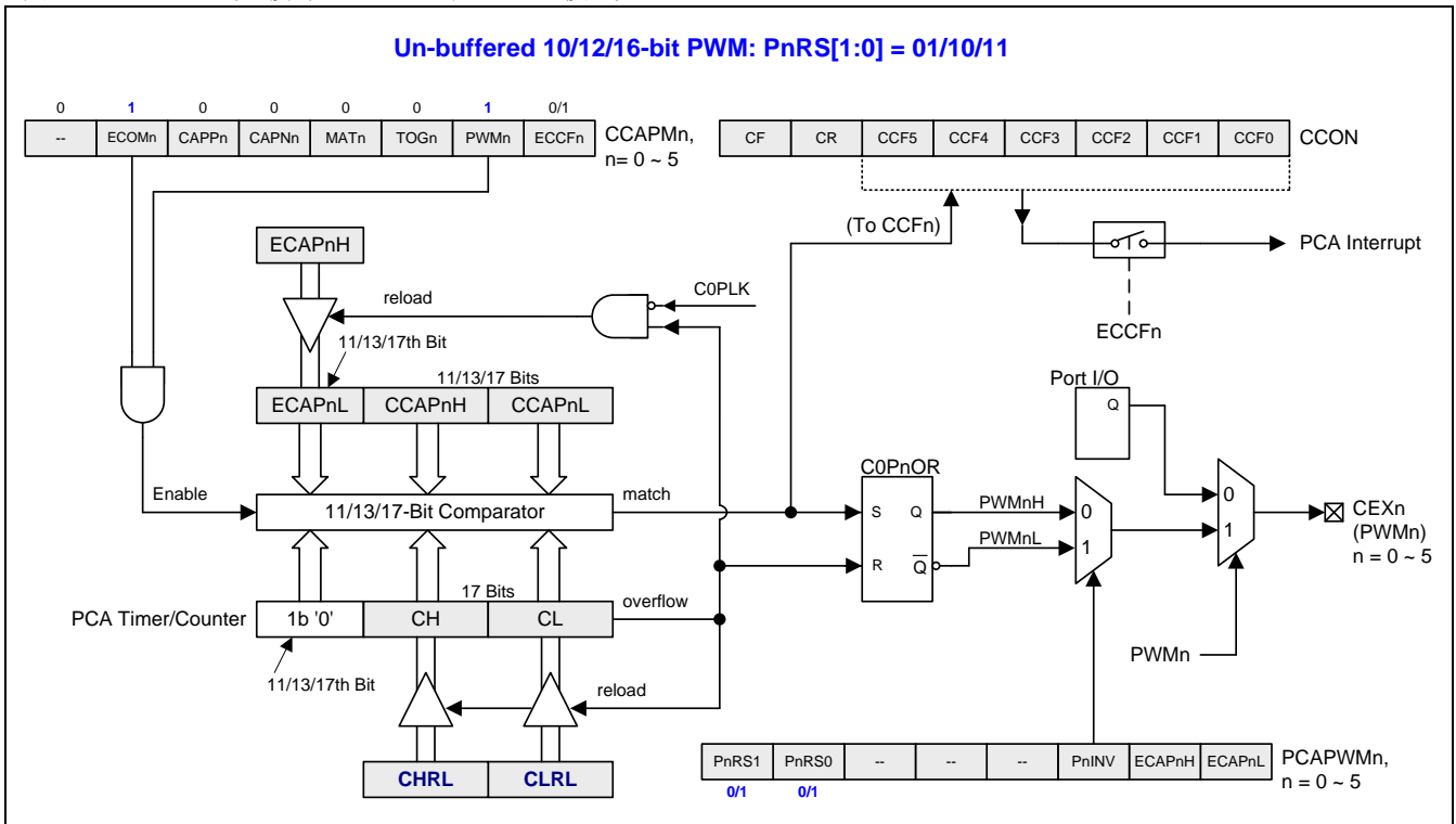
图 16-10. PCA0 无缓冲 10/12/16 位 PWM 模式
