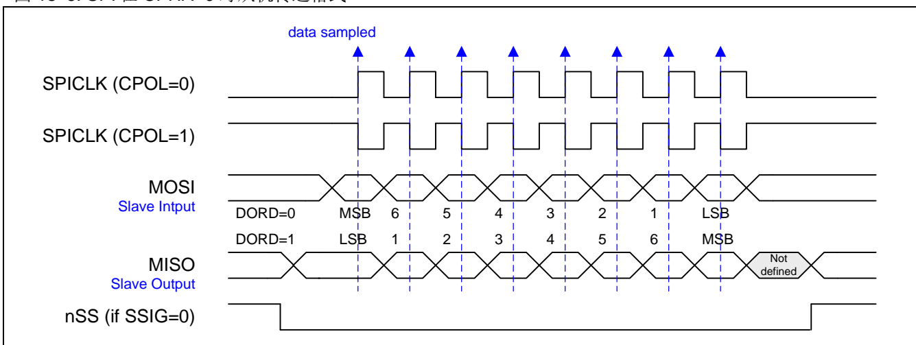
图 18-6. SPI 在 CPHA=0 时从机传送格式
