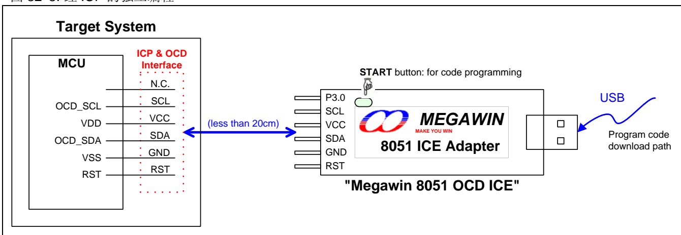
图 32-5. 经 ICP 的独立编程
