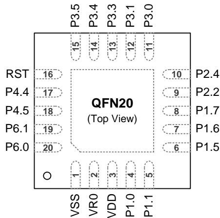
图 4-3. QFN20 顶视图
