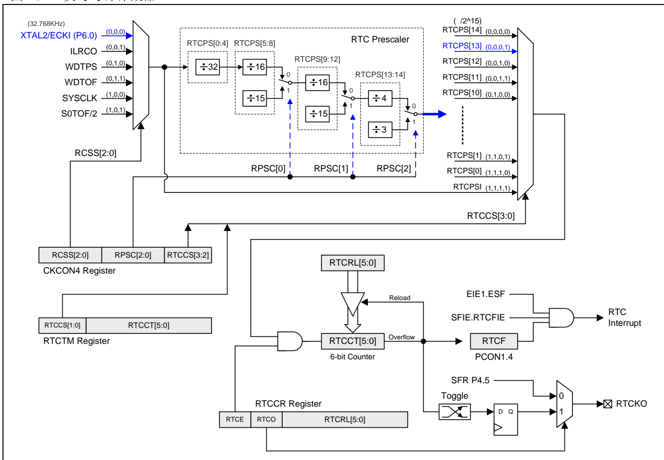
图 10-1. 实时时钟计数器
