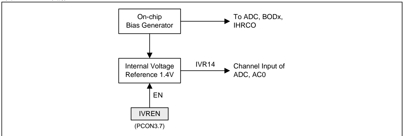
图 27-1. IVR 图解
