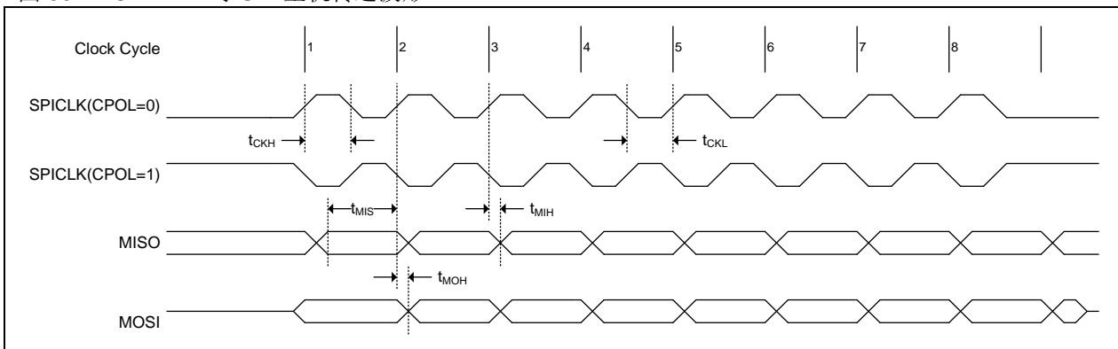
图 33-4. CPHA=1 时 SPI 主机传送波形
