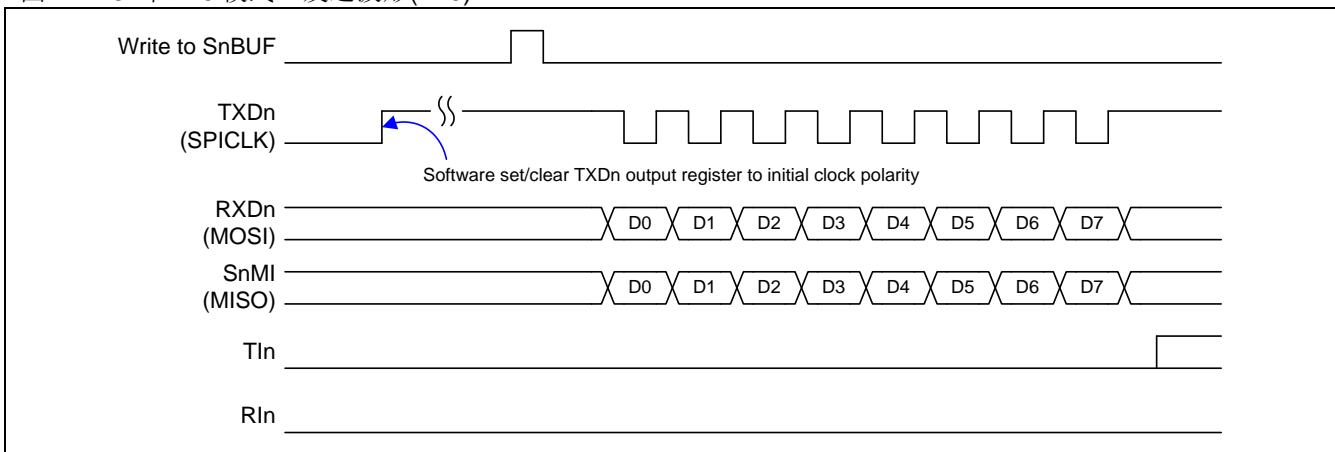
图 17-13. 串口 0 模式 4 发送波形(n=0)
