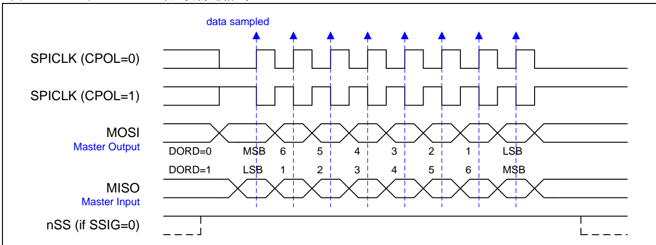
图 18-8. SPI 在 CPHA=0 时主机传送格式
