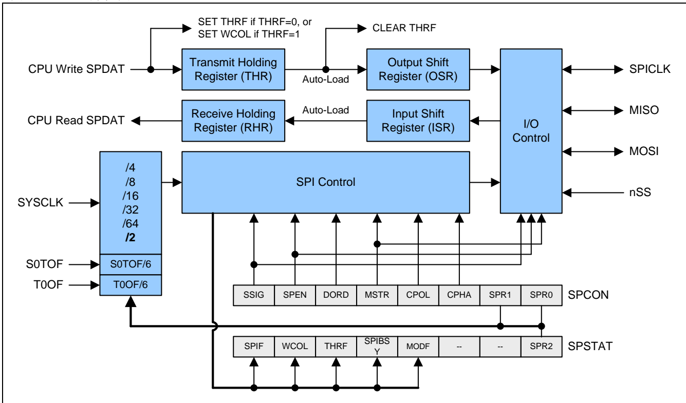
图 18-1. SPI 方框图
