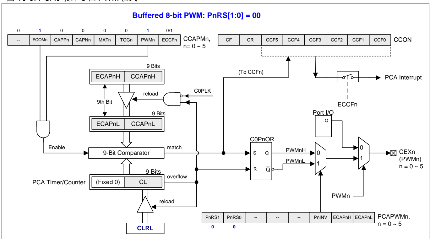
图 16-9. PCA0 缓冲 8 位 PWM 模式
