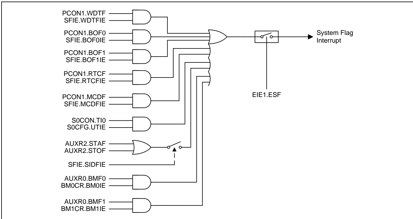
图 14-2. 系统标志中断结构
