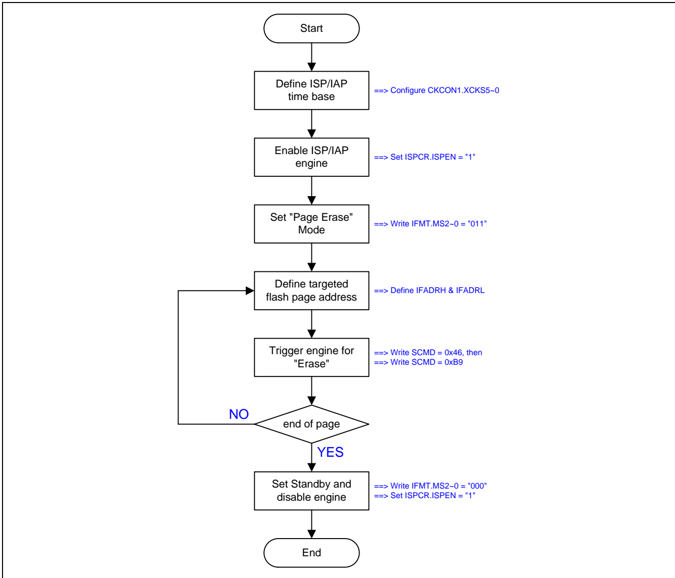
图 28-2. ISP/IAP 页擦除流程
