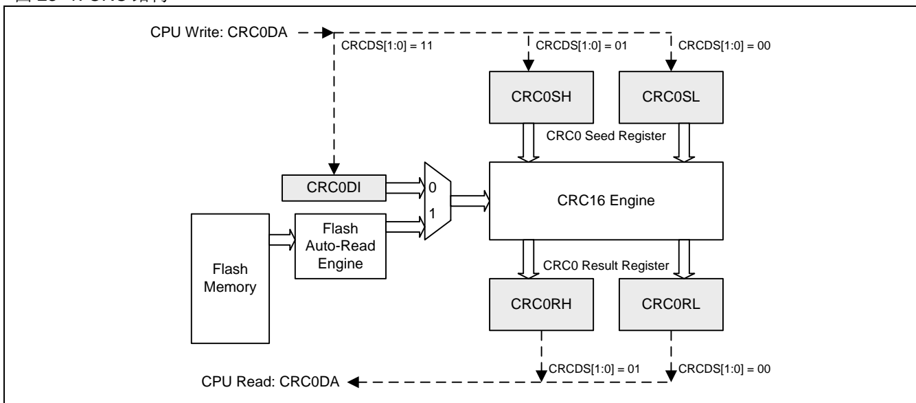
图 23-1. CRC 结构
