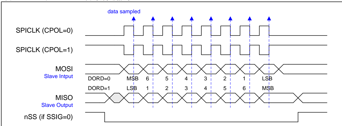
图 18-7. SPI 在 CPHA=1 时从机传送格式
