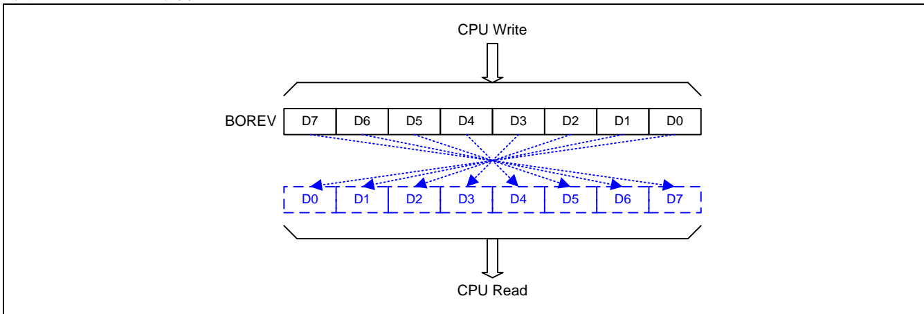
图 23-2. BOREV 结构
