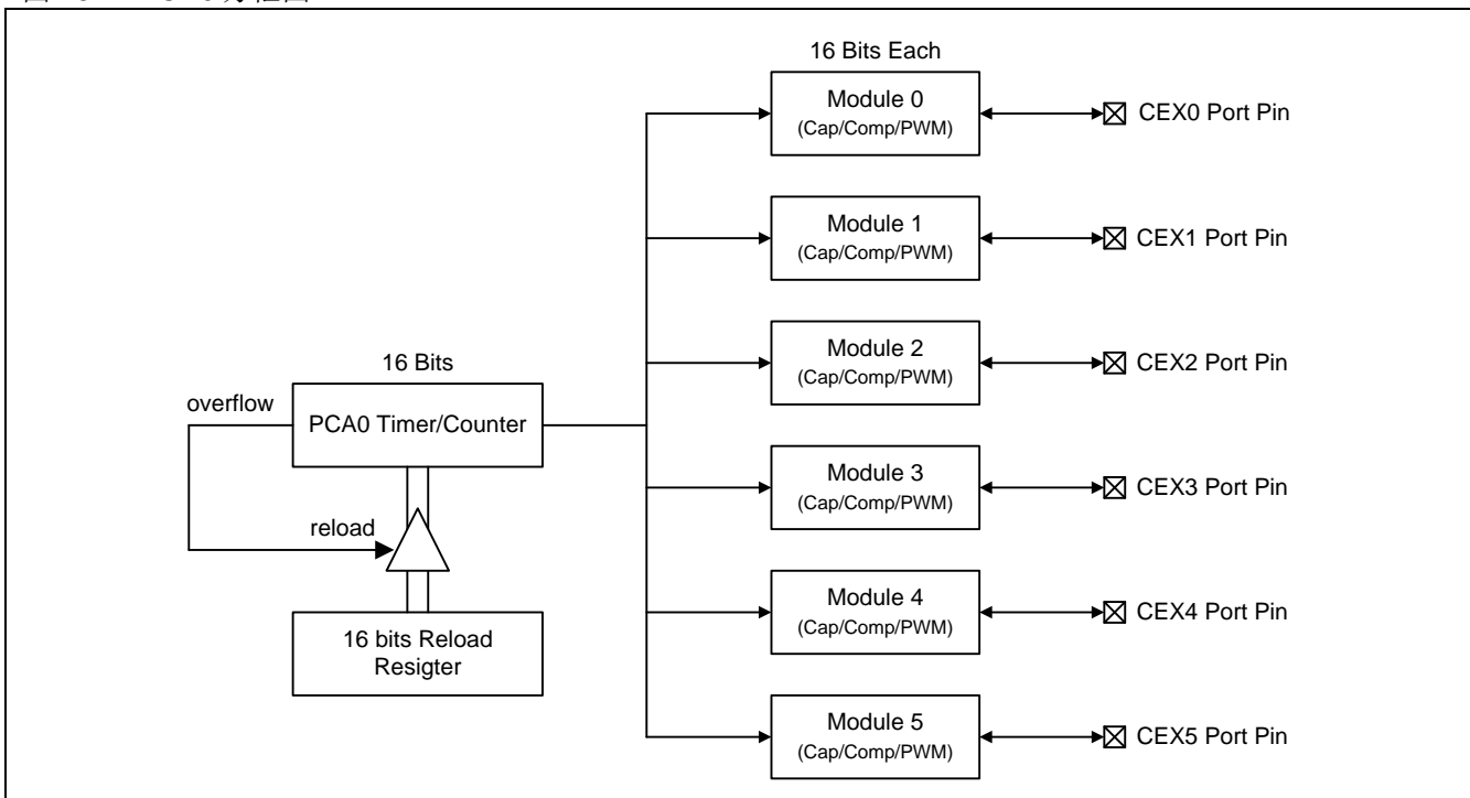
图 16-1. PCA0 方框图
