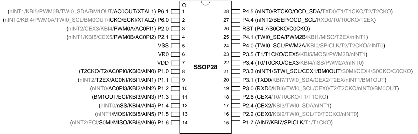
图 4-1. SSOP28 顶视图
