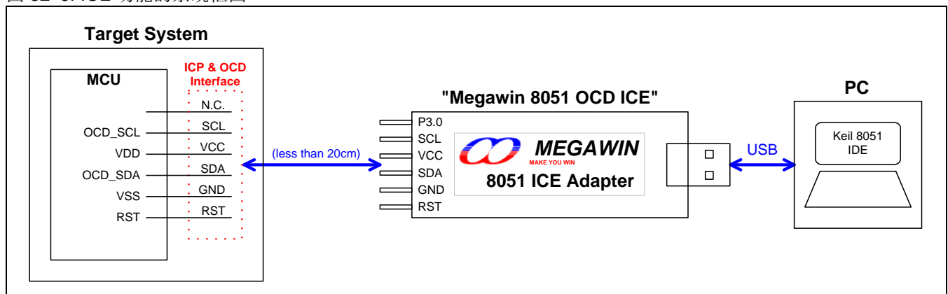
图 32-6. ICE 功能的系统框图
