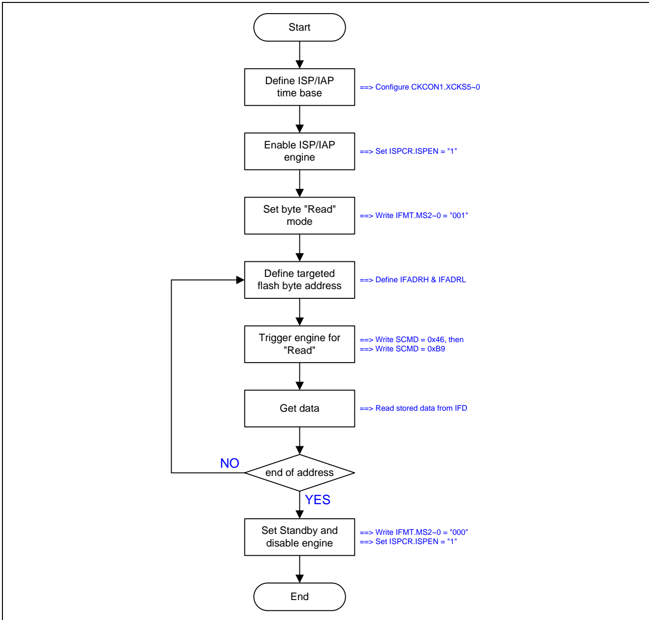
图 28-6. ISP/IAP 字节读流程
