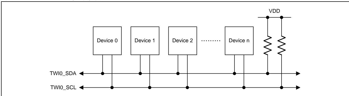
图 19-1. TWI/I2C 总线互联框图
