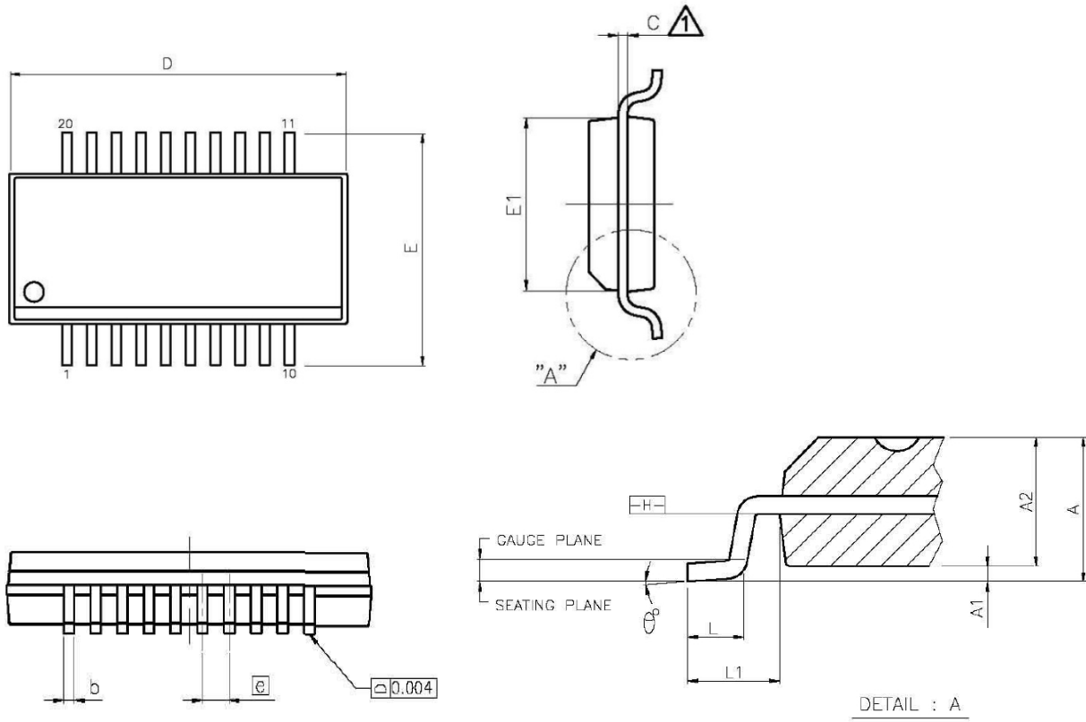
图 35-2. SSOP-20 SSOP20 (150 mil) Package dimension
