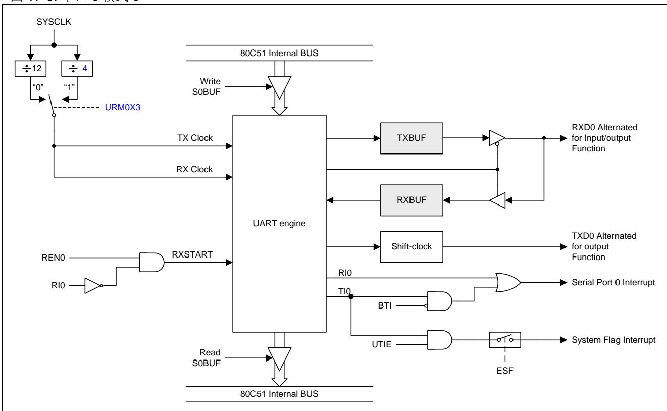
图 17-3. 串口 0 模式 0
