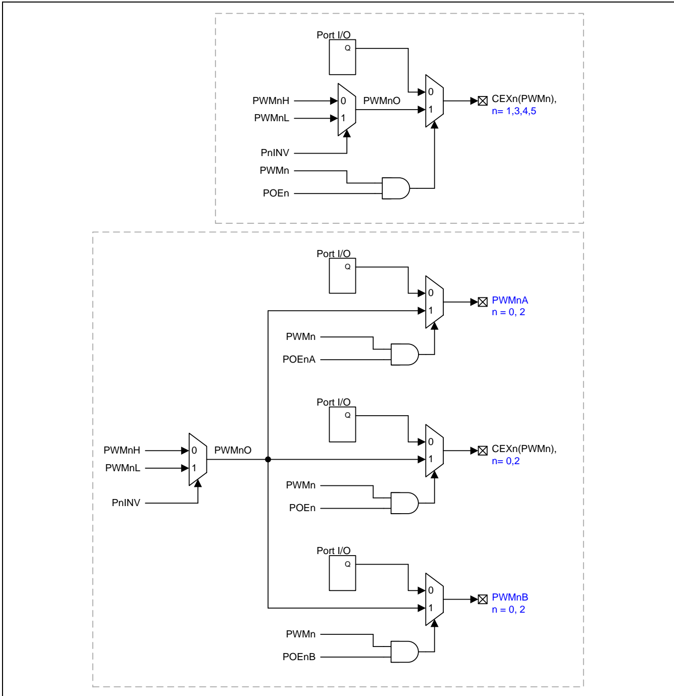
图 16-20. PCA0 模块输出控制
