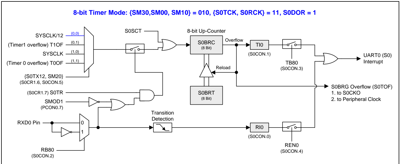
图 17-16. S0 的 8 位定时器模式
