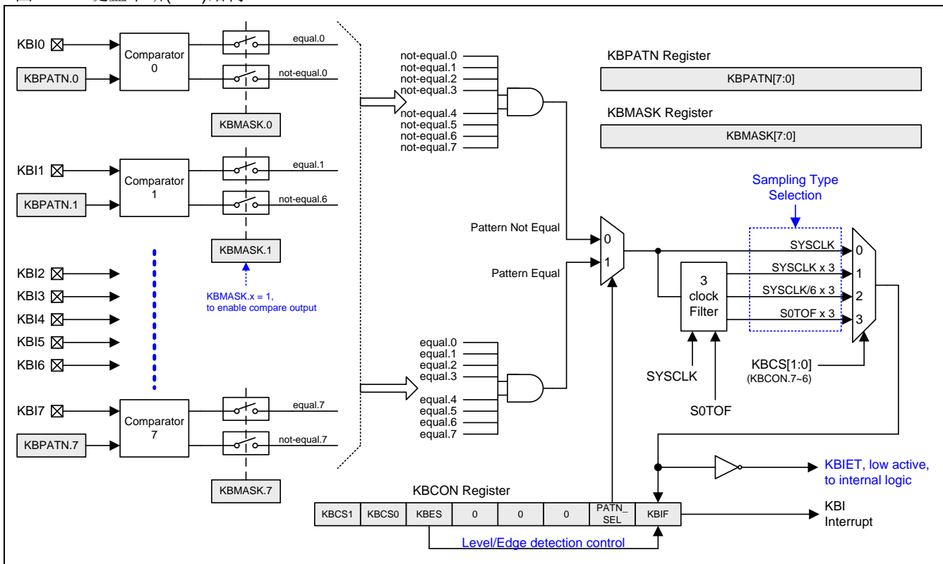
图 22-1. 键盘中断(KBI)结构
