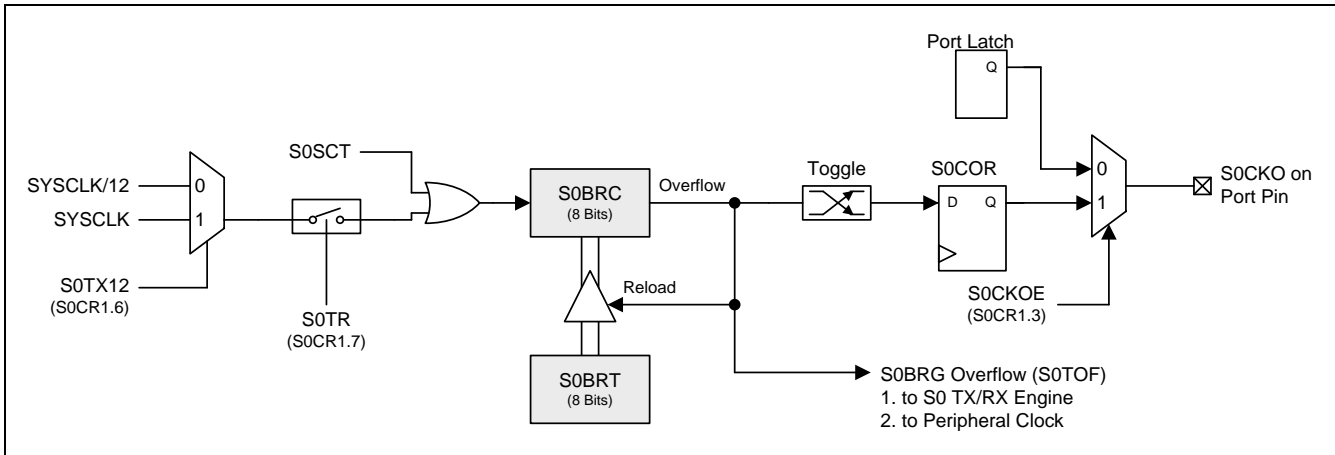
图 17-18. S0 16 位定时器模式
