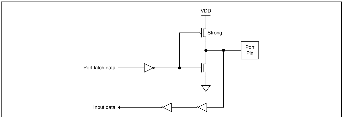
图 13-2. 端口 3 推挽输出结构
