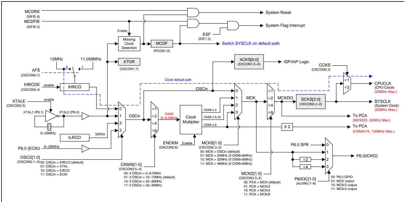
图 8-1. 系统时钟
