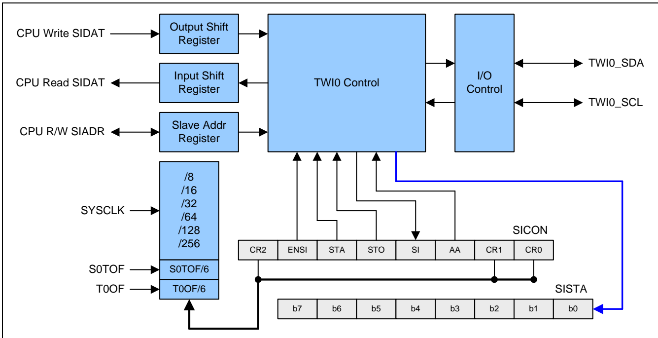
图 19-2. TWI/ I2C 方框图
