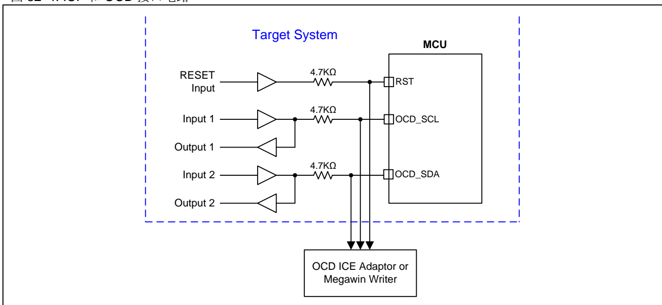
图 32-4. ICP 和 OCD 接口电路
