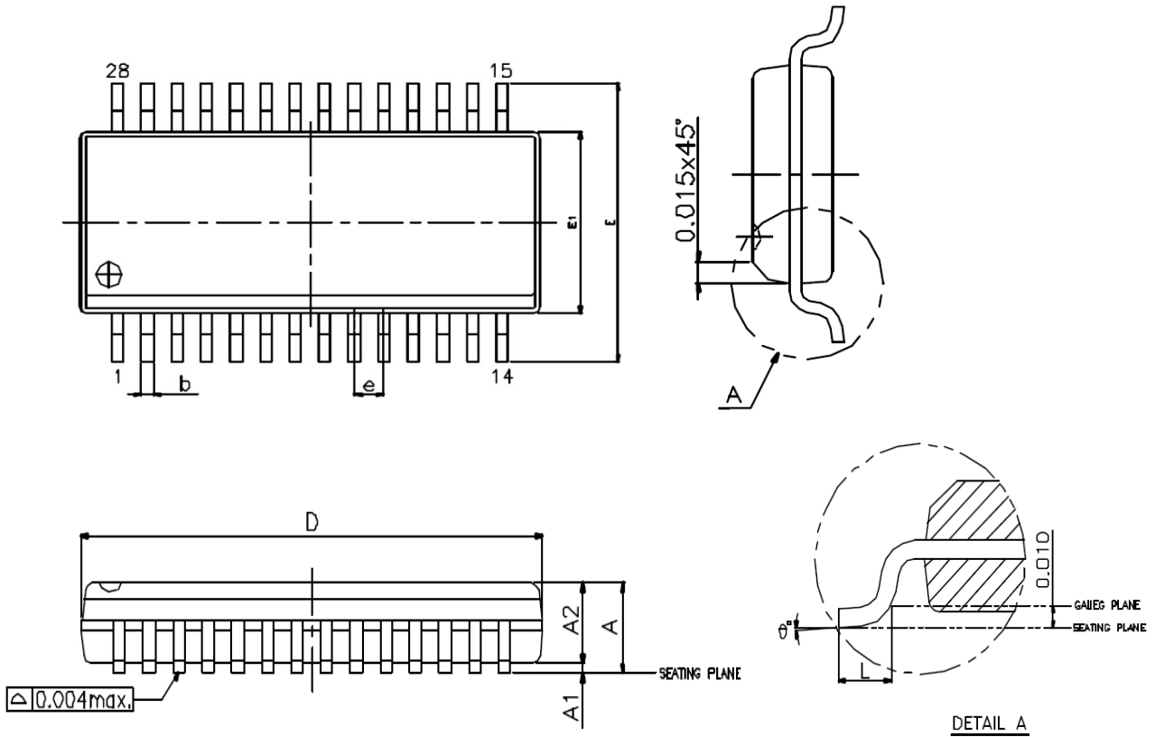
图 35-1. SSOP-28
