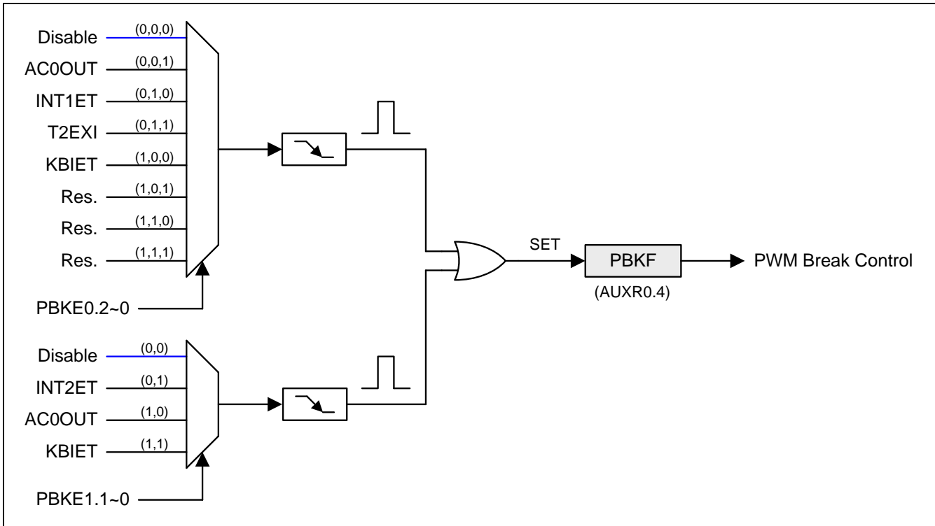
图 16-19. PCA PWM 中止控制源
