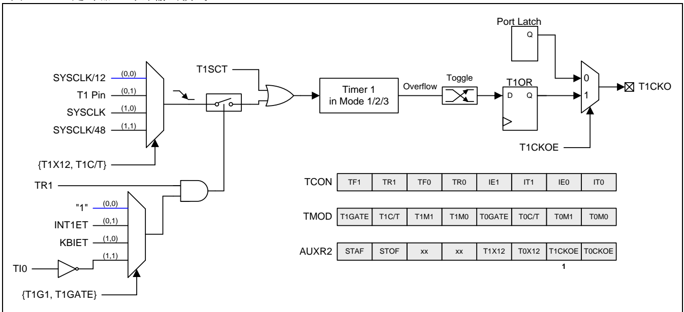
图 15-11. 定时器 1 时钟输出模式
