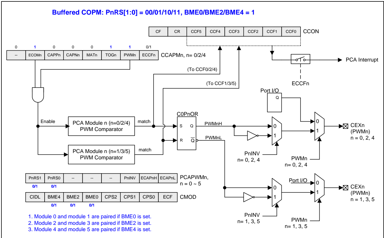
图 16-13. PCA0 缓冲 COPM 模式
