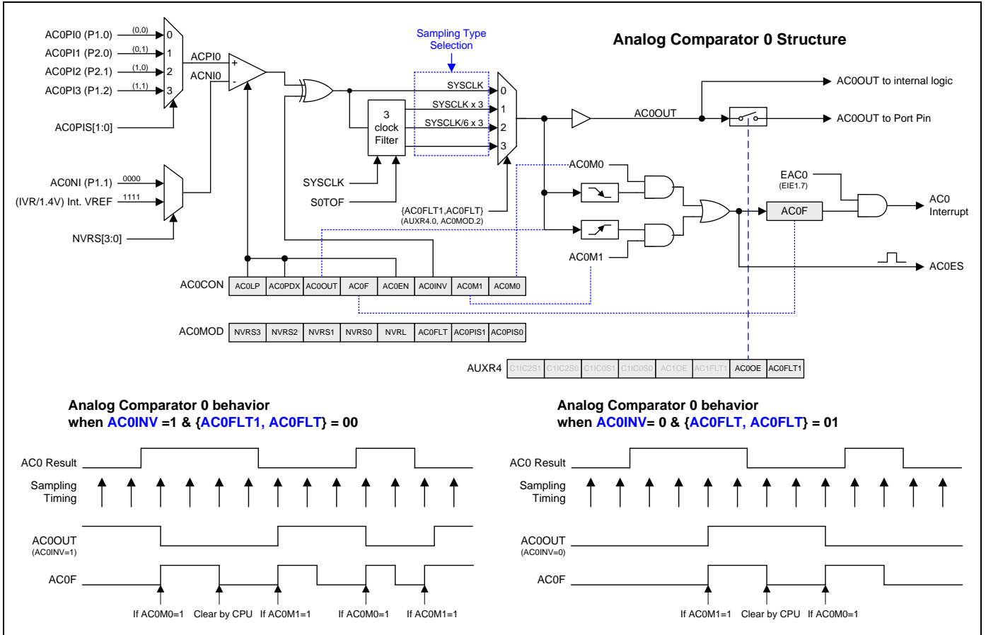
图 26-1. 模拟比较器 0 方框图
