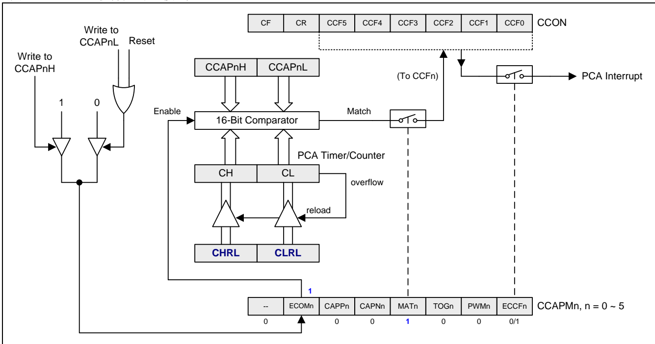
图 16-7. PCA0 软件定时器模式
