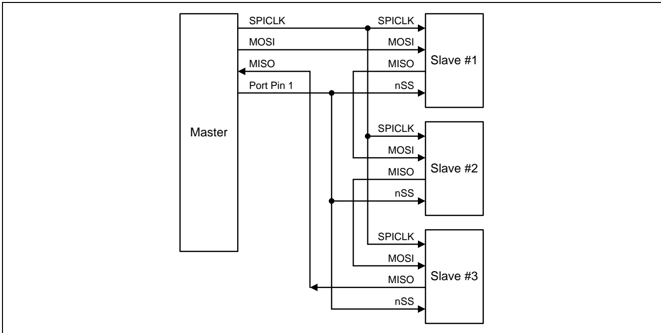
图 18-5. SPI 单主机多从机连接结构
