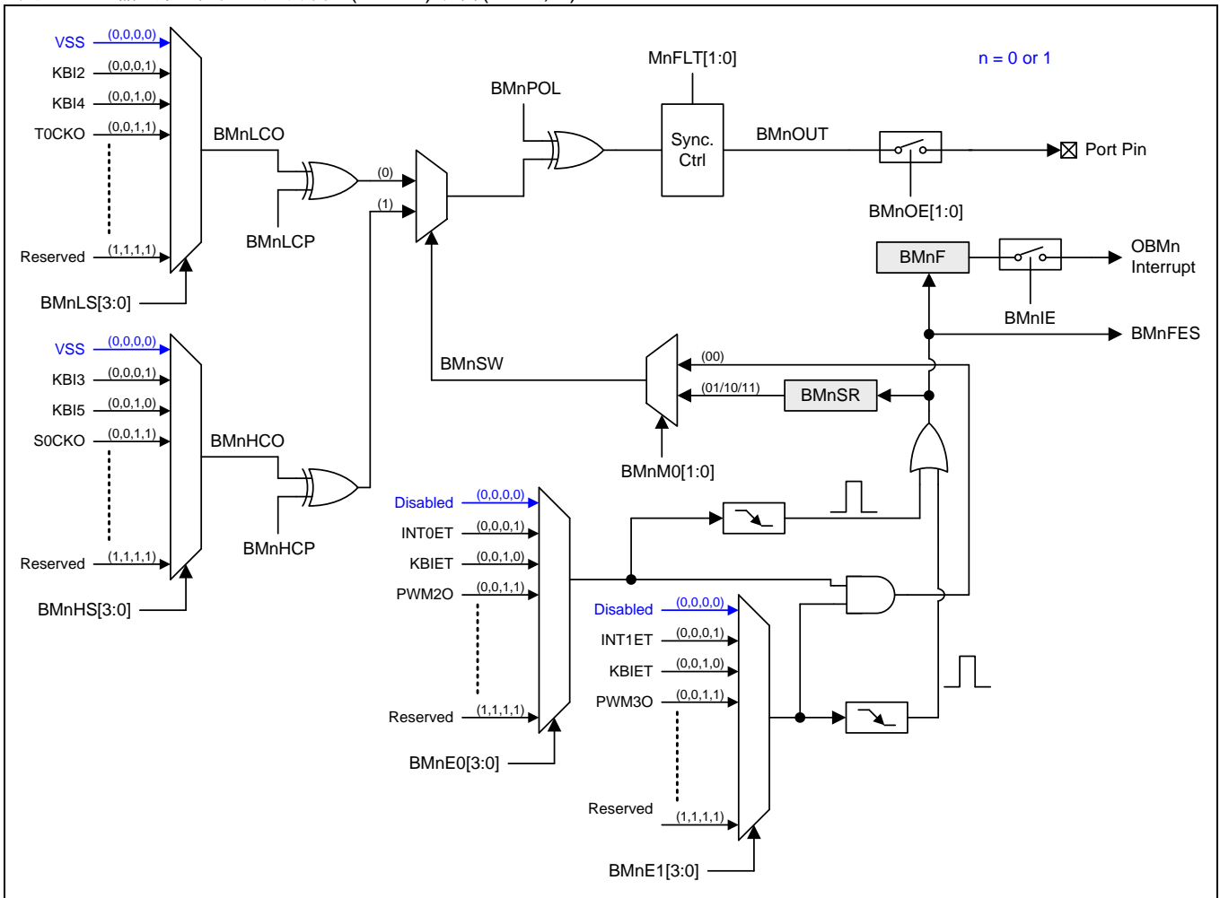
图 24-2. 输出信号中止和调制 n(OBMn)结构(n = 0, 1)
