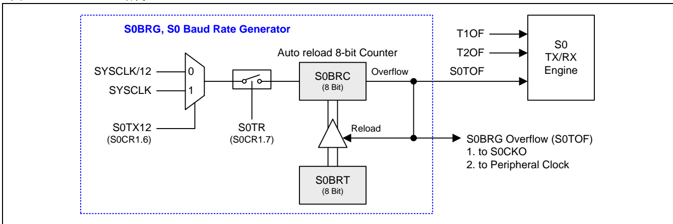
图 17-14. S0BRG 结构
