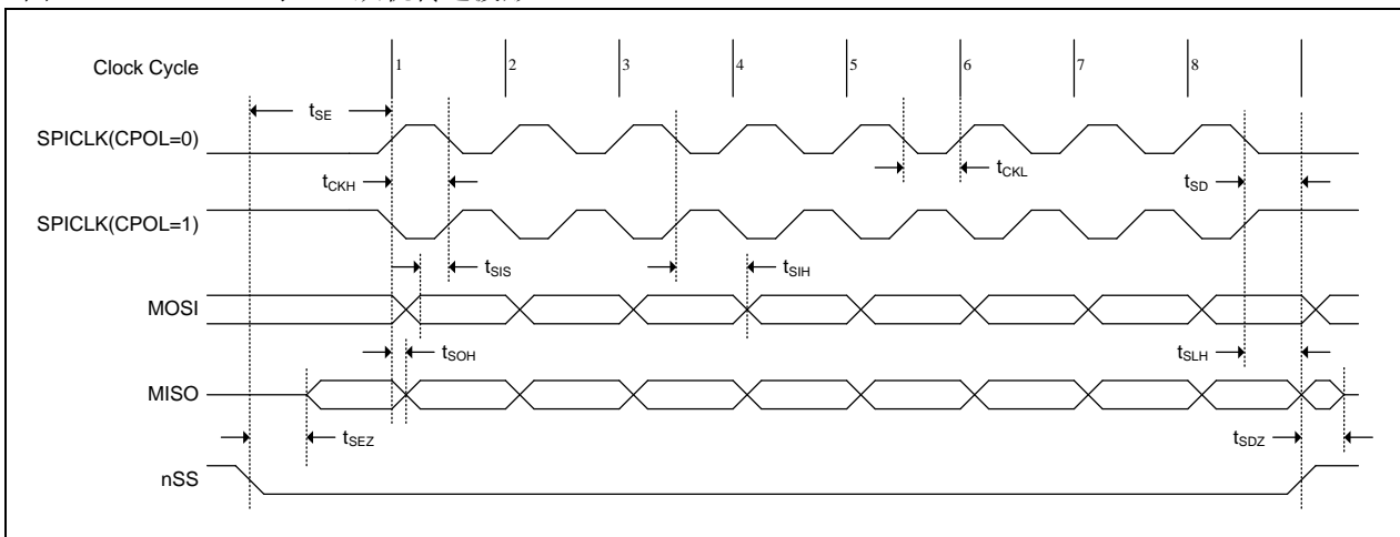
图 33-6. CPHA=1 时 SPI 从机传送波形
