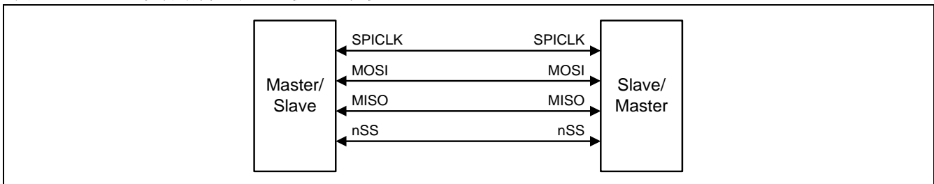
图 18-3. SPI 双设备结构，既是主机也是从机
