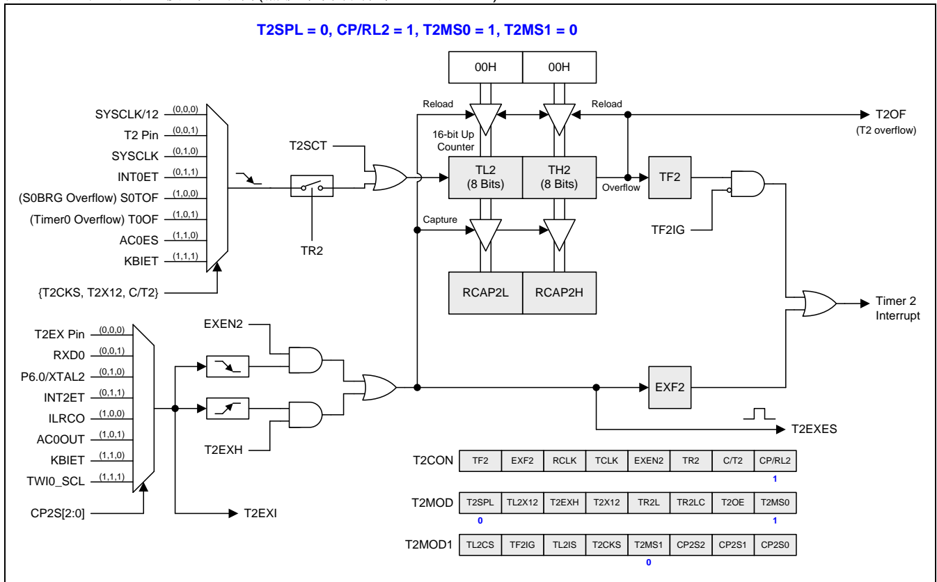
图 15-15. 定时器 2 模式 3 结构(捕获带自动清零 TL2 和 TH2)
