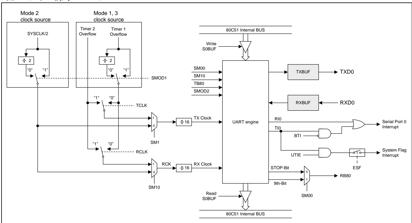
图 17-6. 串口模式 1、2、3
