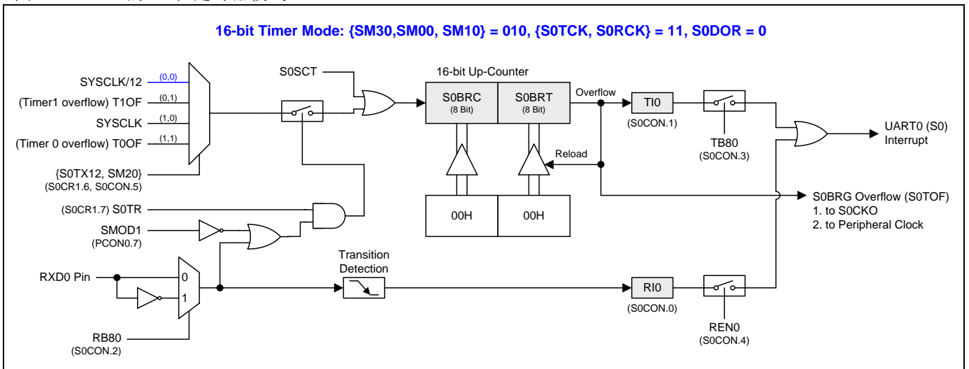
图 17-17. S0 的 16 位定时器模式
