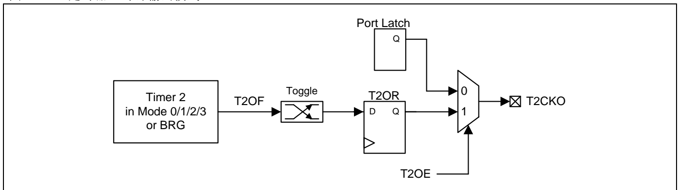
图 15-24. 定时器 2 时钟输出模式
