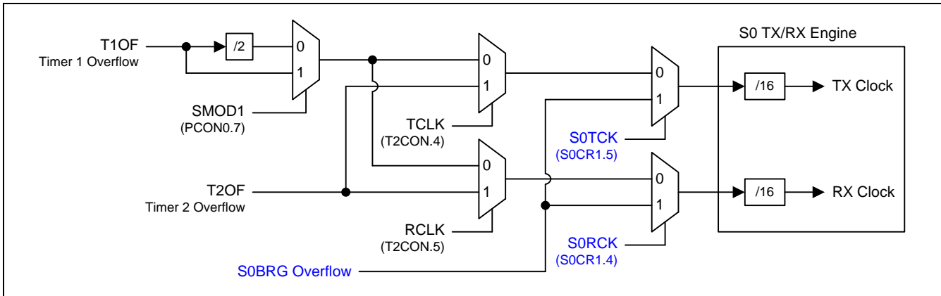
图 17-15. S0 波特率选择
