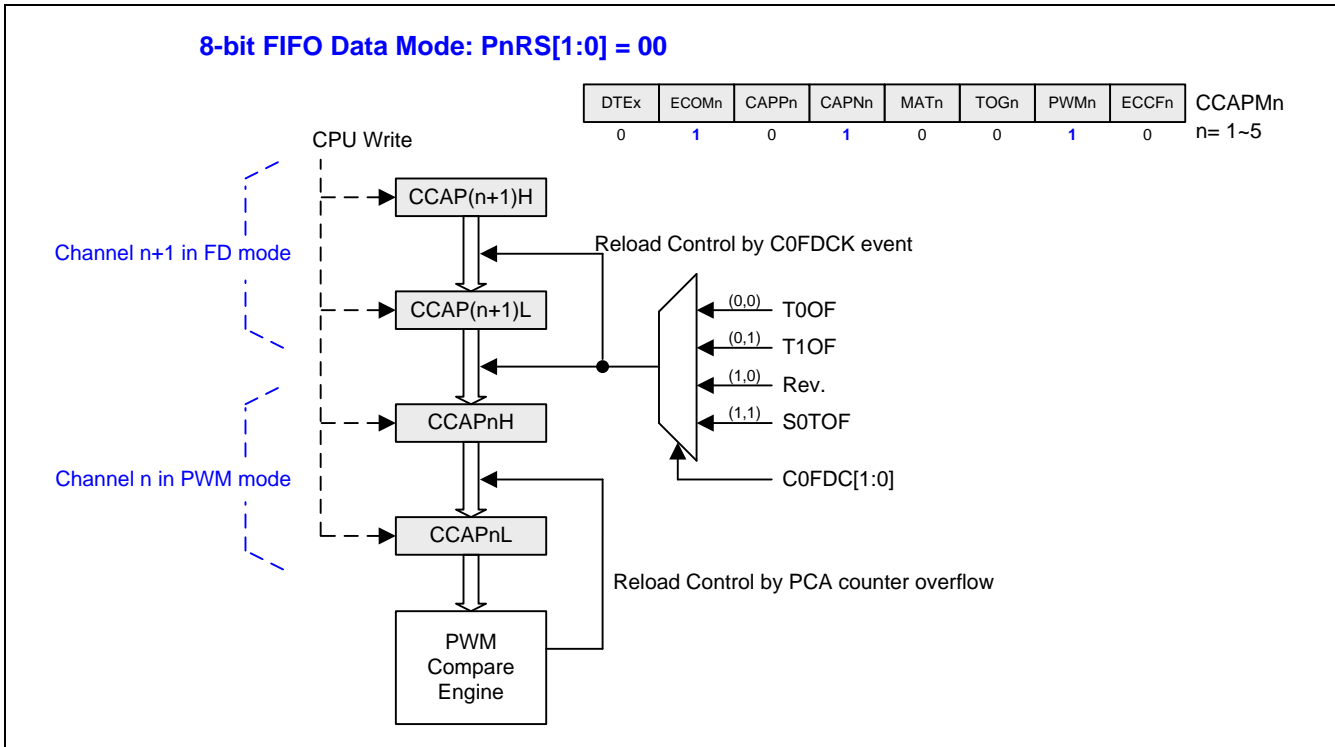
图 16-14. PCA0 信道作为 FIFO 数据模式
