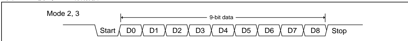
图 17-2. 模式 2, 3 数据帧
