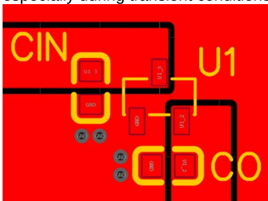
SOT233 PCB
